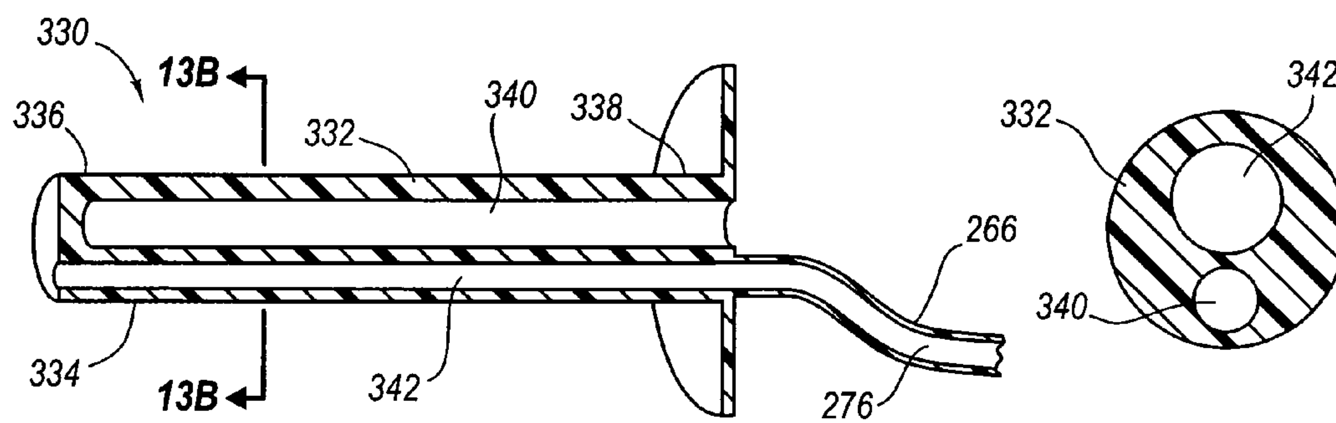
FIG. 13A
