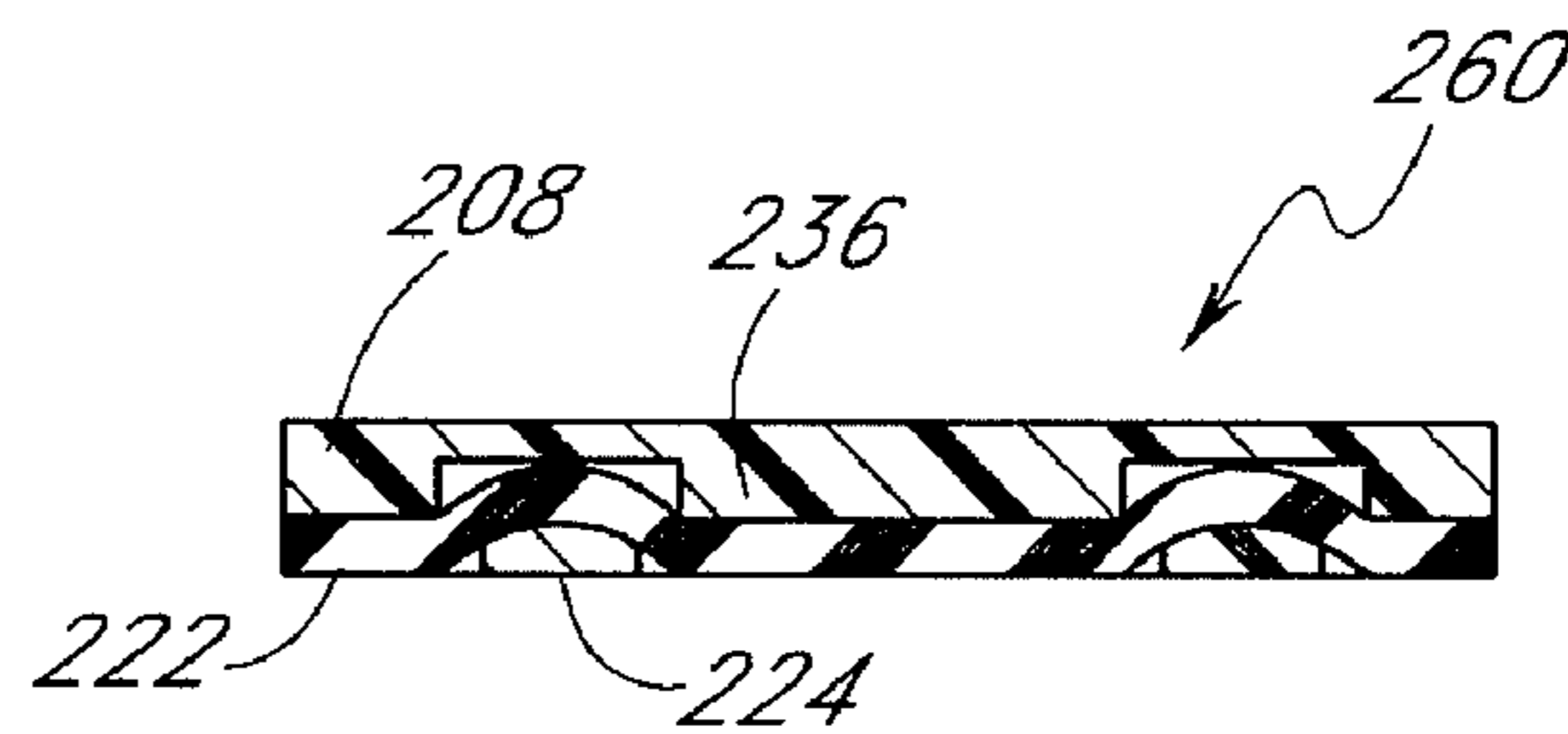
FIG. 21A
