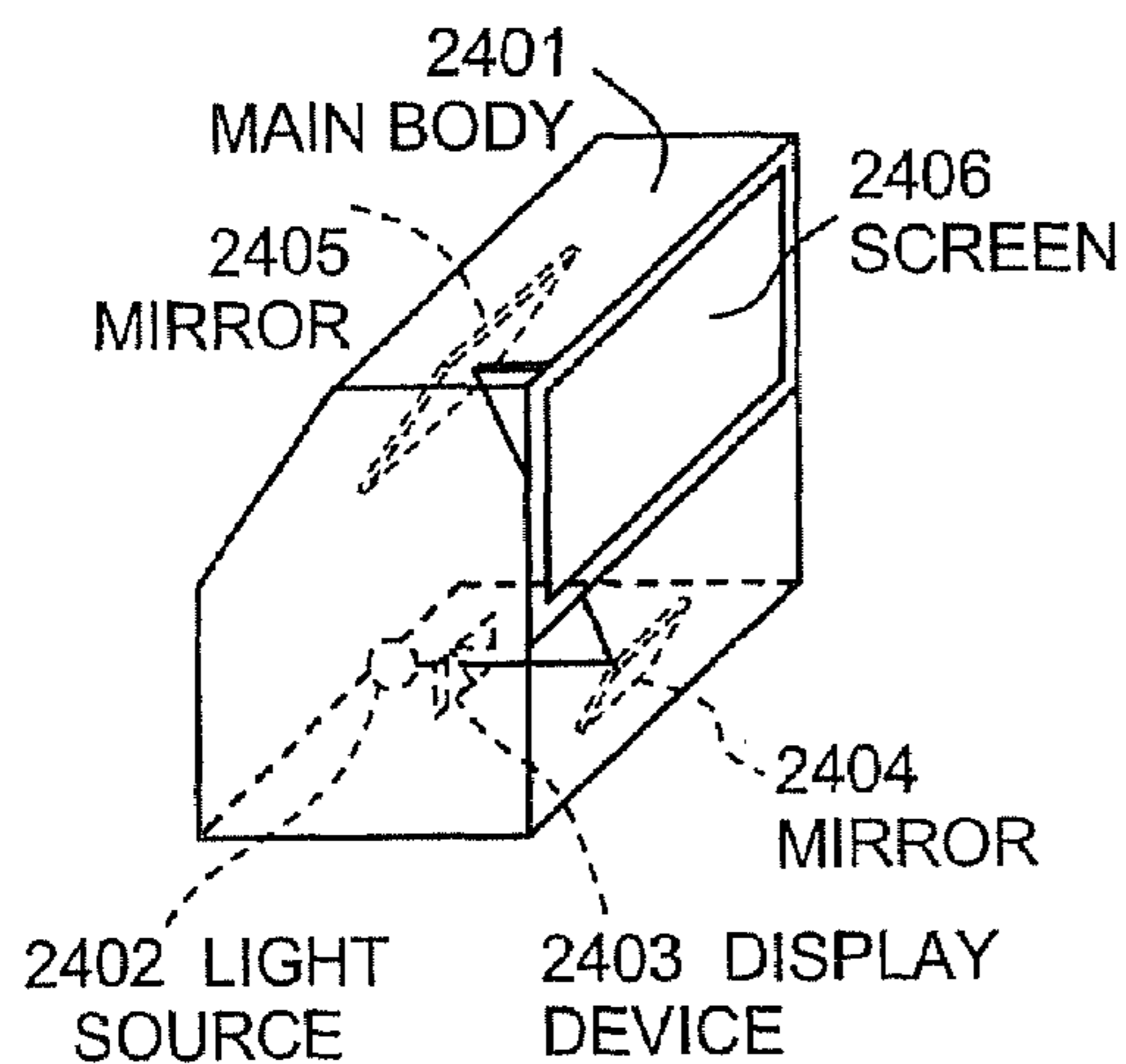
FIG. 15E
