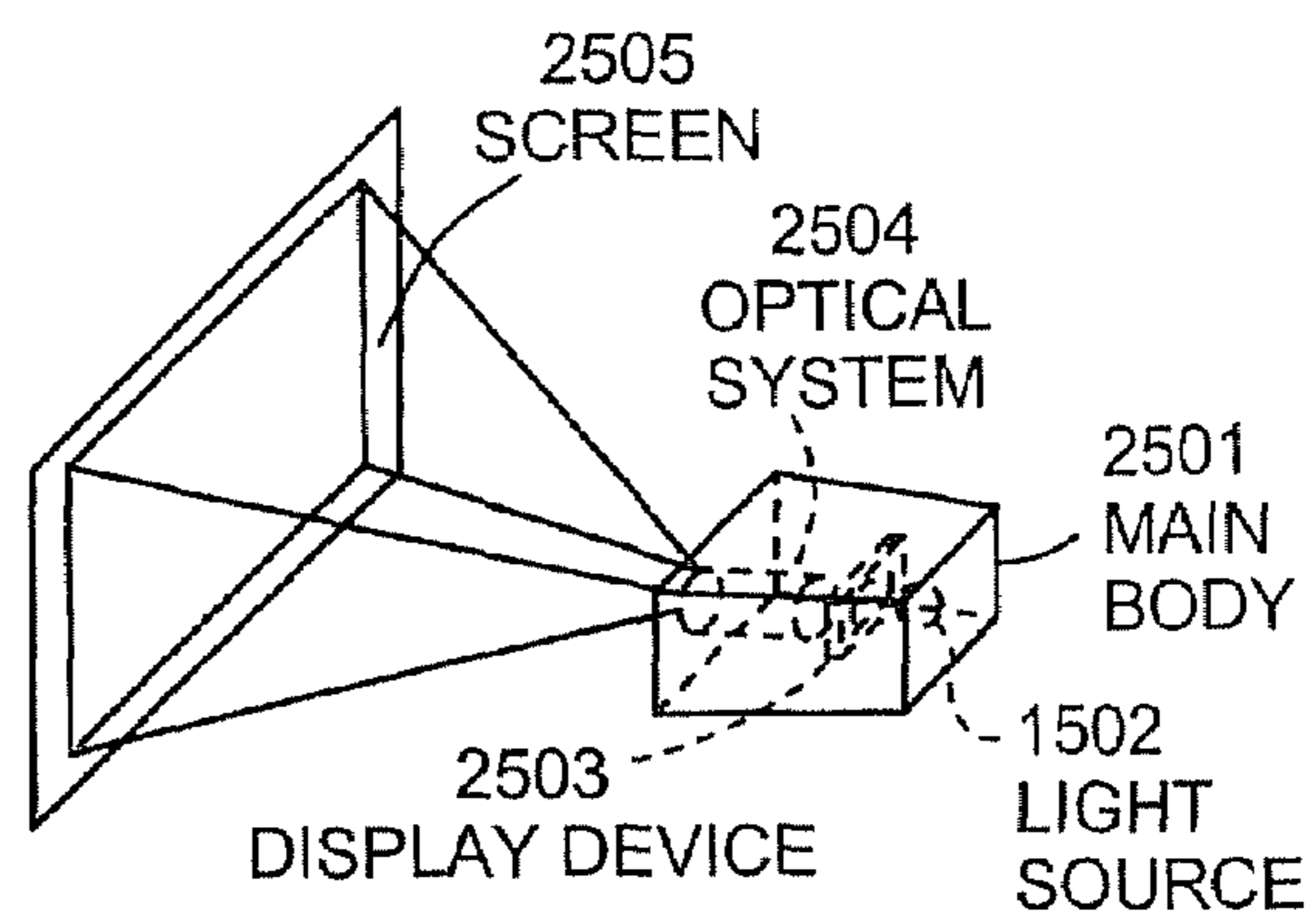
FIG. 15F
