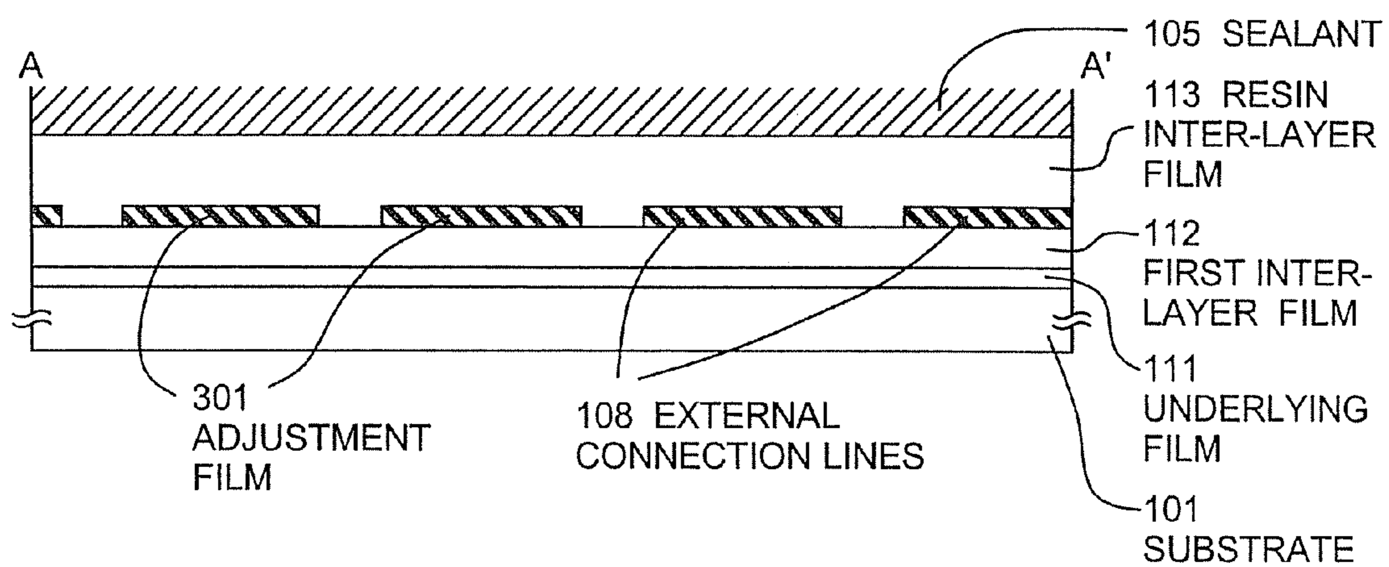
FIG. 3B
