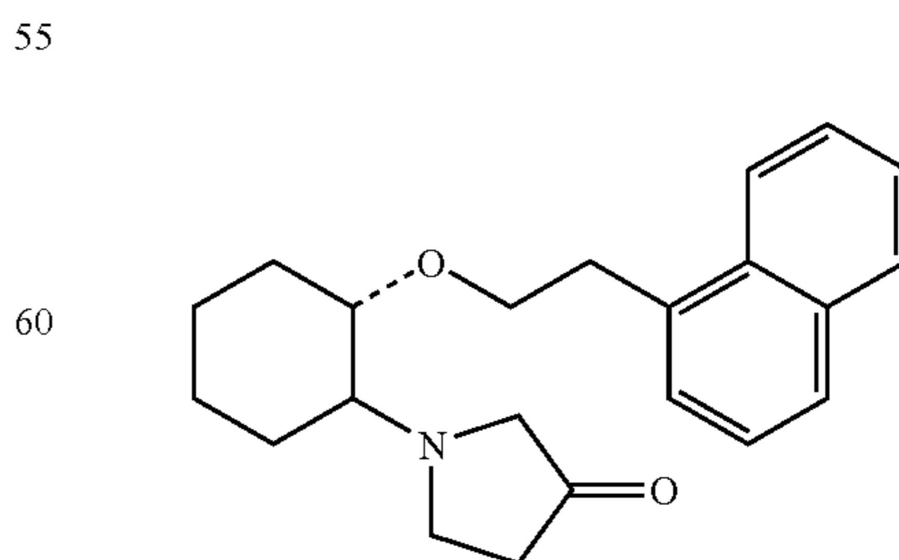
(1R,2R)/(1S,2S)-2-(3-ketopyrrolidinyl)-1-(1-naphthenethoxy)cyclohexane
