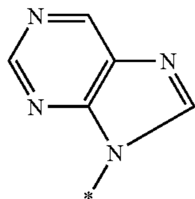
pyrimidinoimidazole
