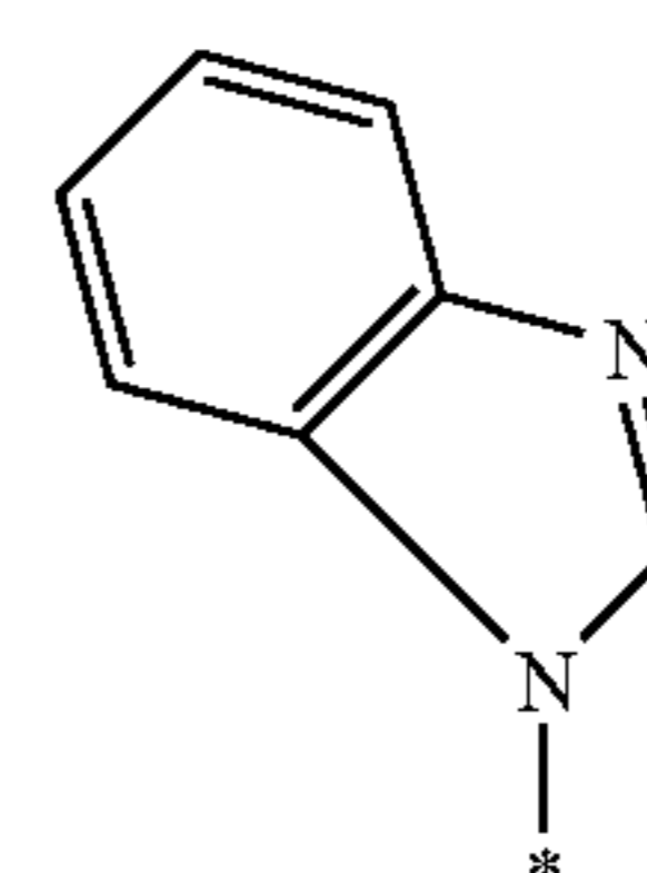
benzimidazole
