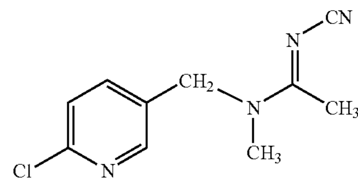
(acetamiprid)
