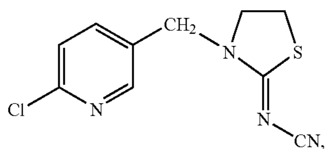
(thiacloprid)
