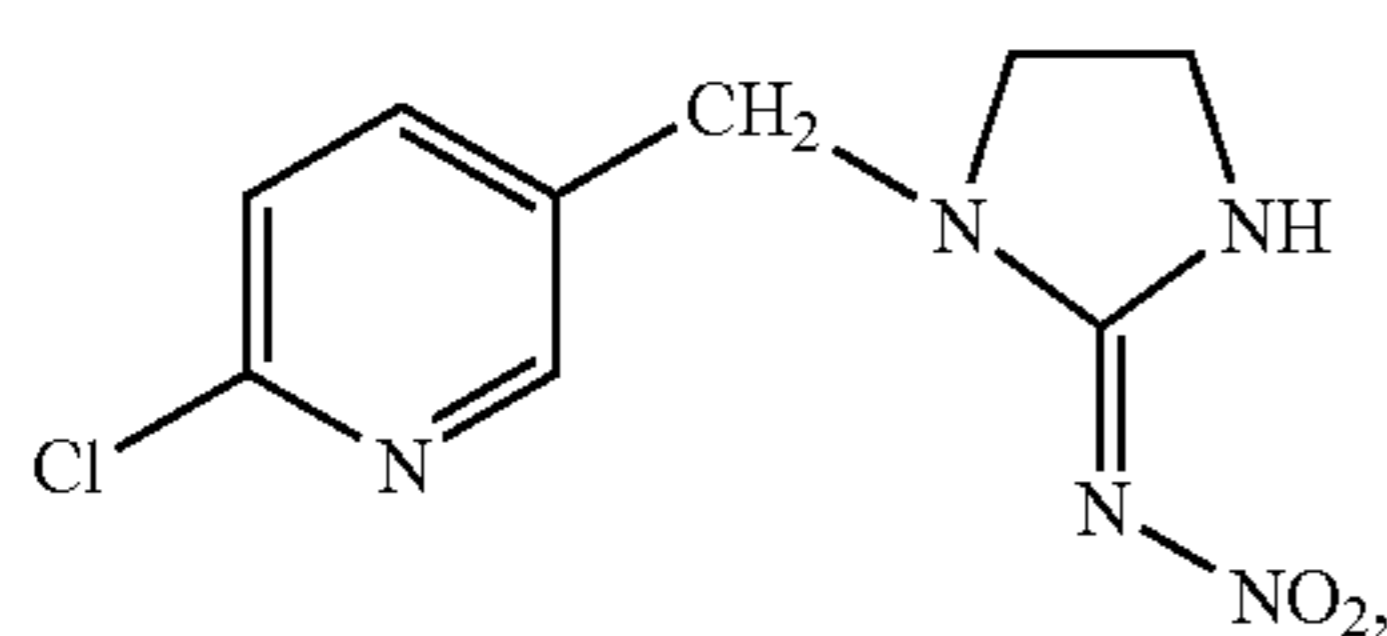
(imidacloprid)
