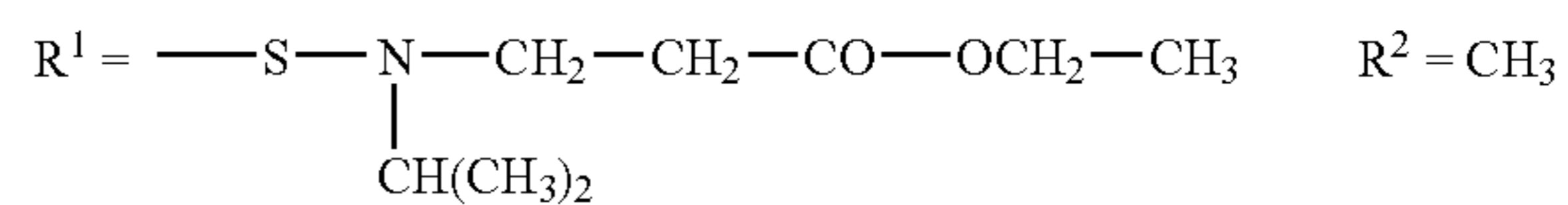
(benfuracarb)
