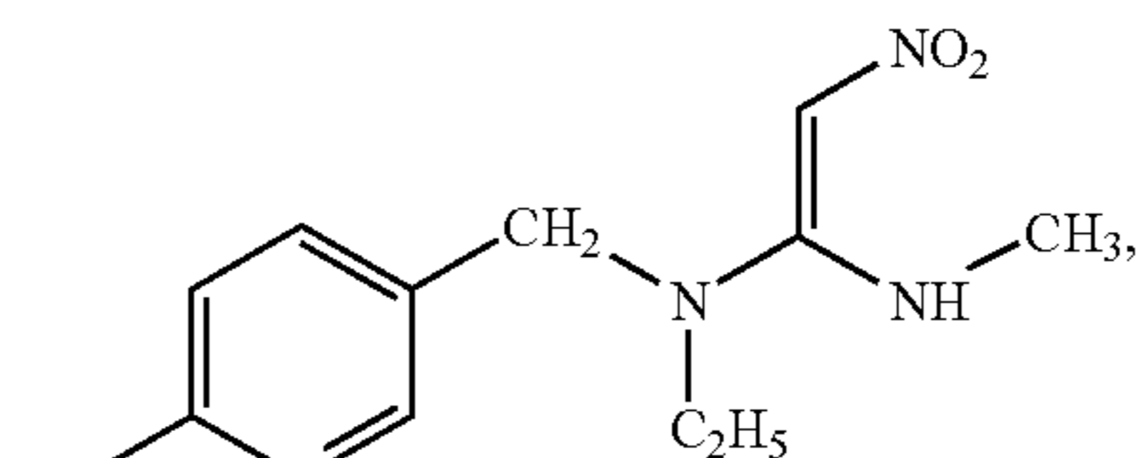
(nitenpyram)
