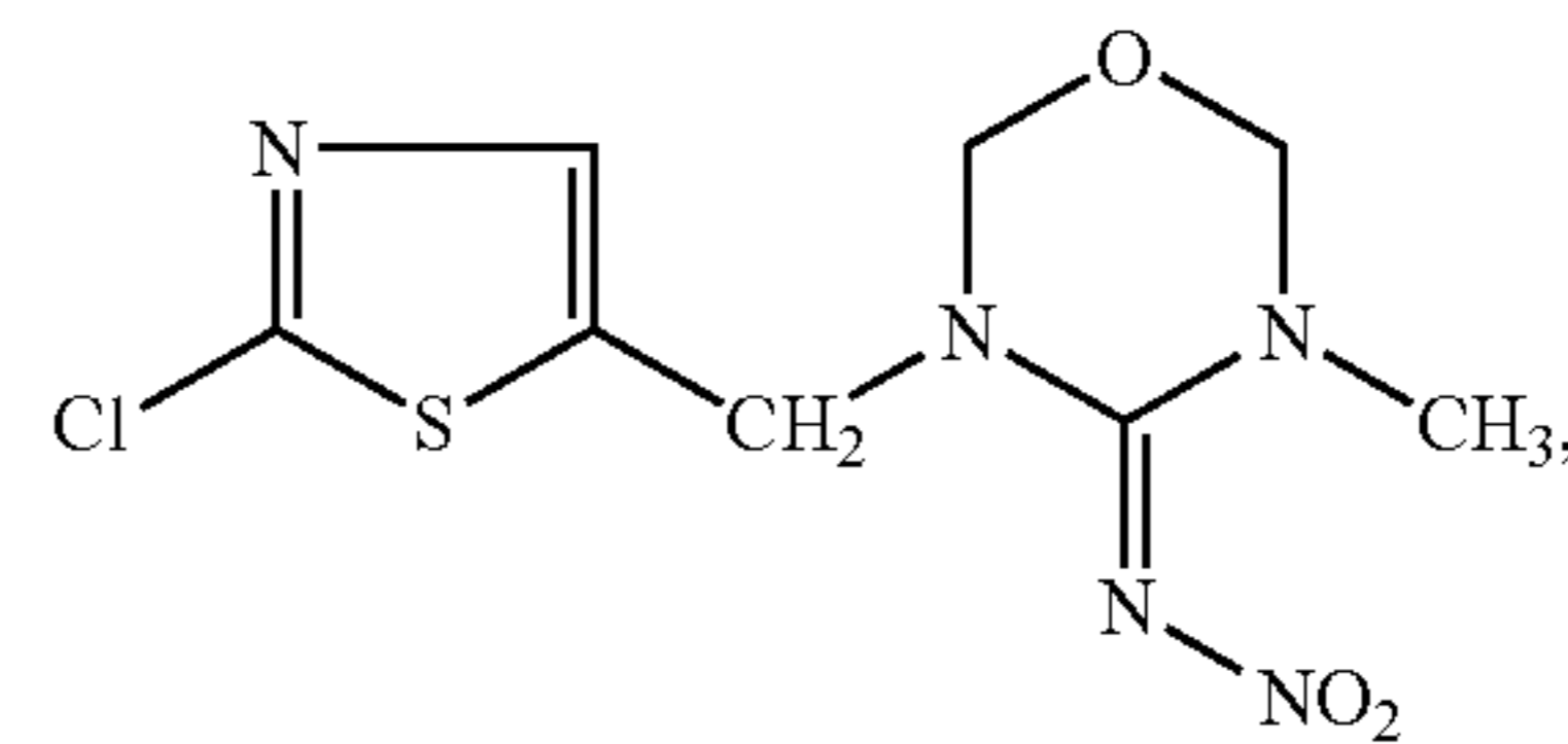
(thiamethoxam)
