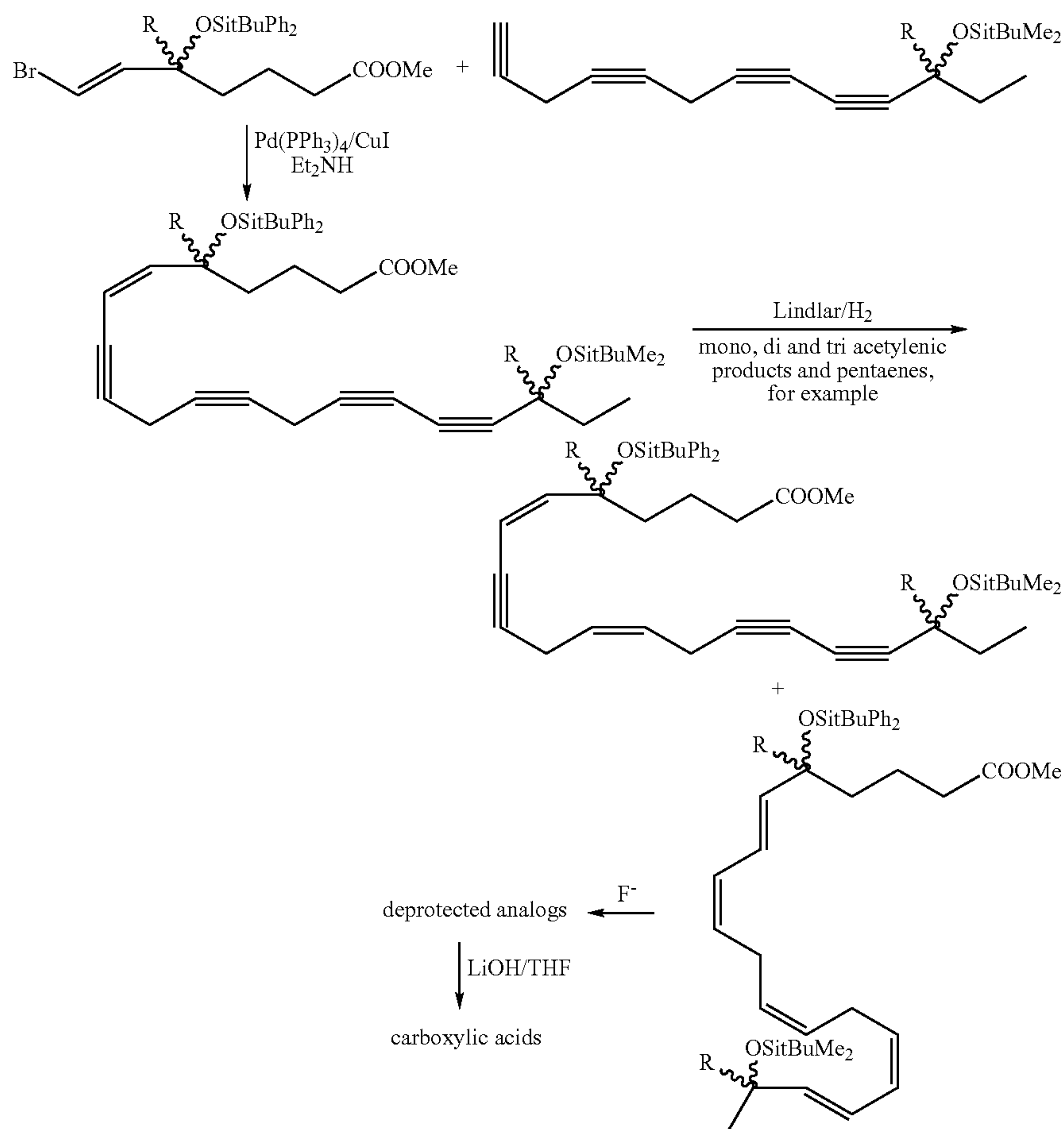
Scheme VI
