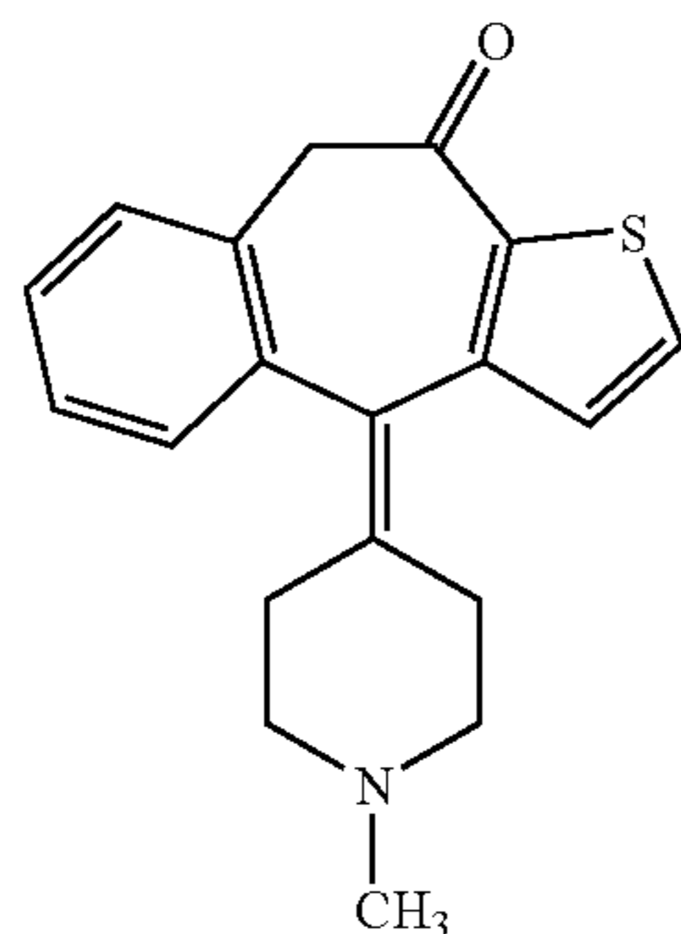
KETOTIFEN
