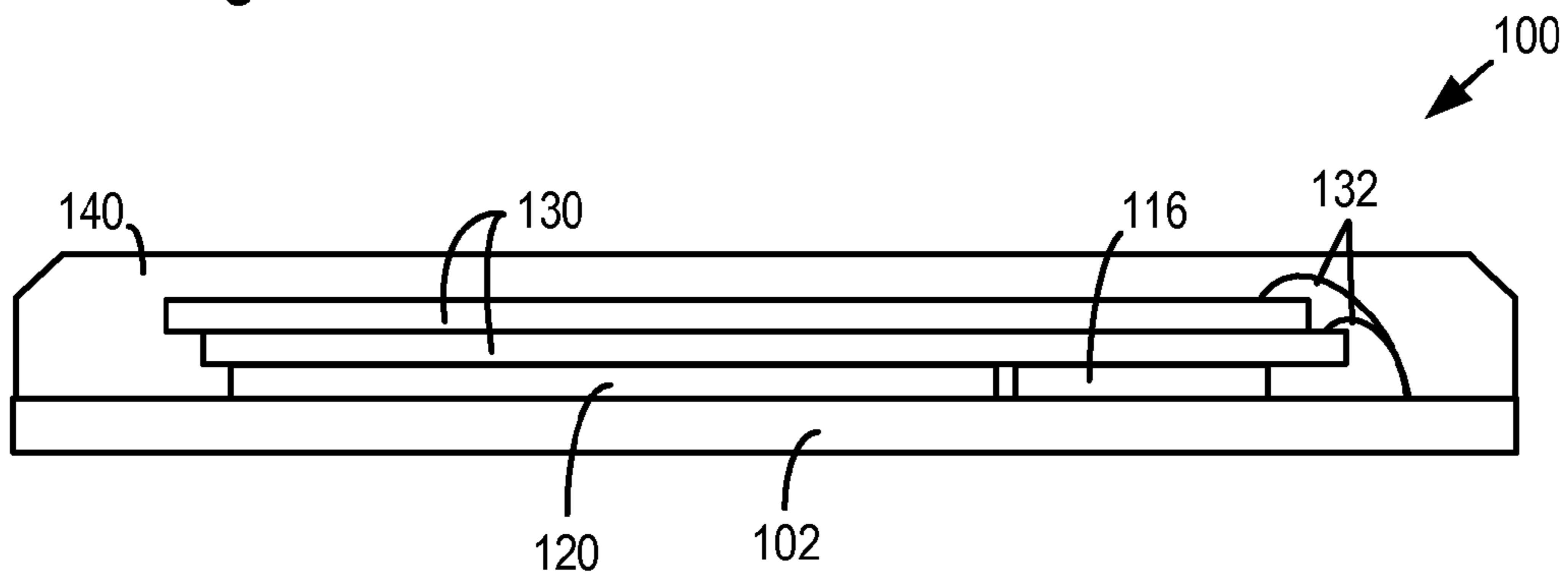
Fig. 14
