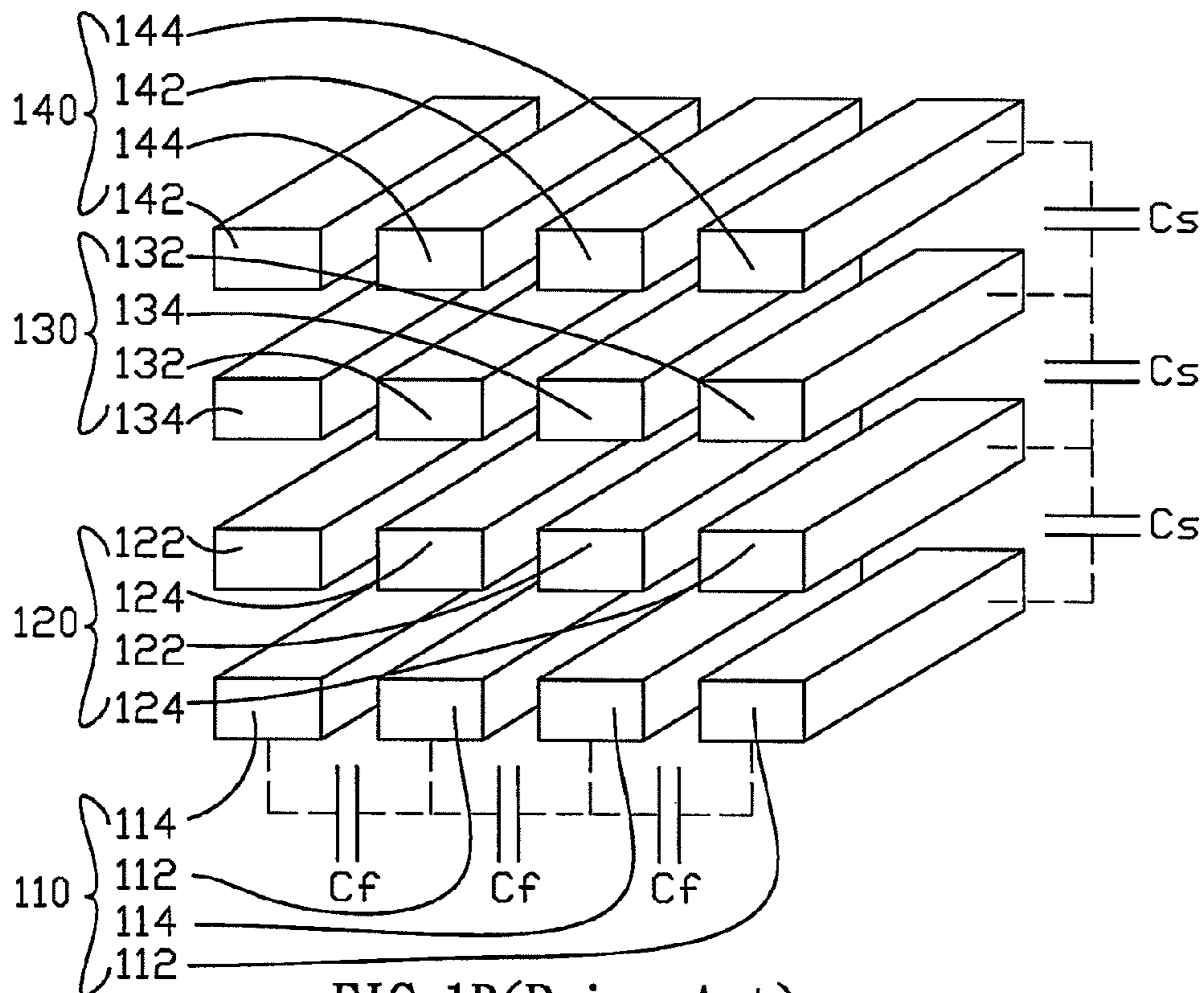
FIG. 1B(Prior Art)
