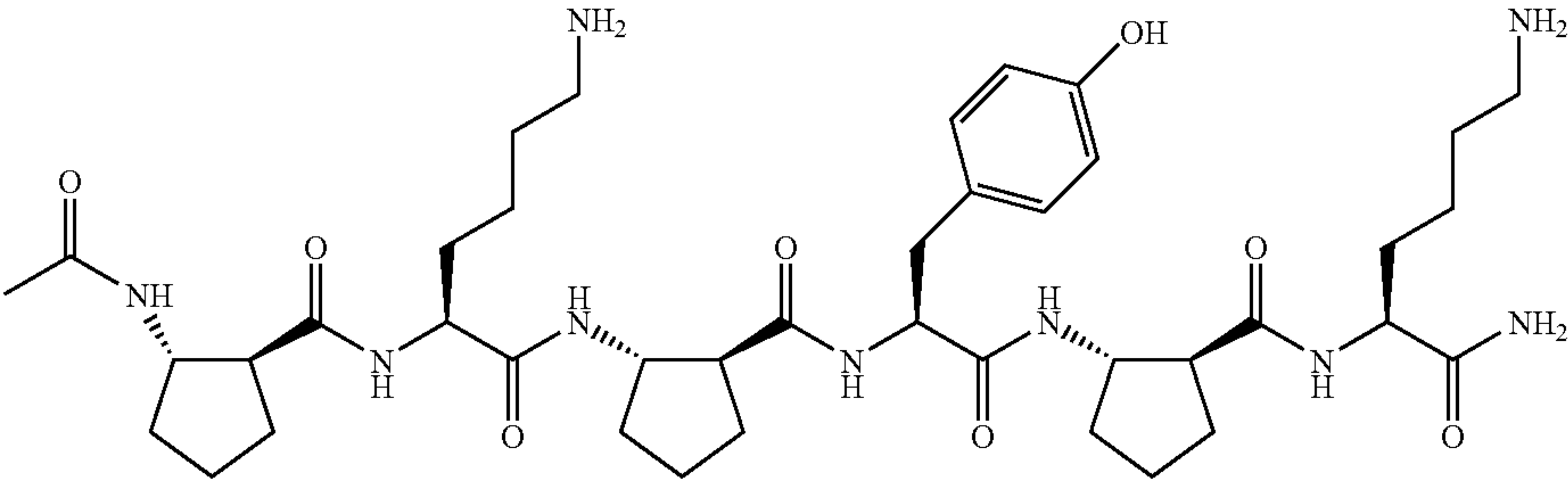
(S,S)-ACPC L-amino acids
