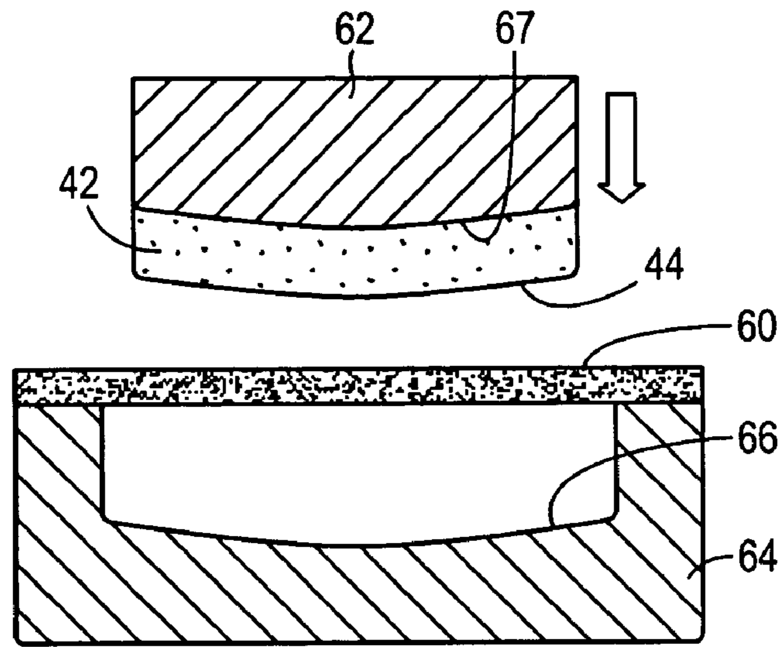
FIG. 5D
