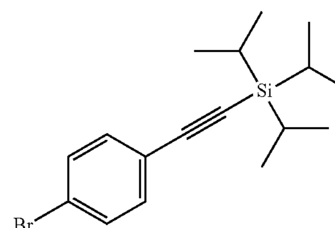
1-bromo-4-triisopropylsilylethynyl-benzene
