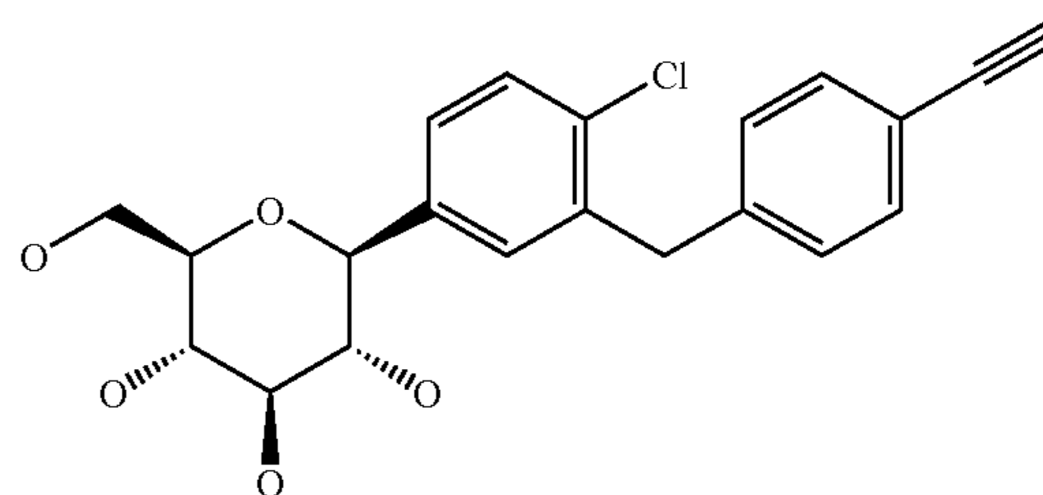
1-chloro-4-(β-D-glucopyranos-1-yl)-2-(4-ethynylbenzyl)-benzene
