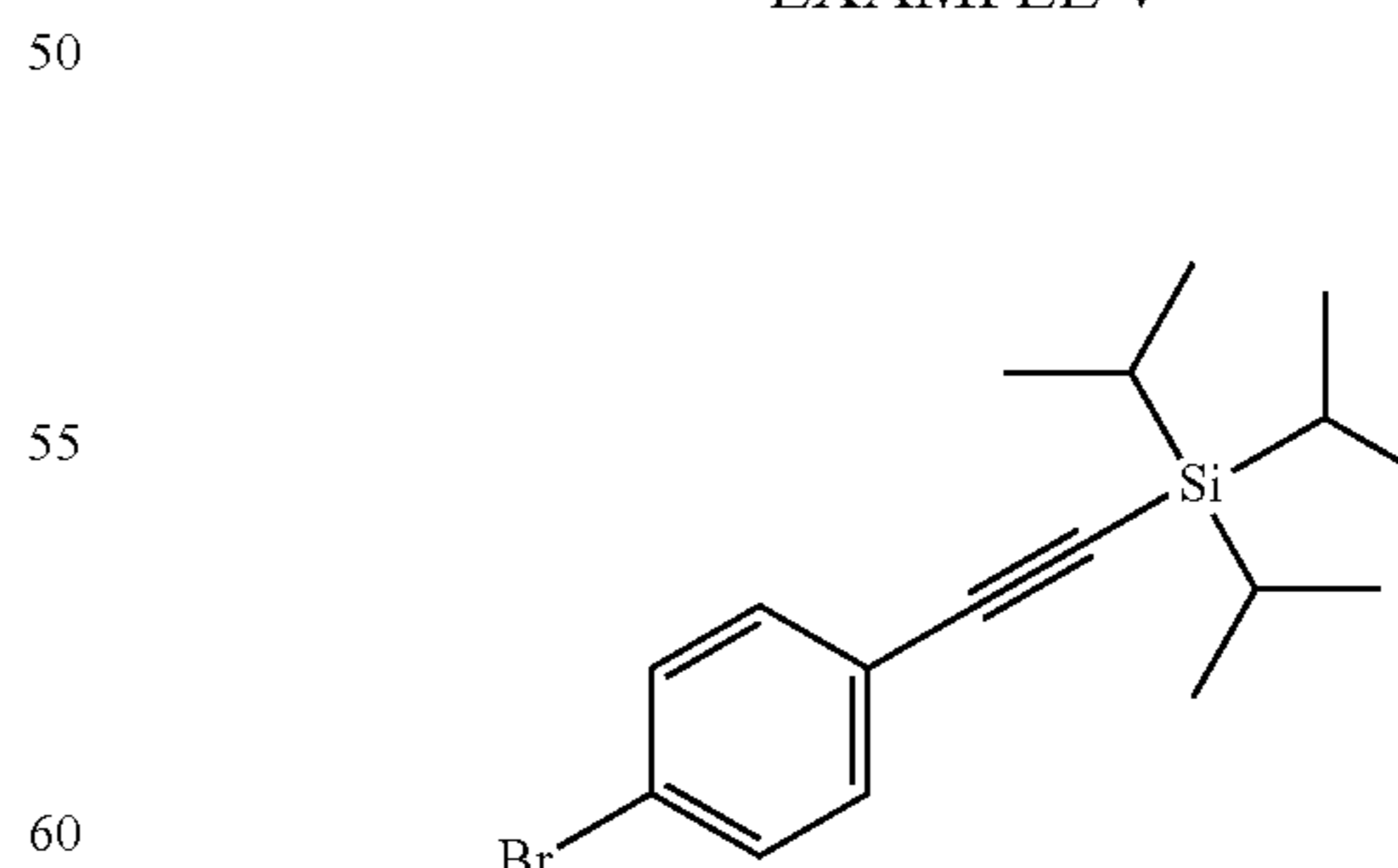
1-bromo-4-triisopropylsilylethynyl-benzene
