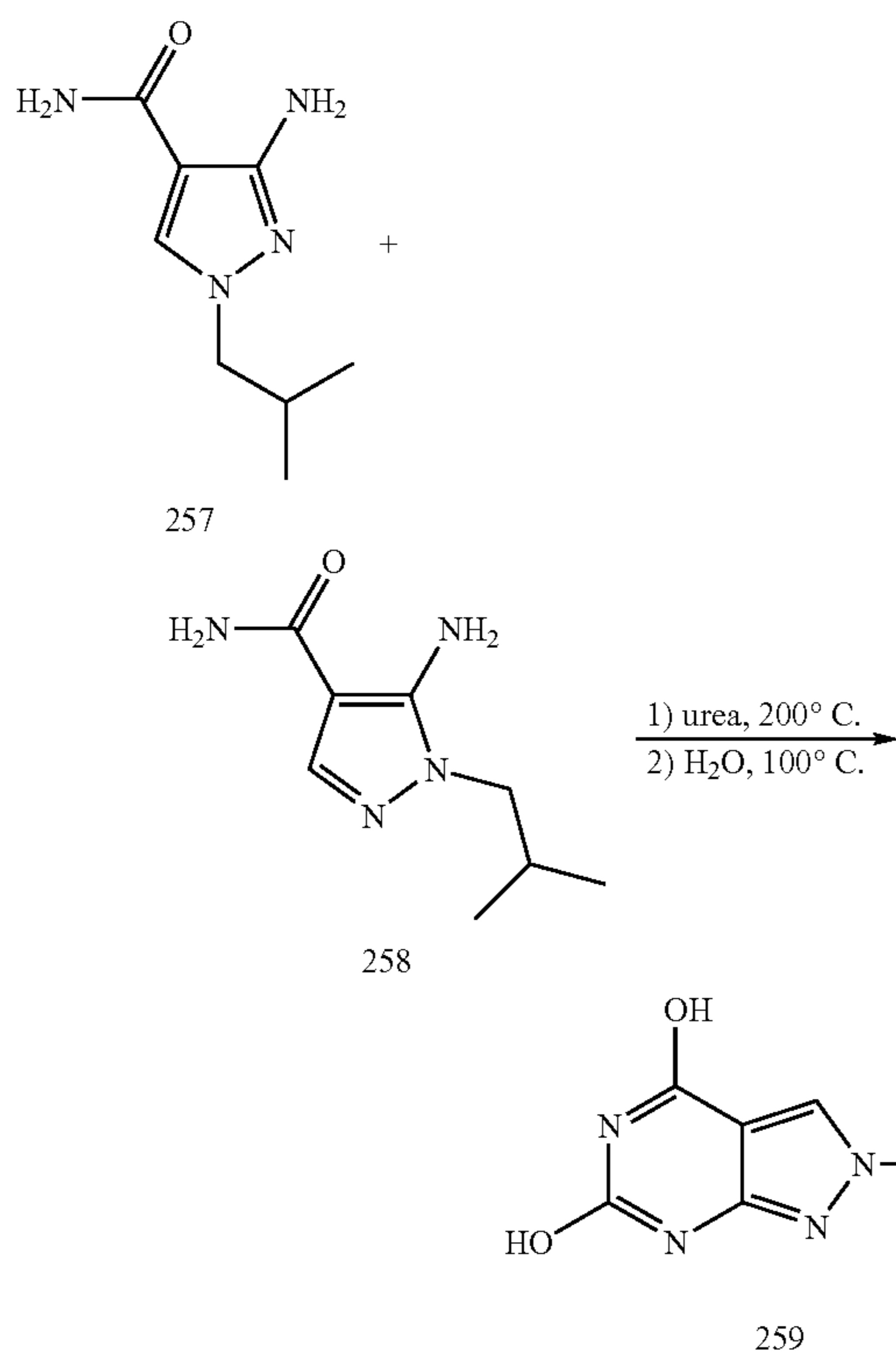
2-Isobutyl-2H-pyrazolo[3,4-d]pyrimidine-4,6-diol
