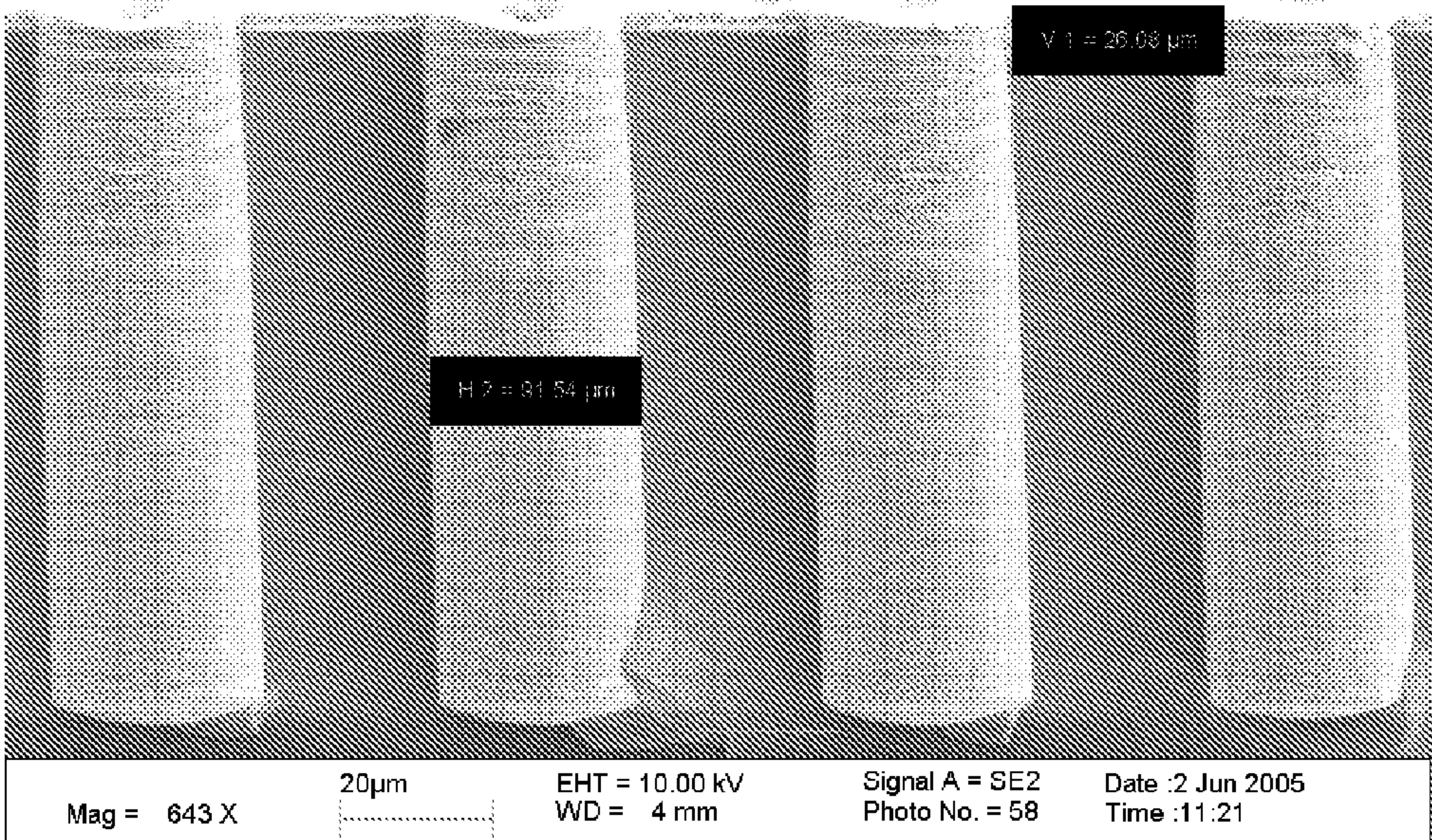
20 um diameter 100um deep filled Via
