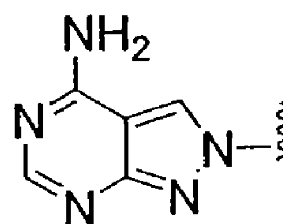
N8-(7-deaza-8-aza-A)
