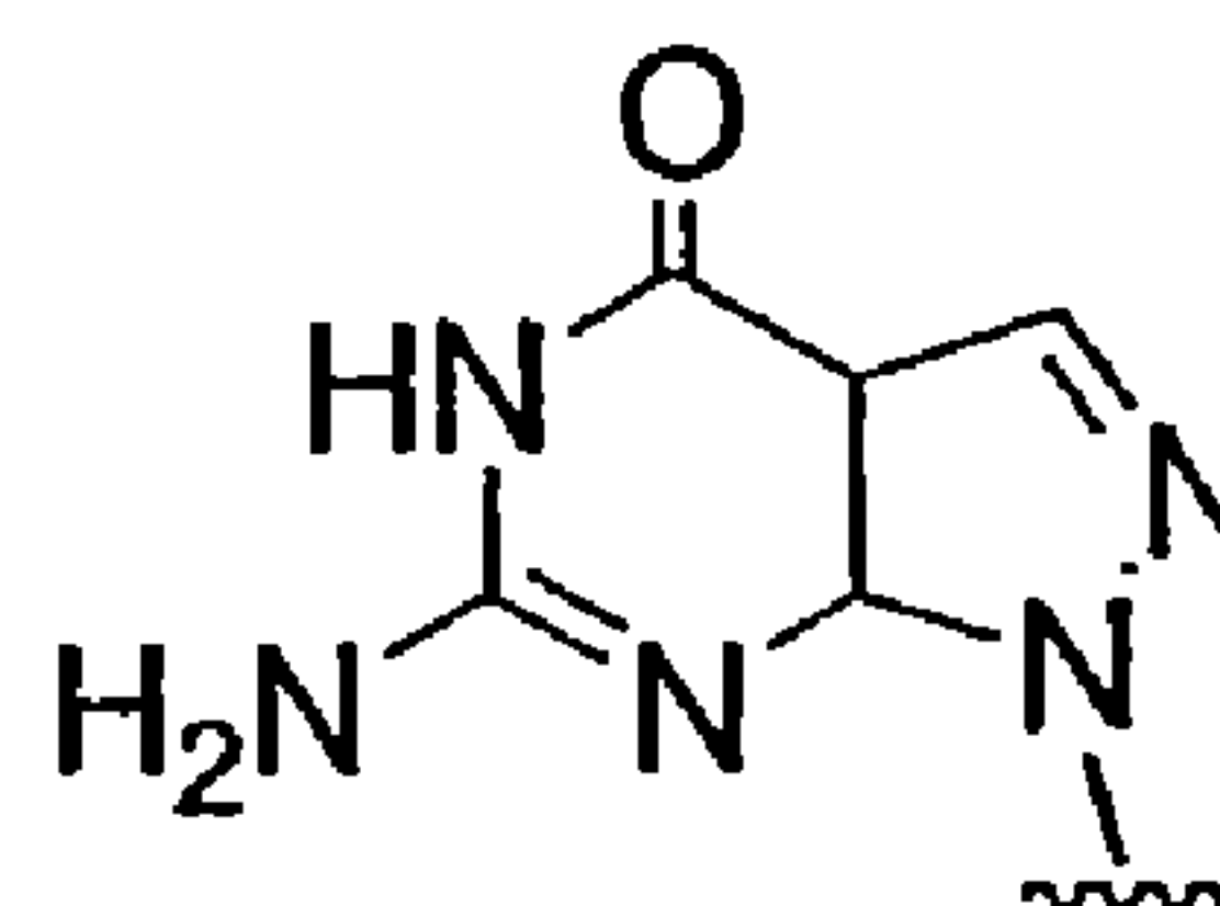
N9-(7-deaza-8-aza-G)
