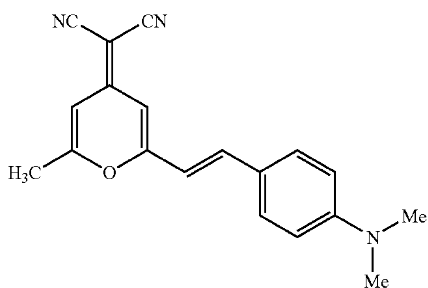
DCM1
