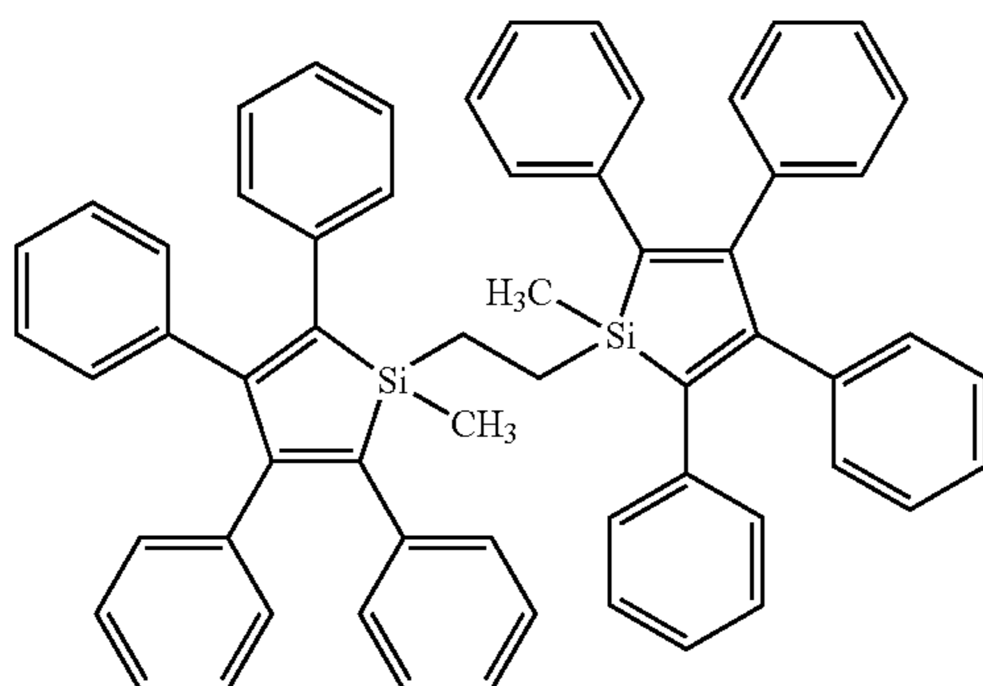
2PSP
