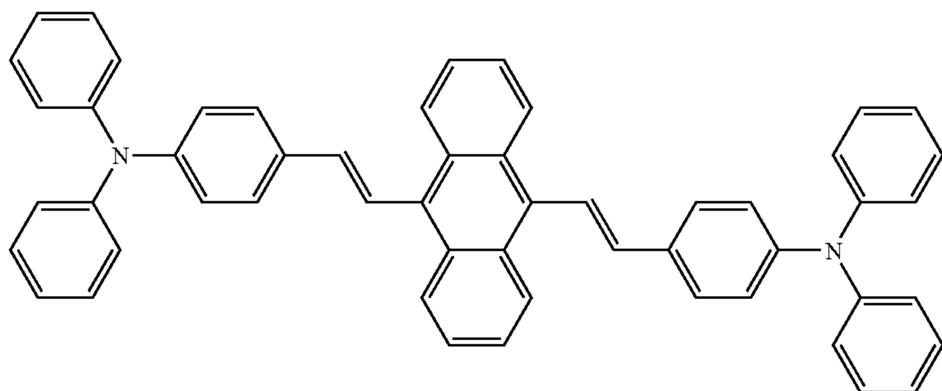
DSA
