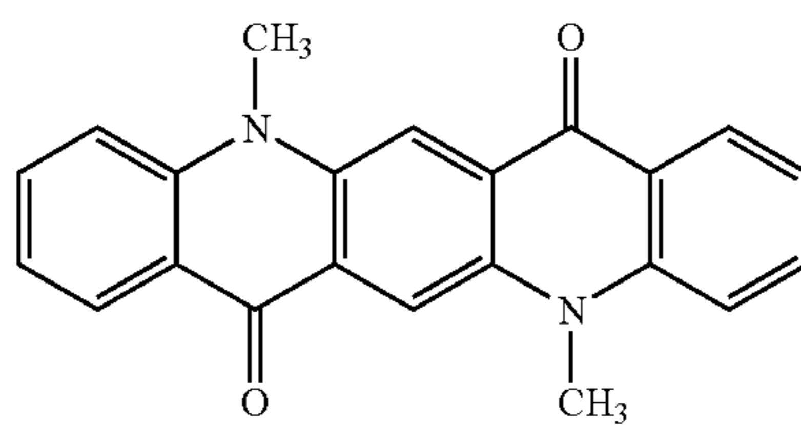
Qd-2
