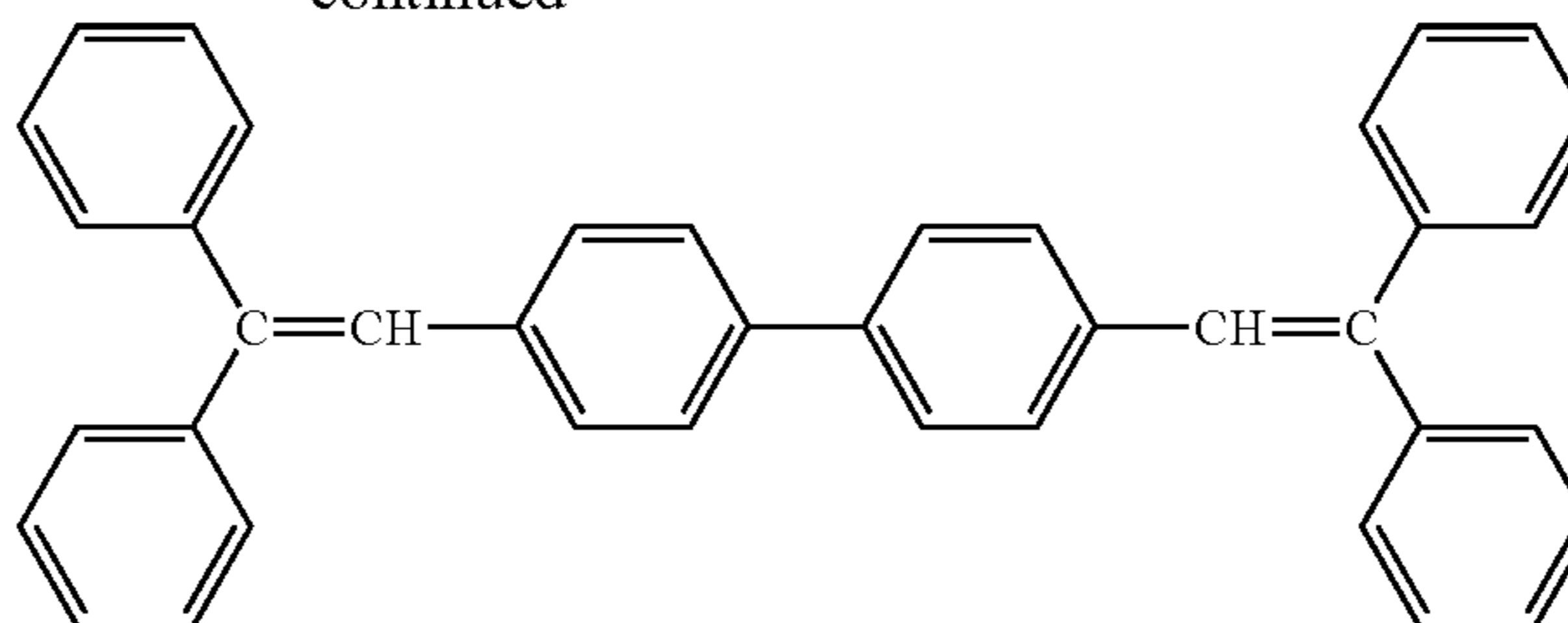
DPVBi
