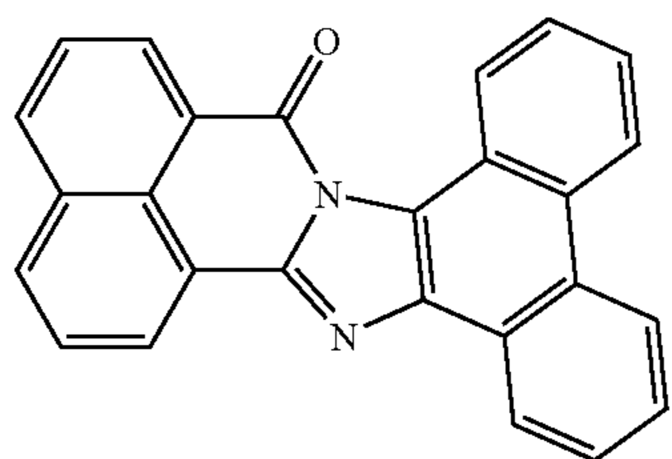
P1
