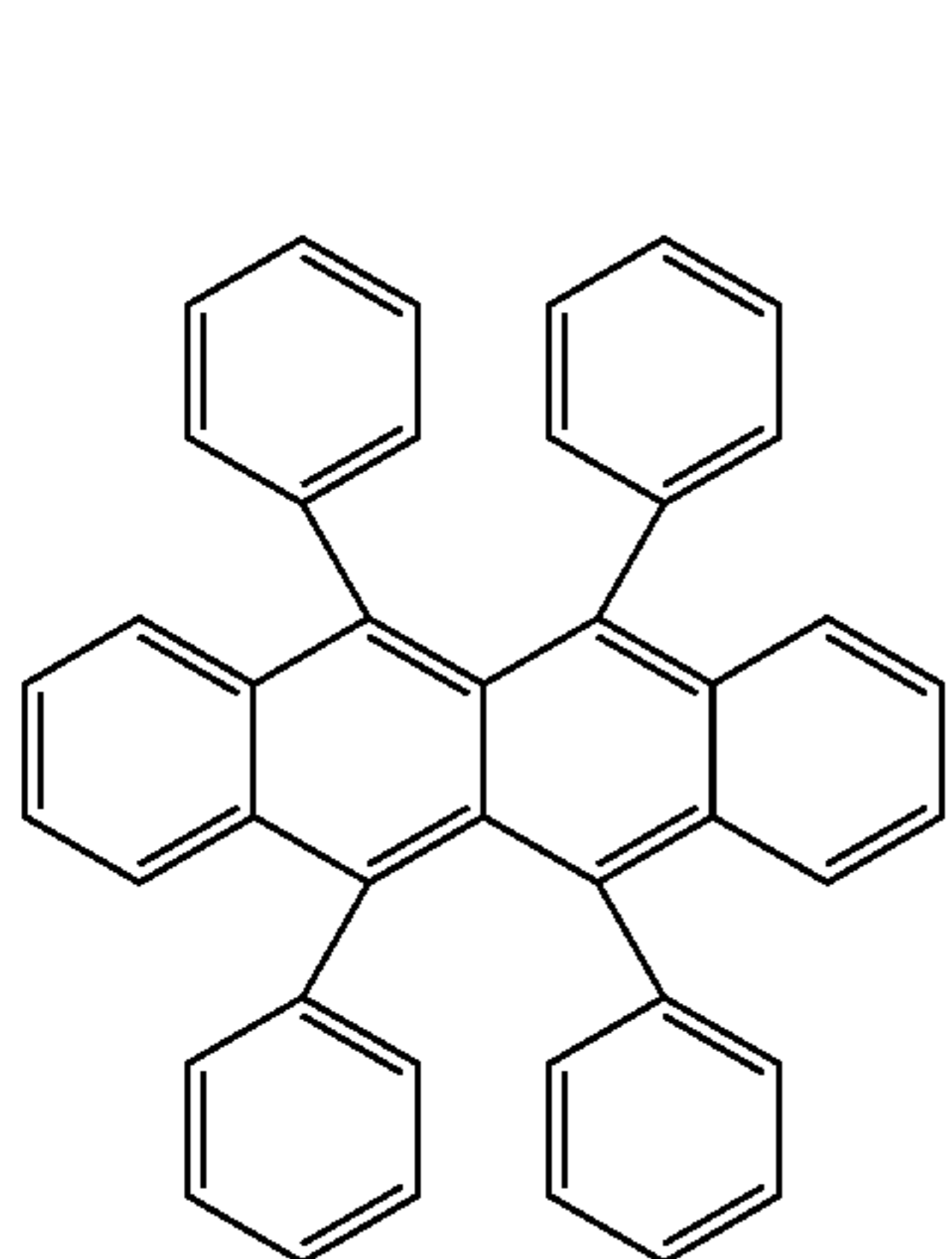
DCM1
