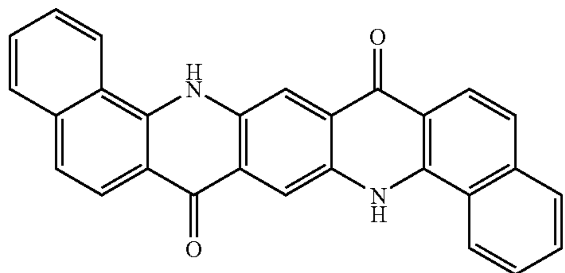
Qd-3
