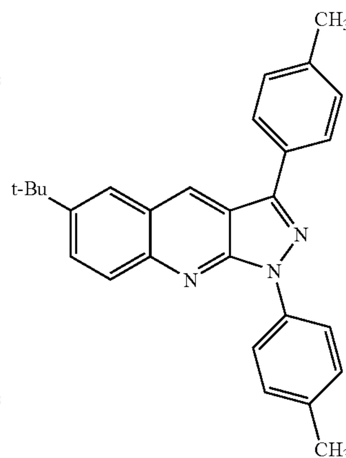
PZ10
