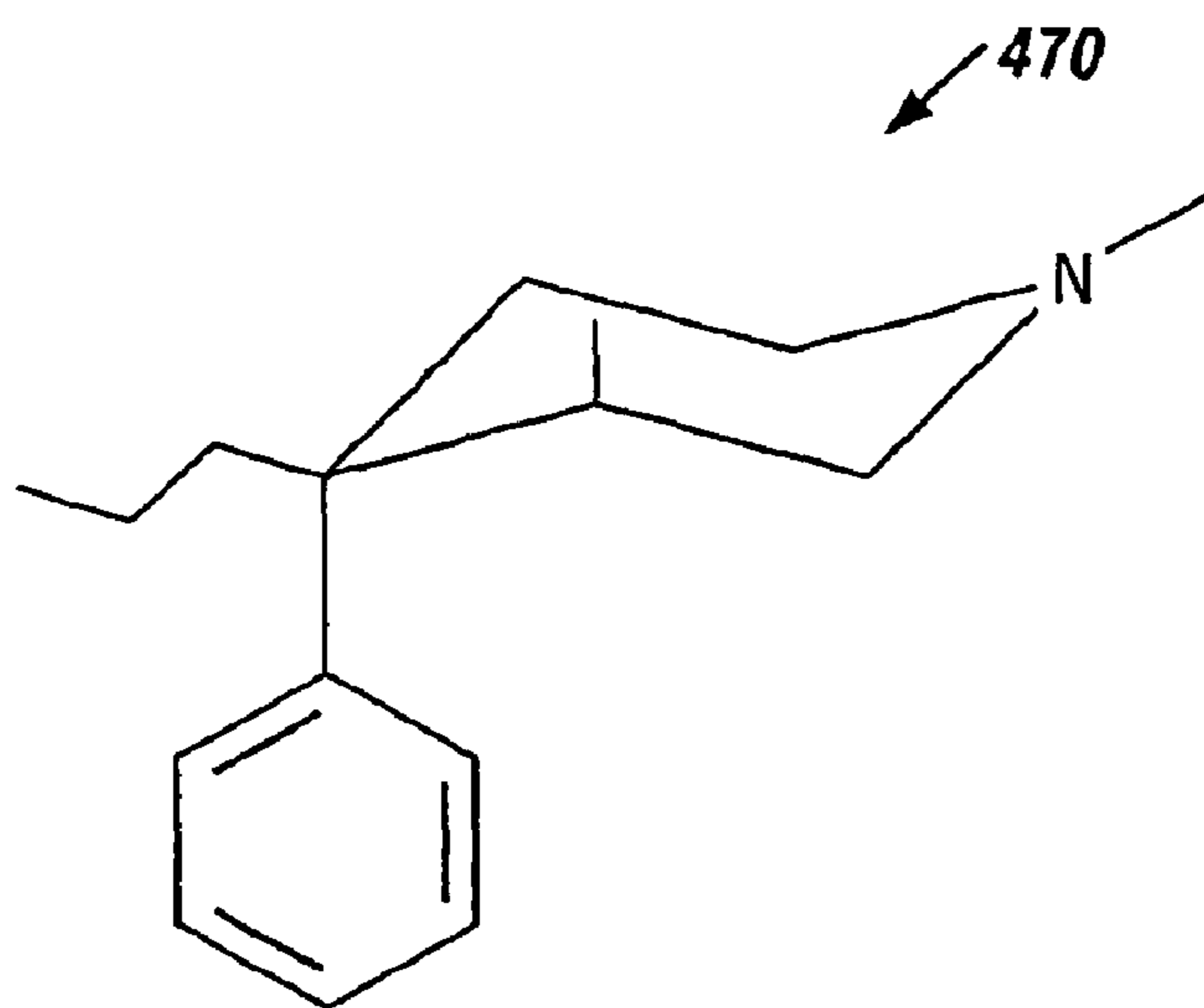
Picenadol (-) Isomer
