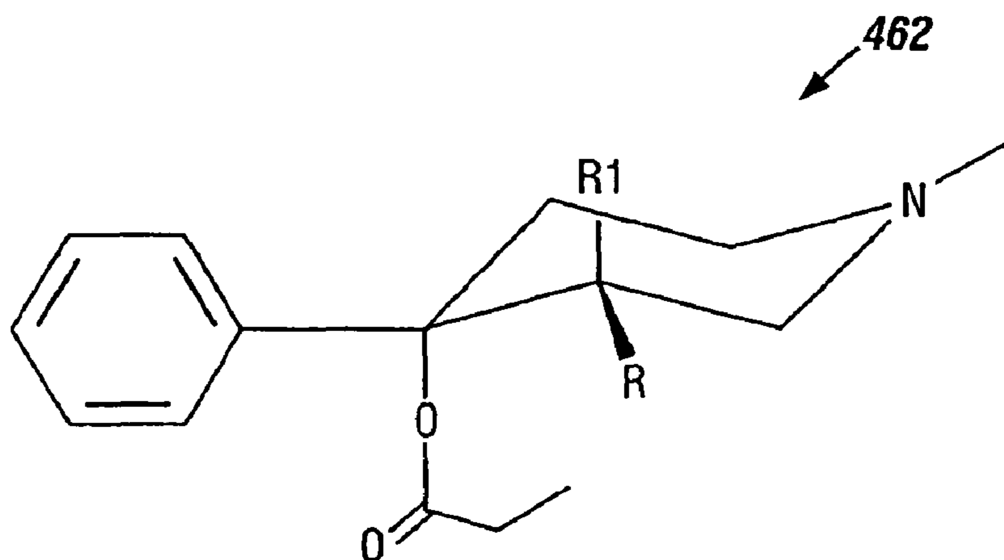
Prodine (-) Isomer
