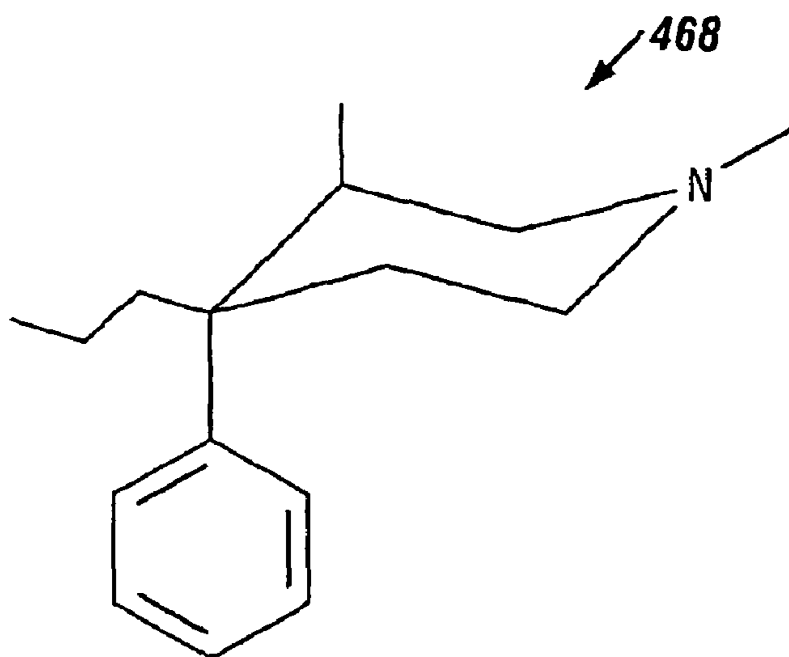
Picenadol (+) Isomer
