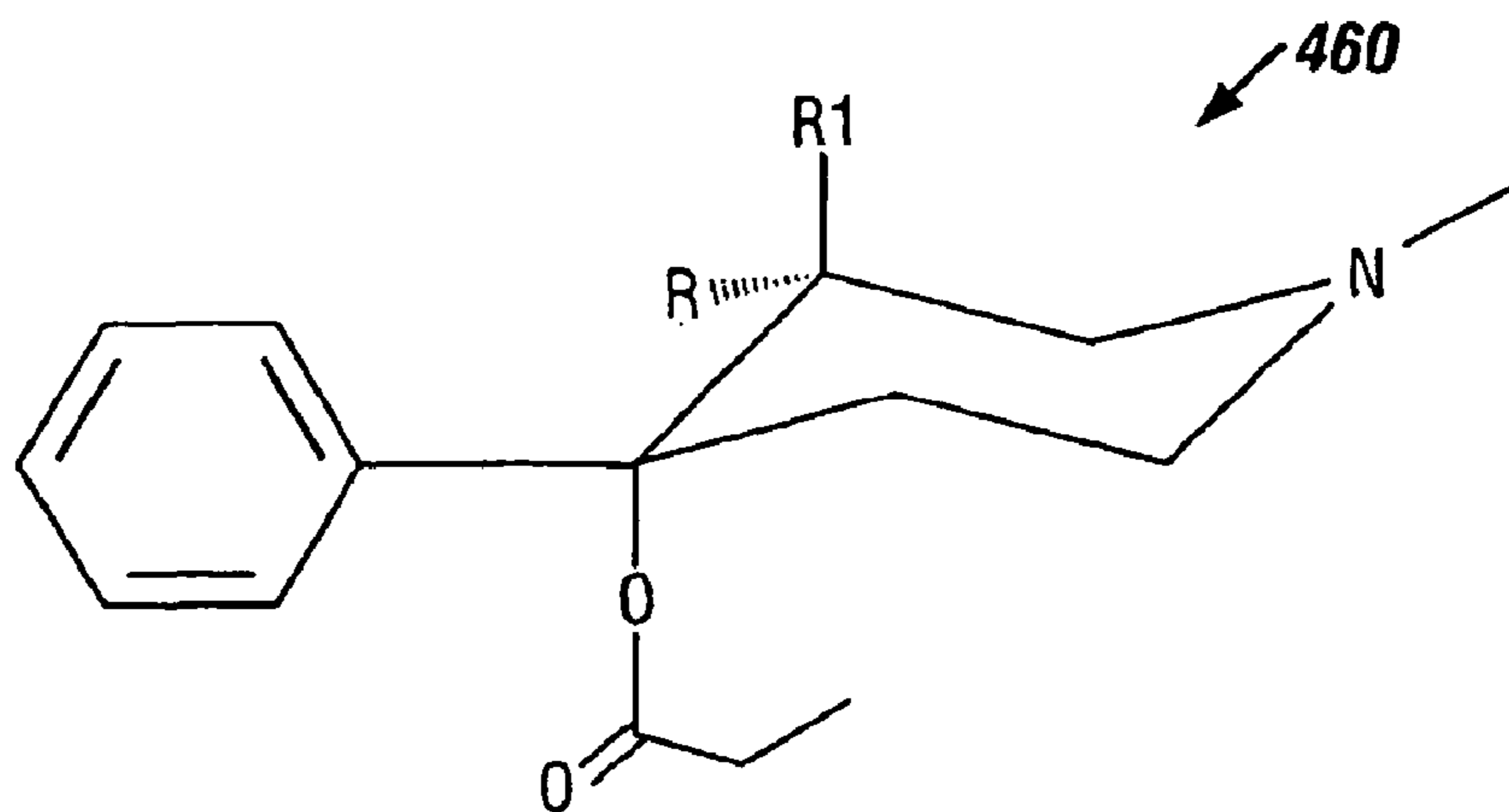
Prodine (+) Isomer
