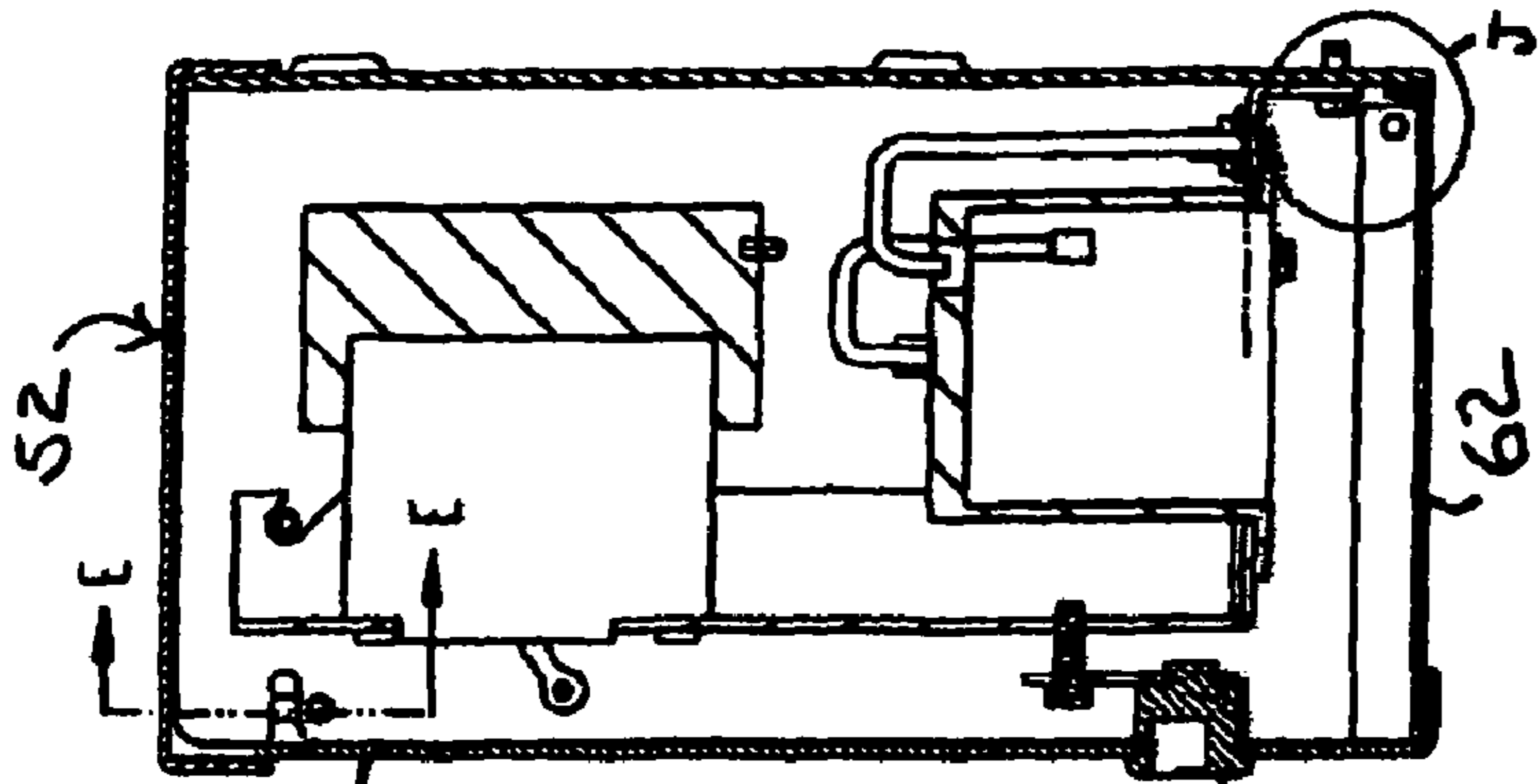
SECTION A-A FIG. 11
