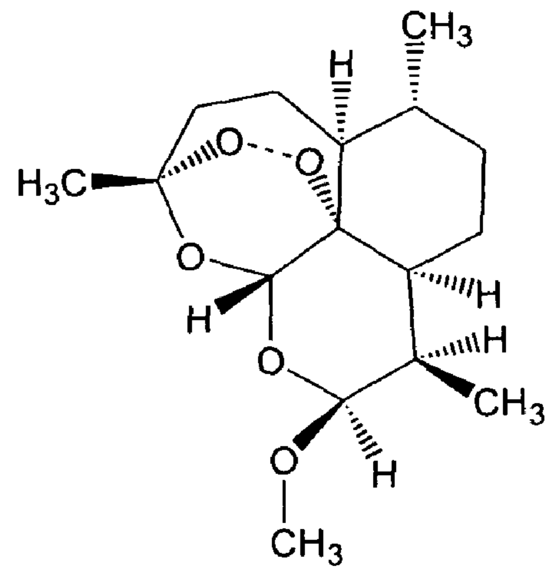
Artemether
