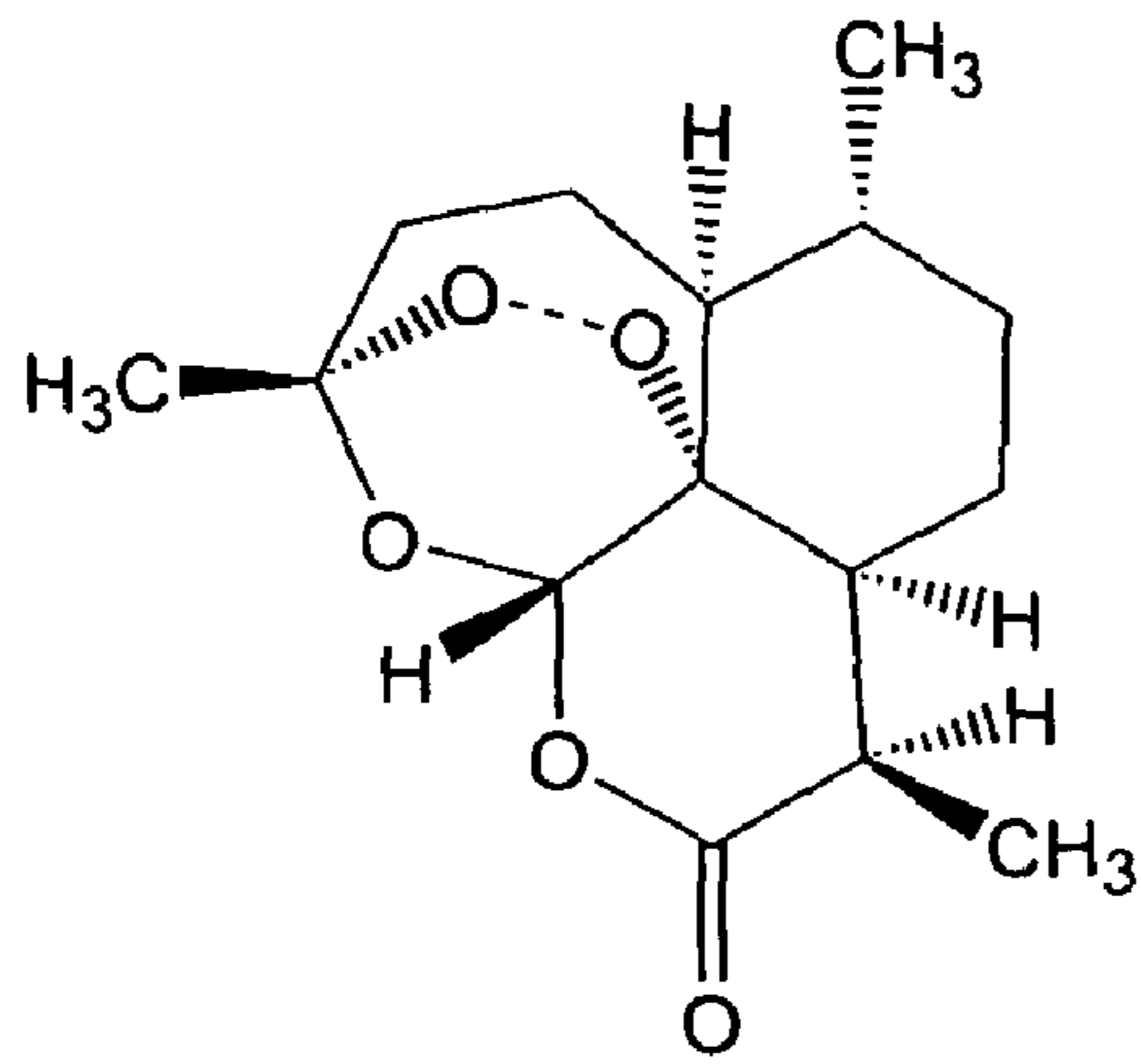
Artemisinin
