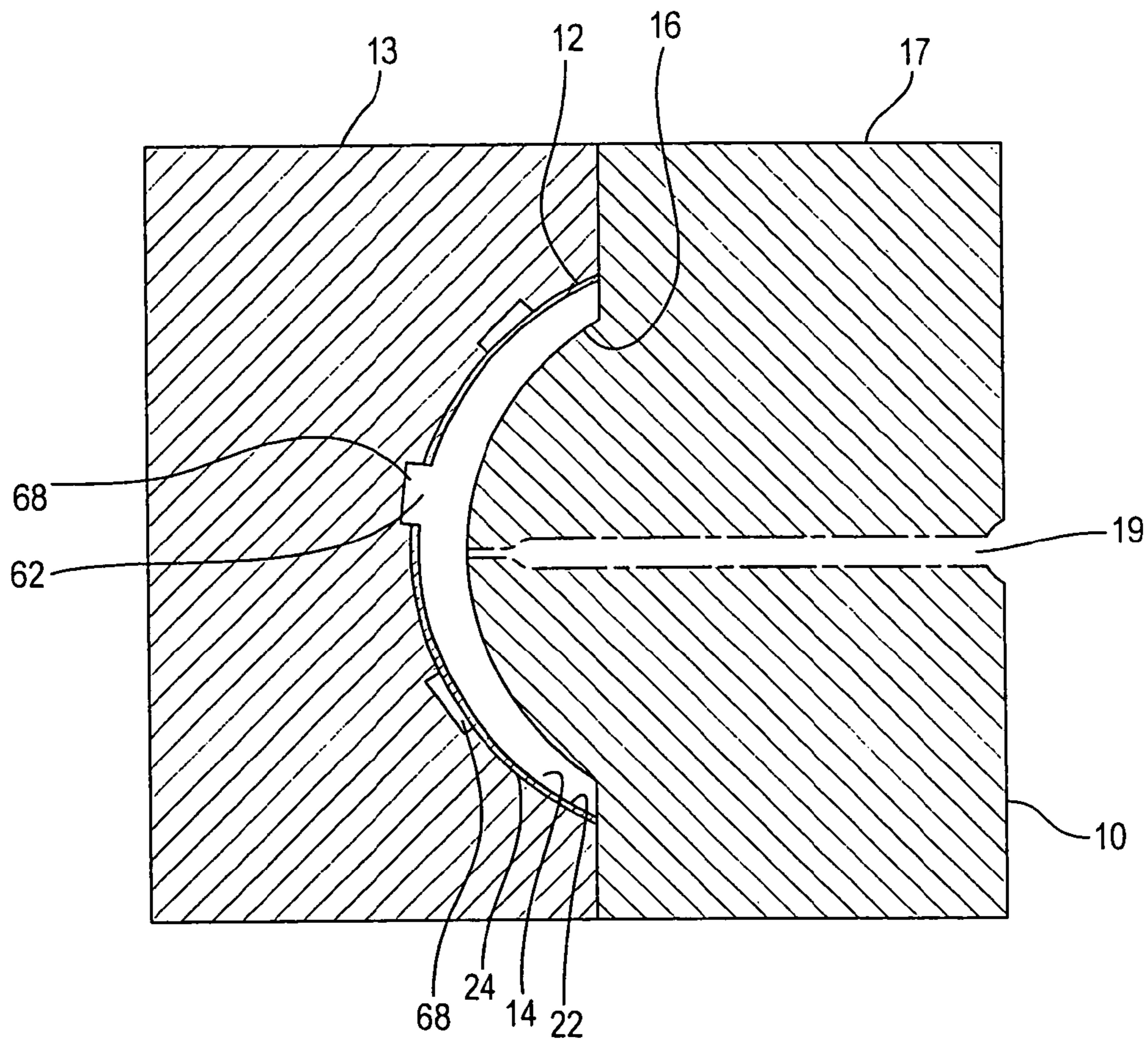
FIG. 12A
