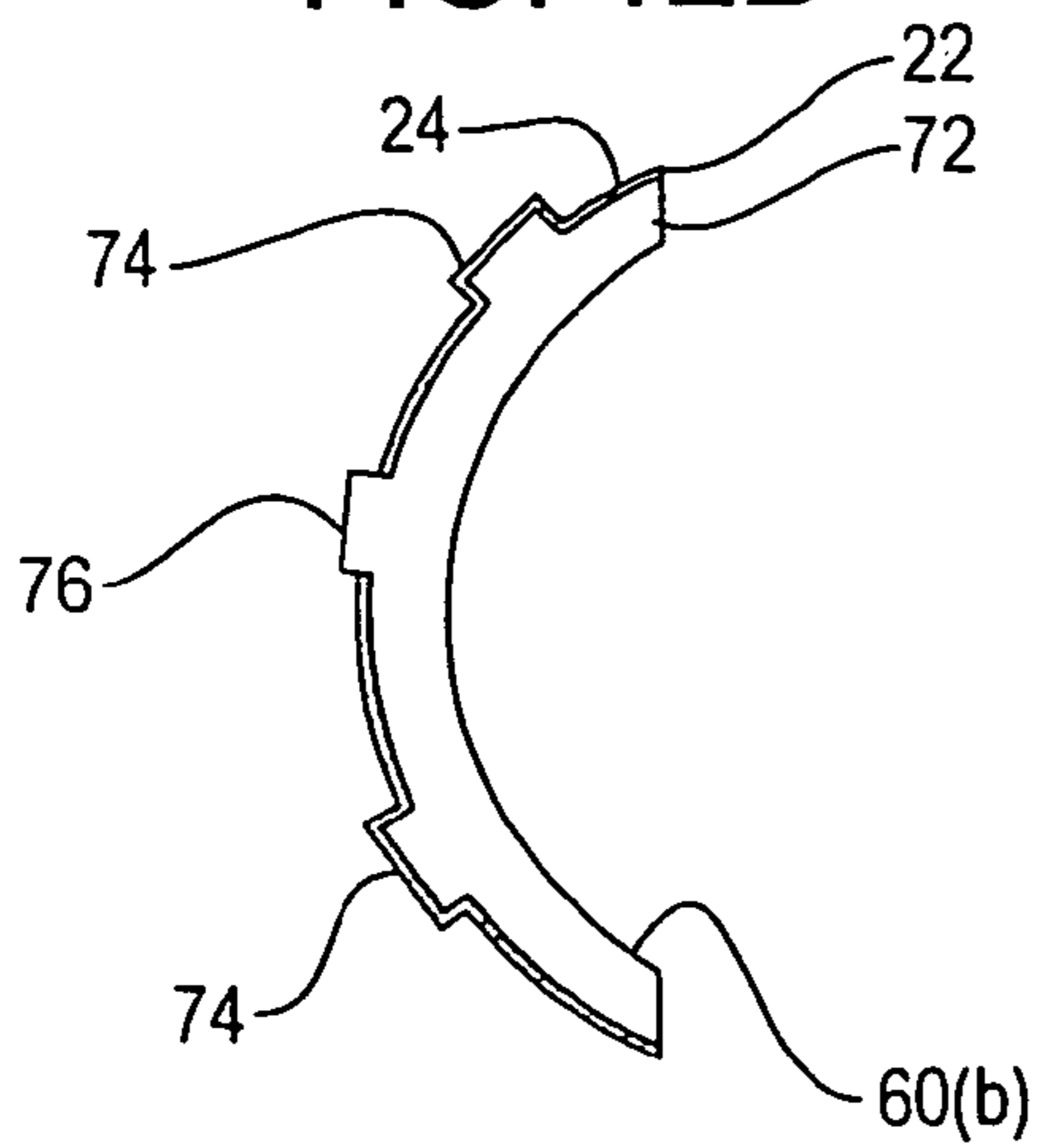
FIG. 12B
