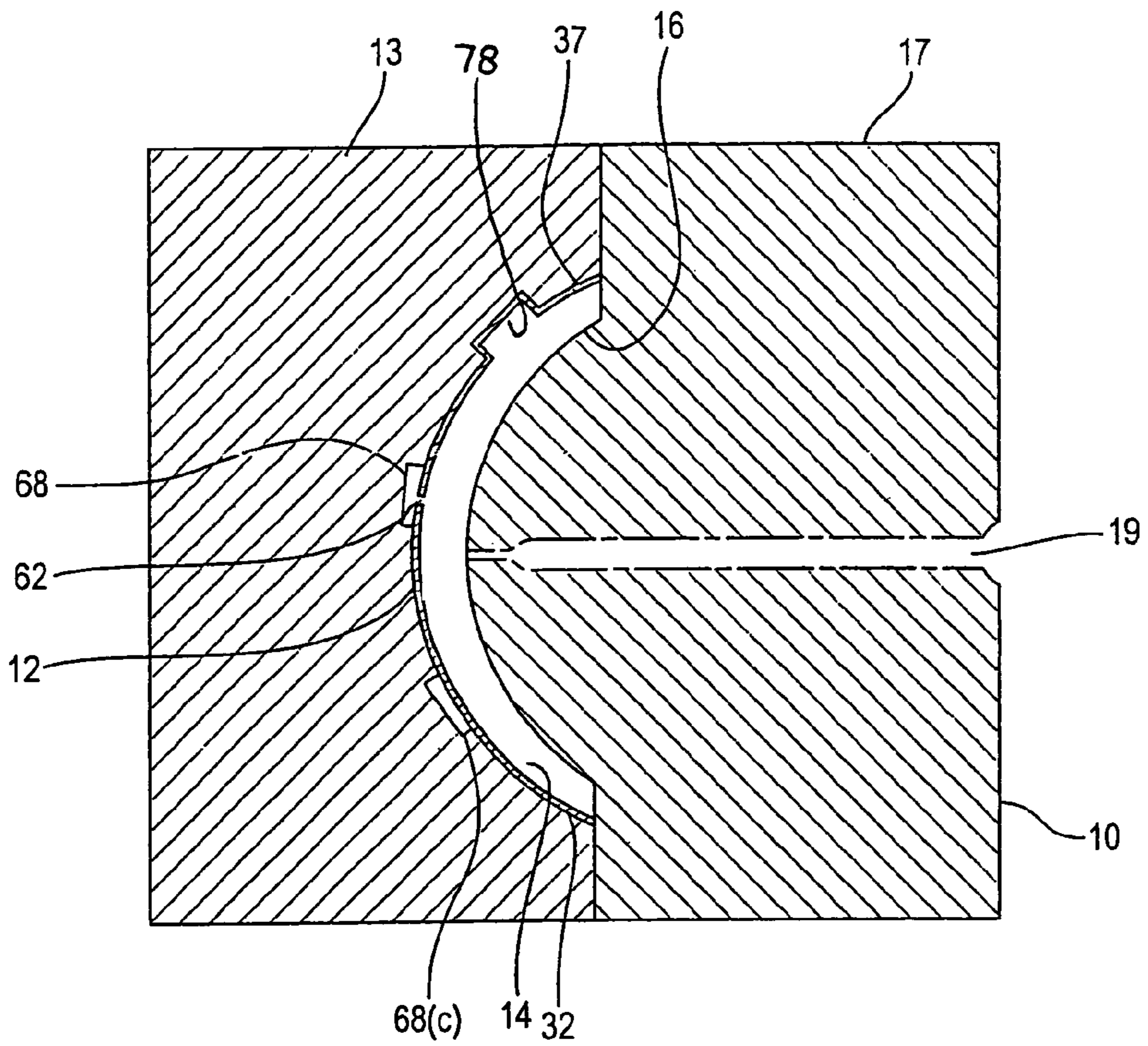
FIG. 13A
