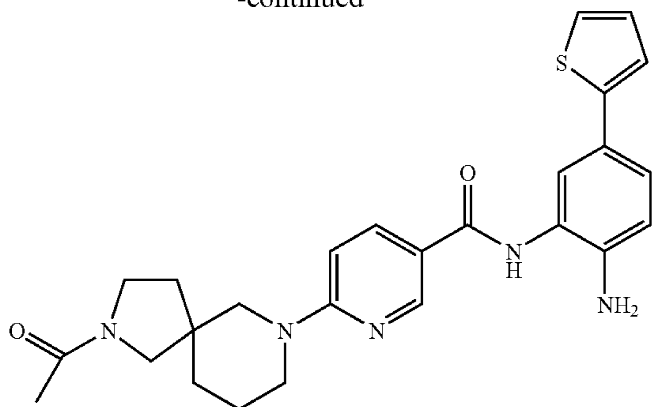
6-(2-Acetyl)-2,7-diazaspiro[4.5]dec-7-yl-N-[2-amino-5-(2-thienyl)phenyl]-nicotinamide
