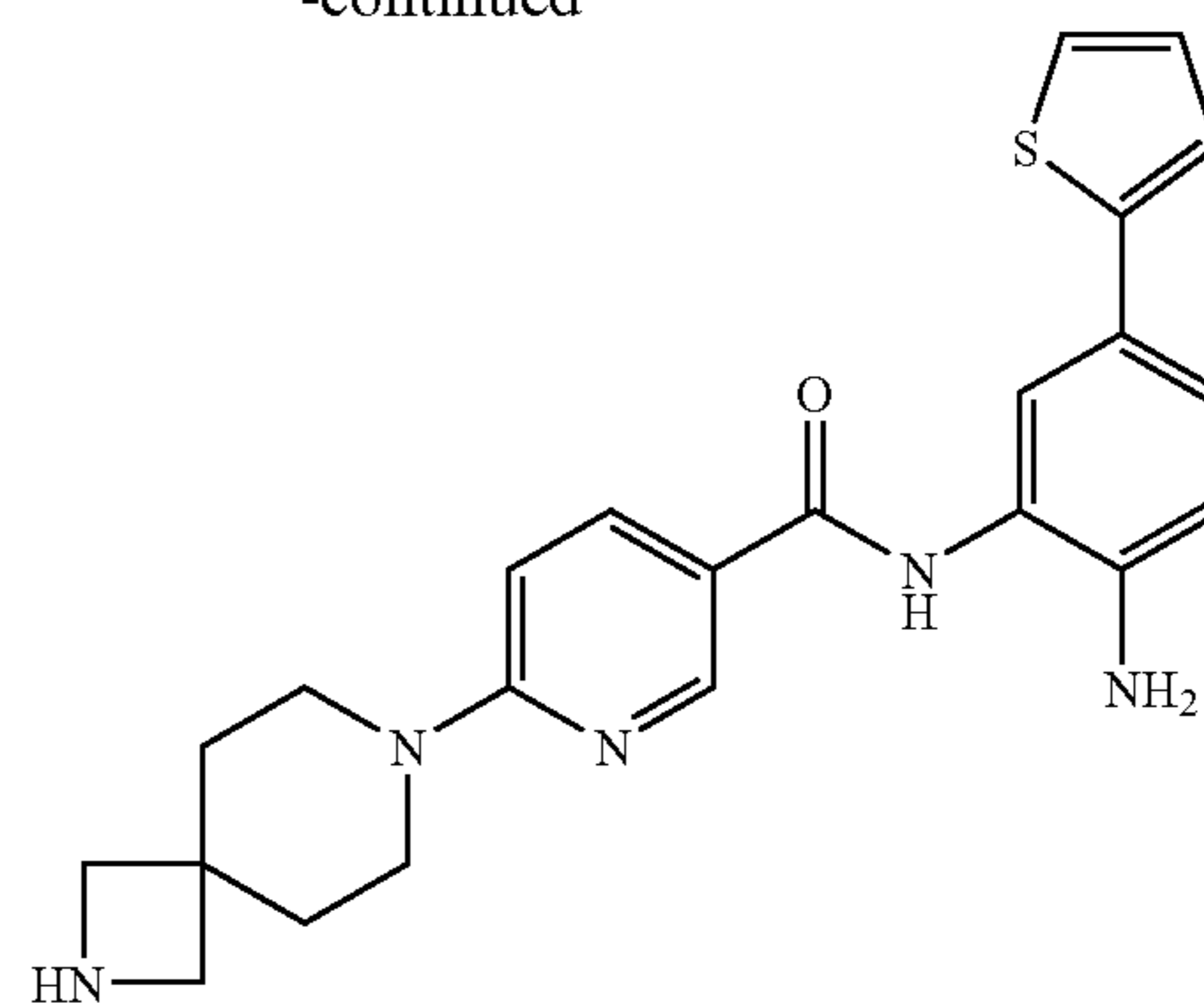
N-[2-amino-5-(2-thienyl)phenyl]-6-(2,7-diazaspiro[3.5]non-7-yl)nicotinamide
