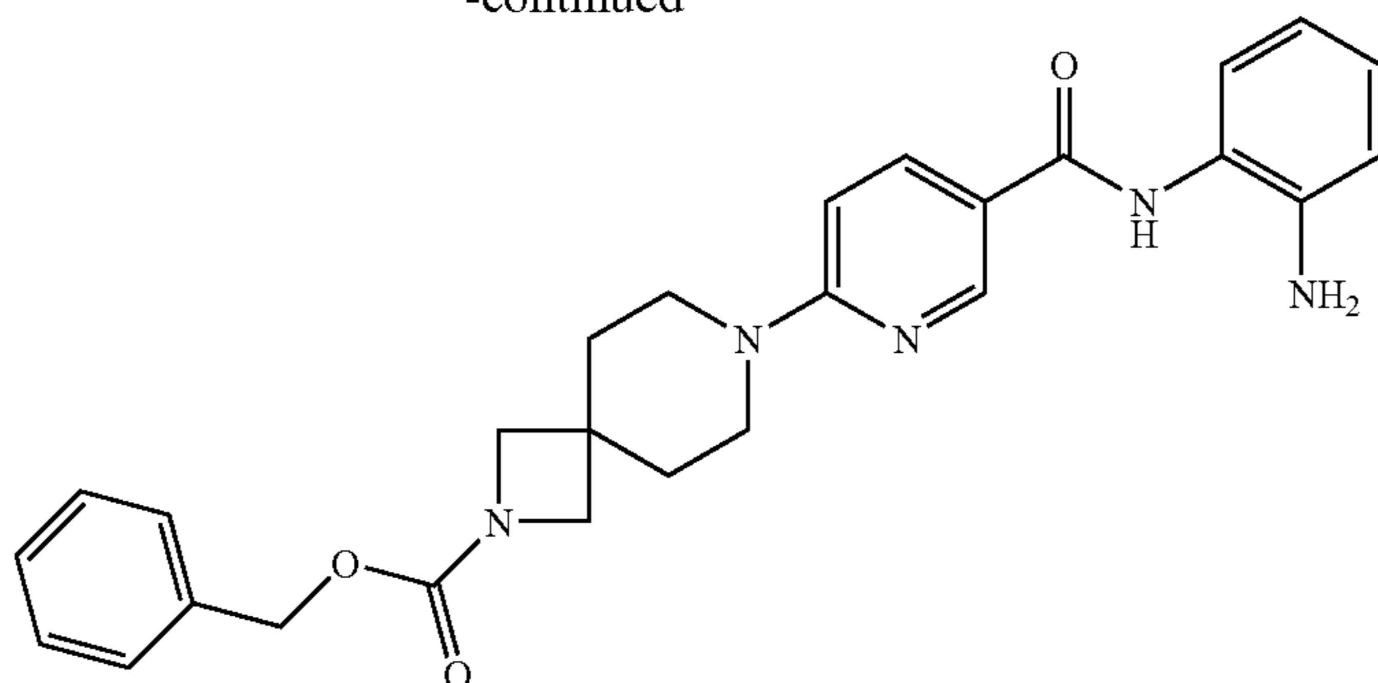
Benzyl 7-(5-((2-aminophenyl)amino)carbonyl)pyridine-2-yl)-2,7-diazaspiro[3.5]nonane-2-carboxylate
