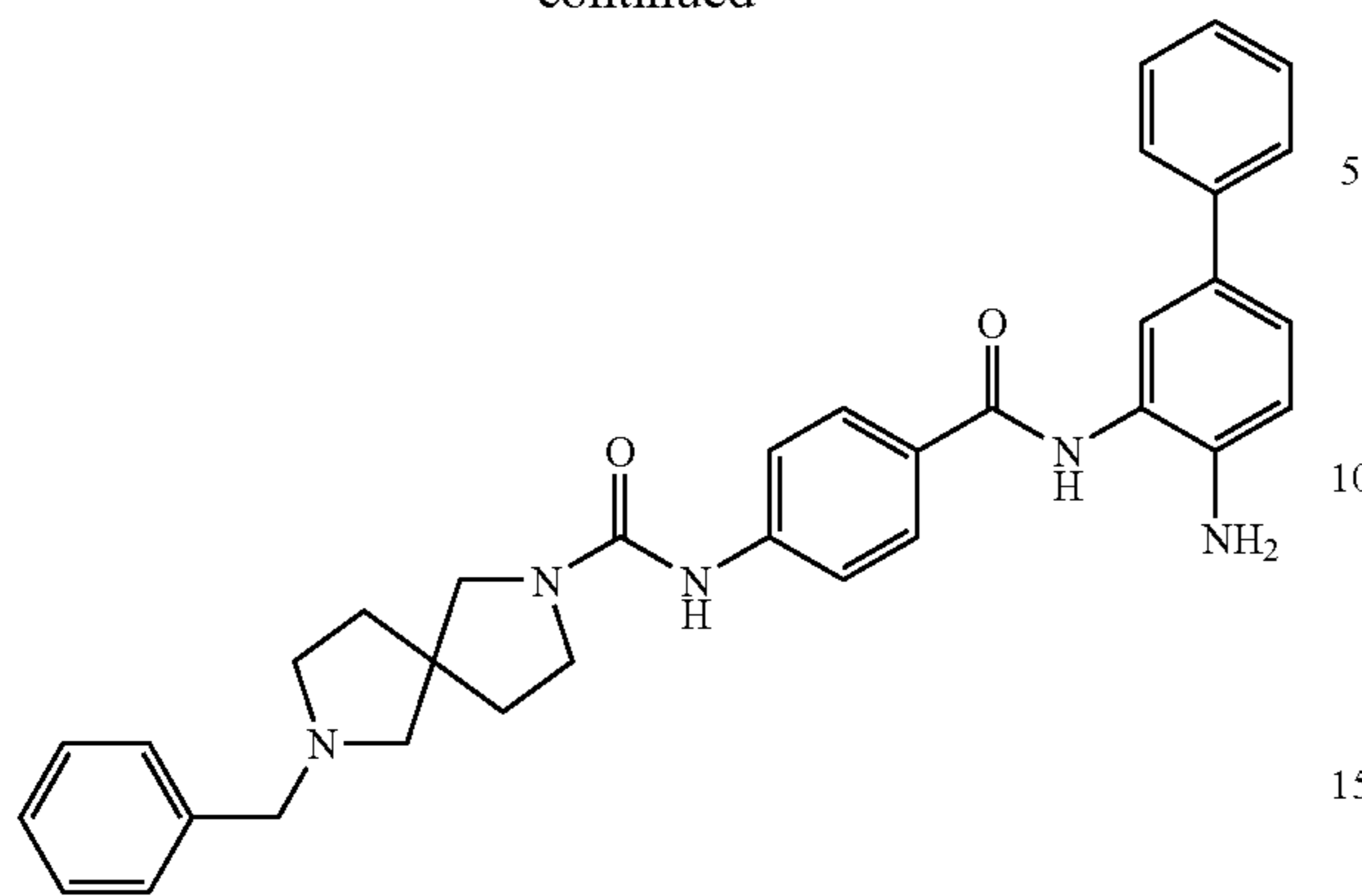
N-(4-[[[4-aminobiphenyl-3-yl)amino]carbonyl]phenyl)-7-benzyl-2,7-diazaspiro[4.4]nonane-2-carboxamide
