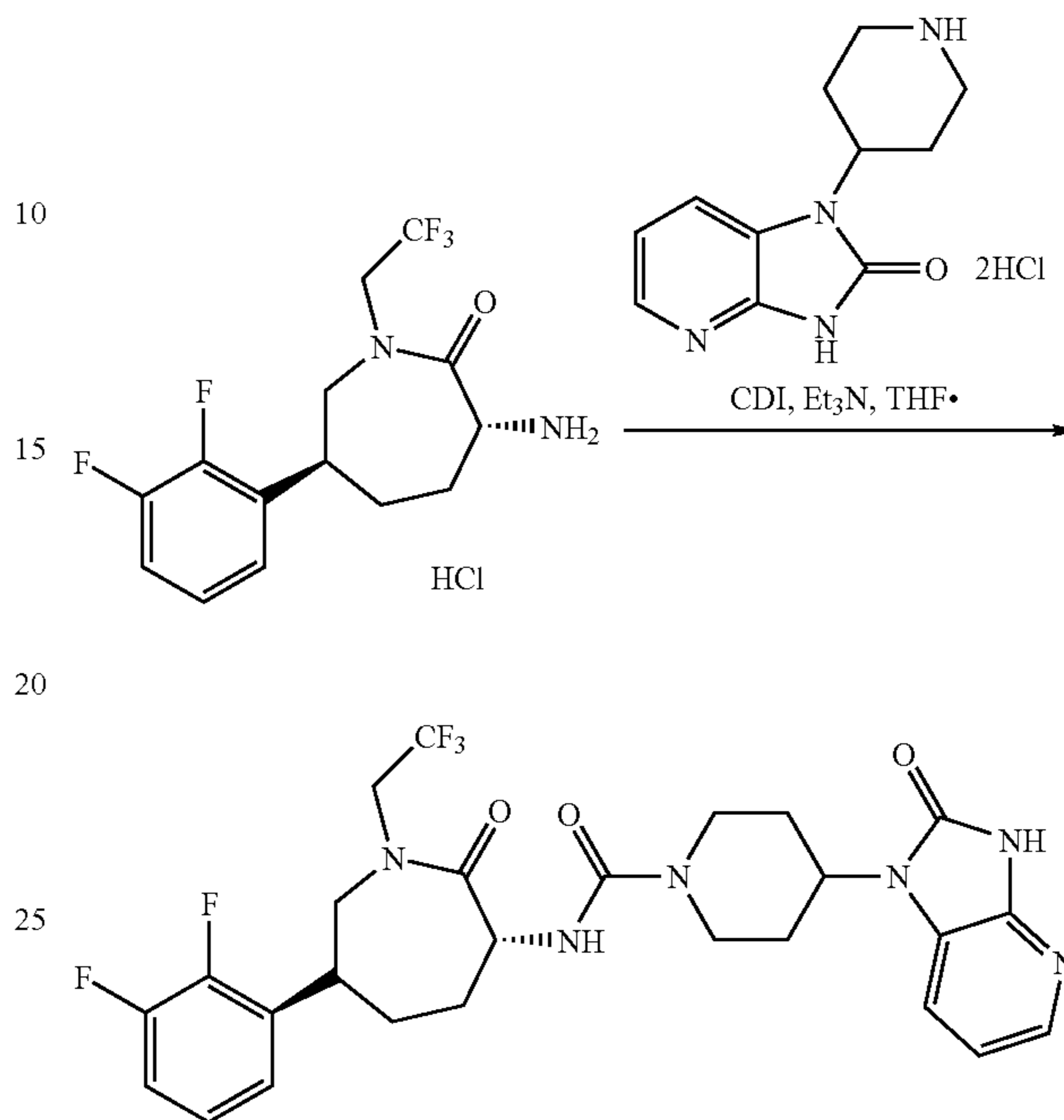
Scheme 1A
