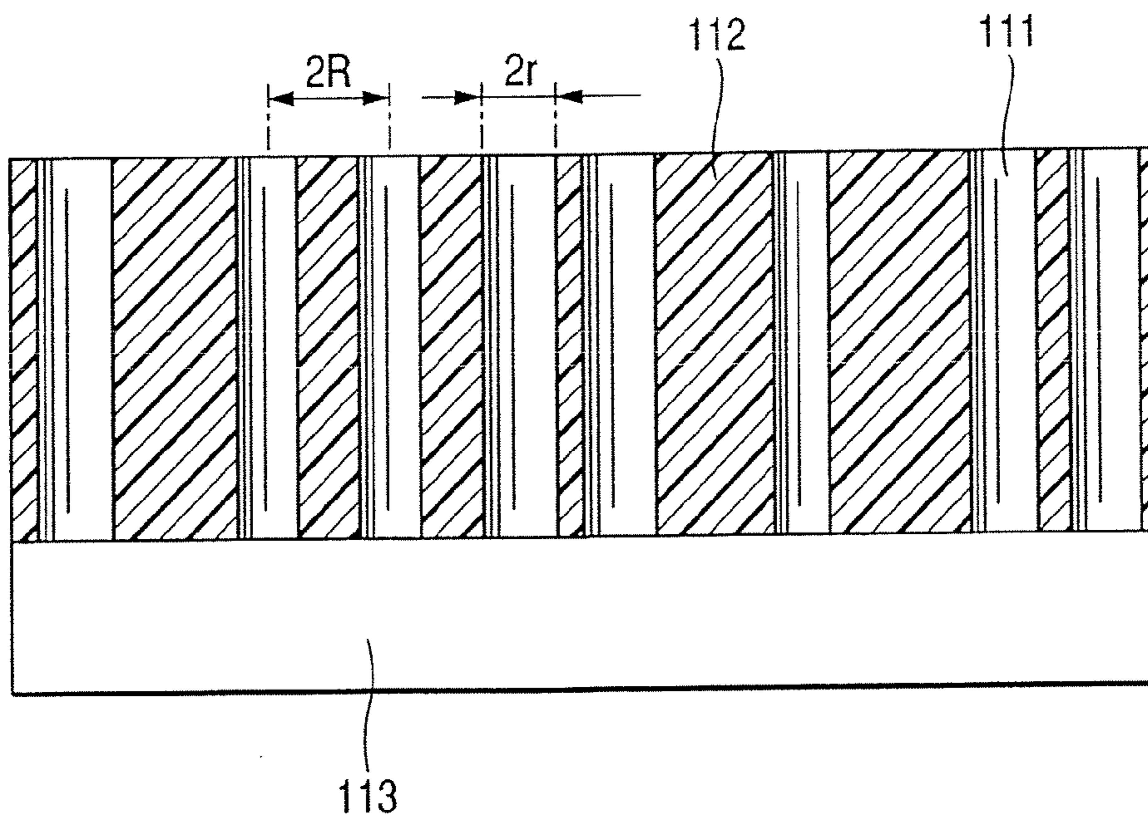
FIG. 2B
