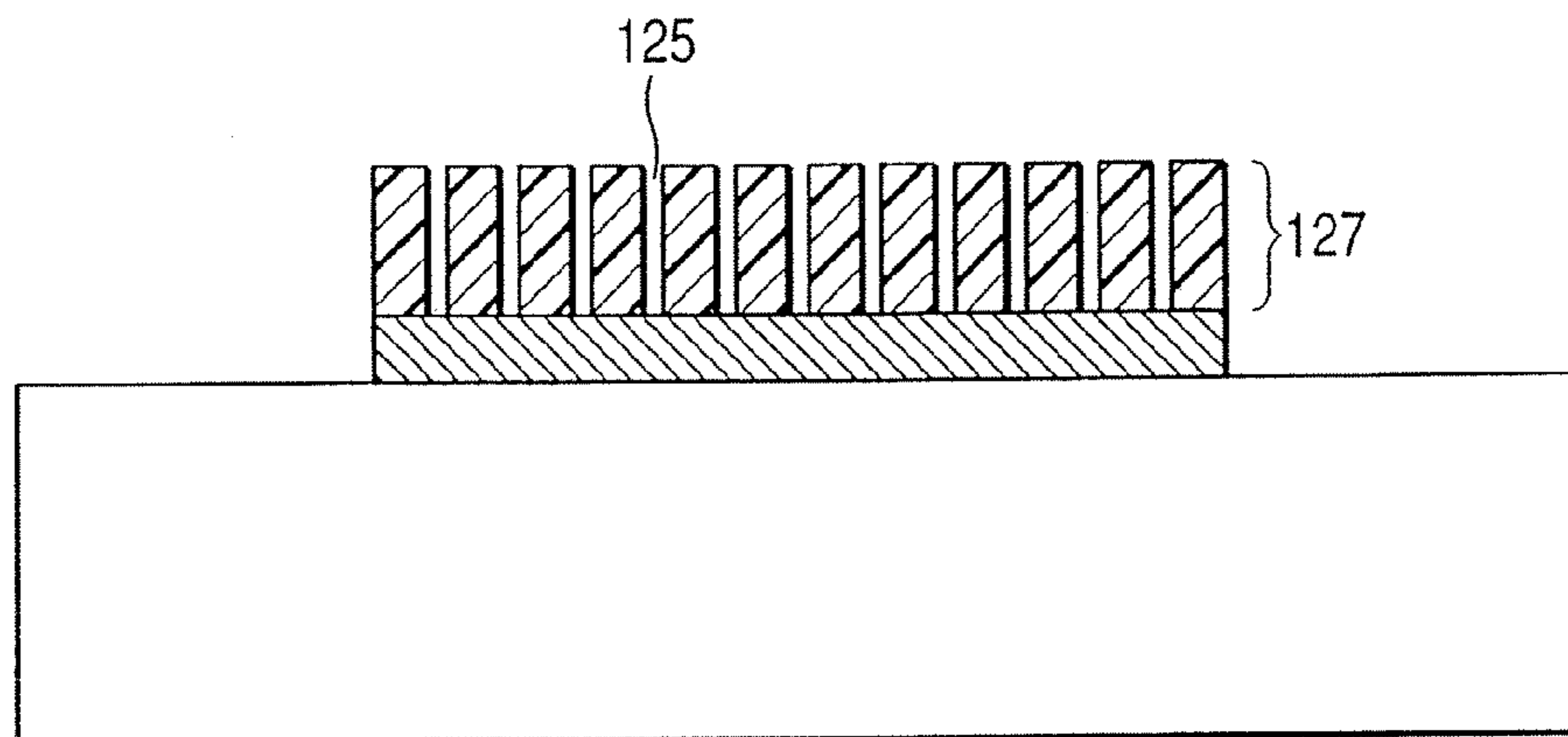
FIG. 7E
