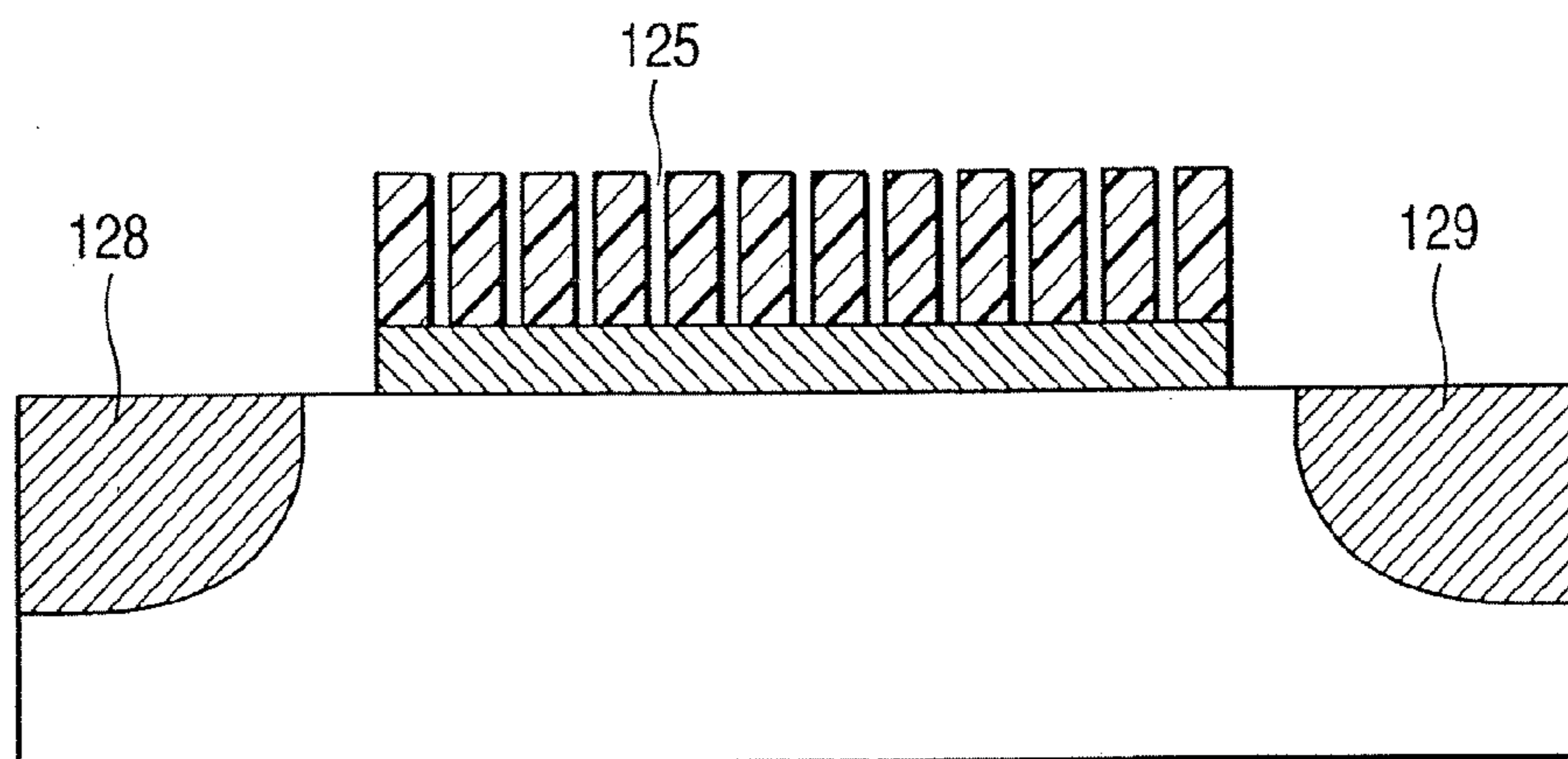
FIG. 7F
