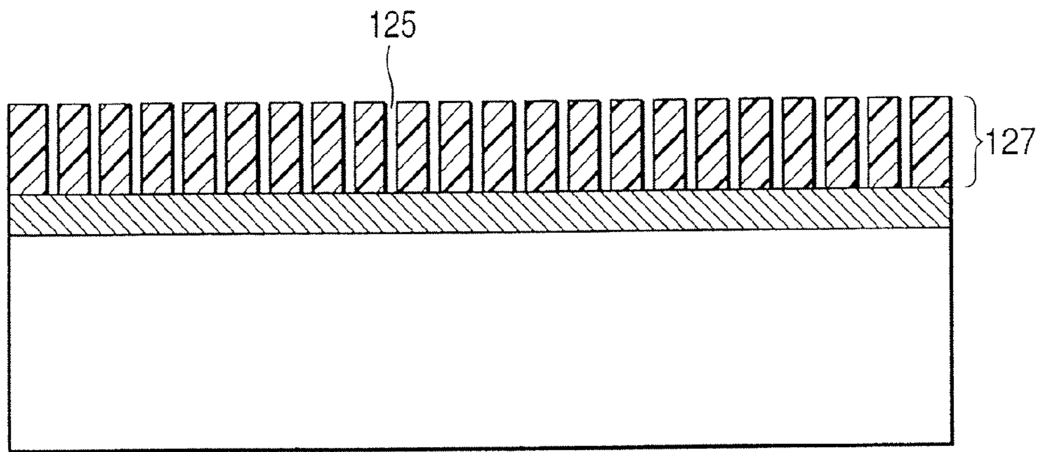
FIG. 7D
