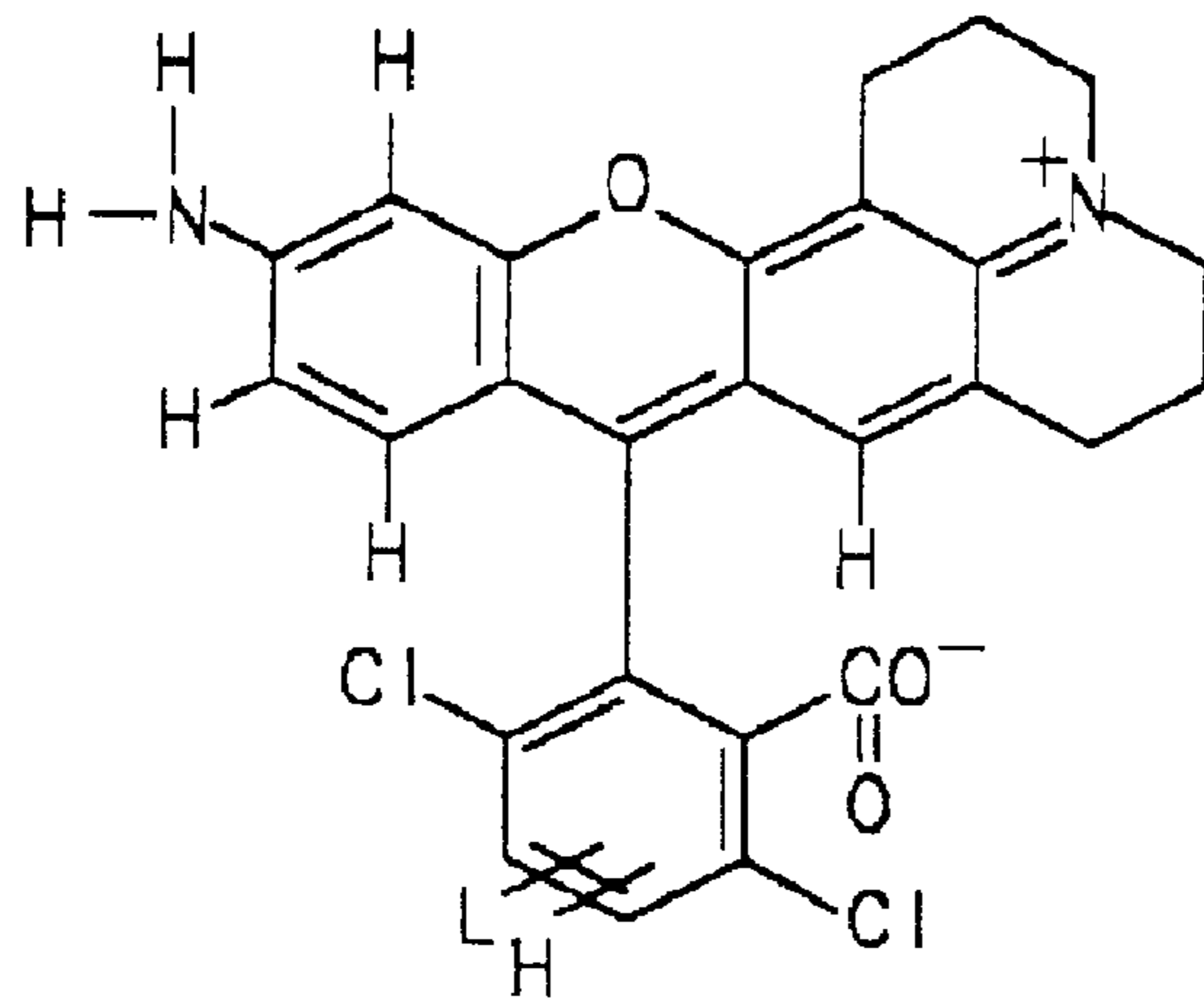
FIG. 3B-D
