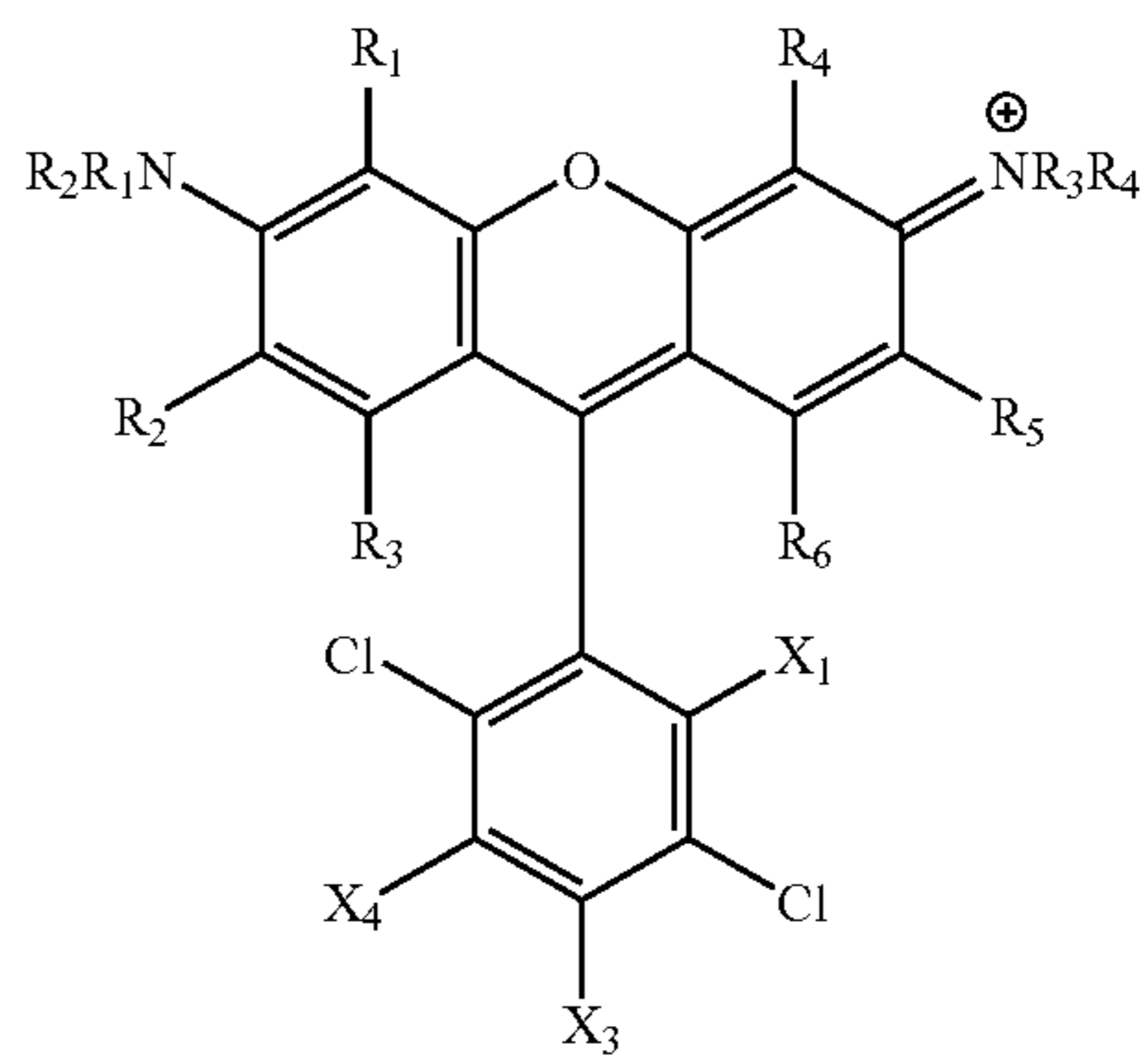
4,7-Dichlororhodamine
