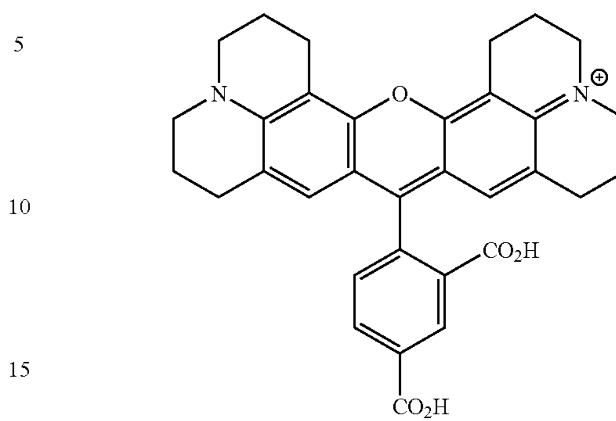
ROX
