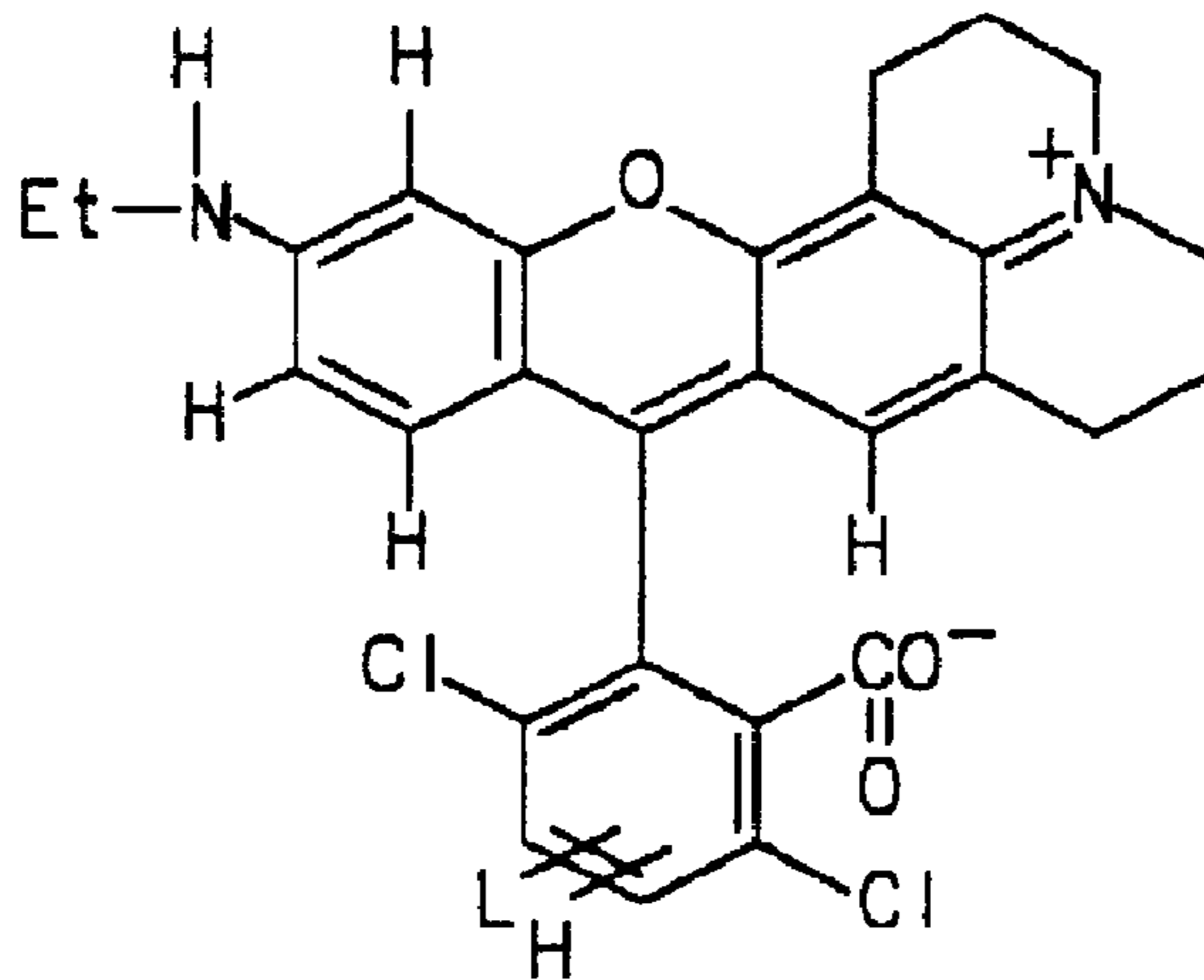
FIG. 3B-E
