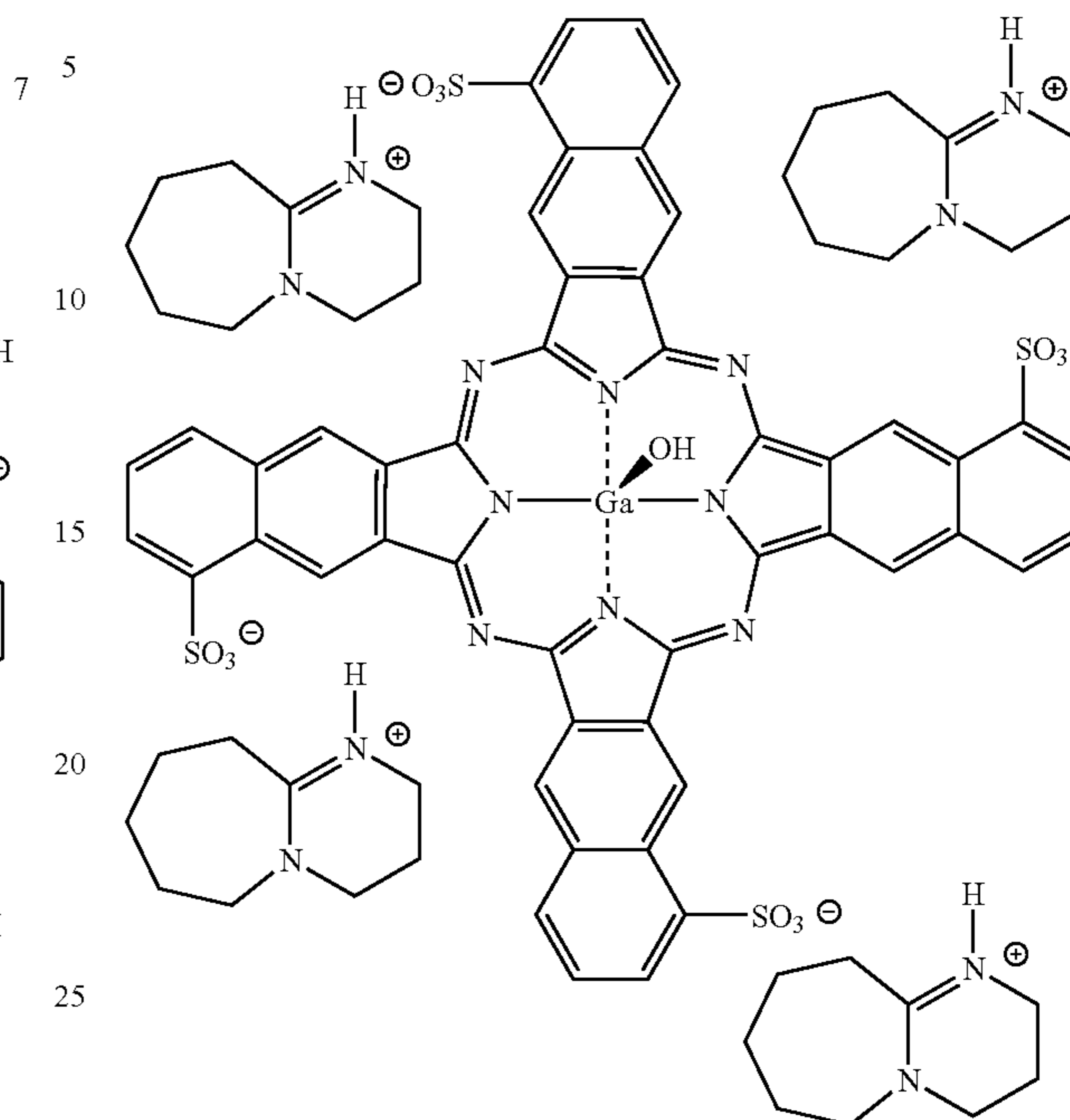
(a) Tetrapyrrolyl 5
