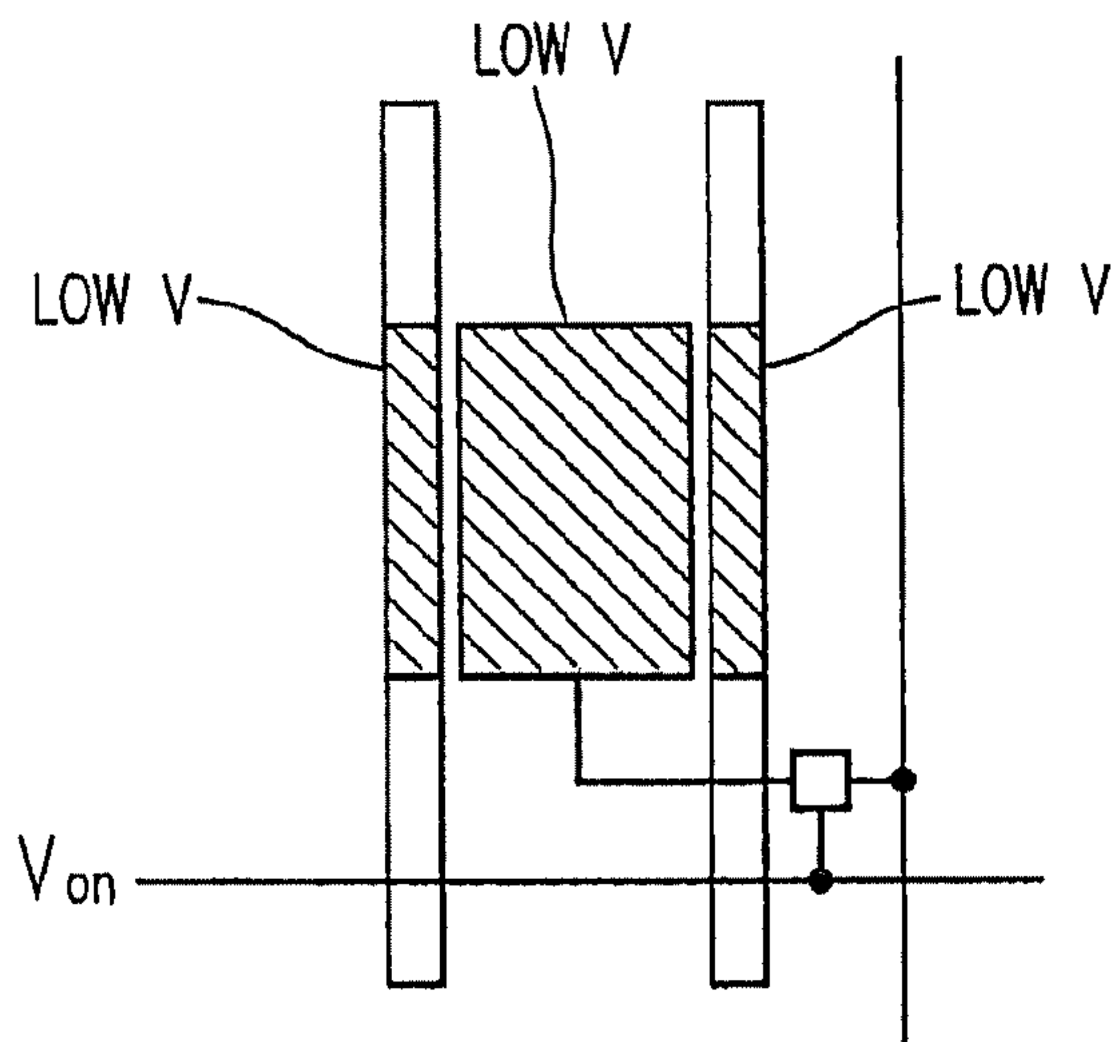
COLOR STATE FIG. 12C-1
