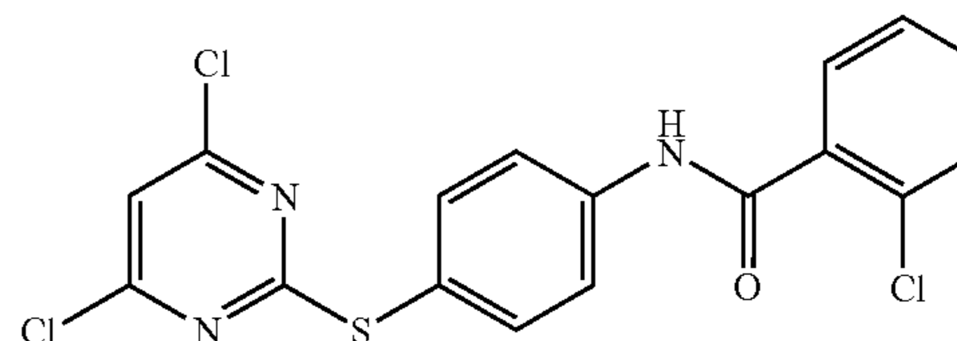
2-Chloro-N-[4-(4,6-dichloro-pyrimidin-2-ylsulfanyl)-phenyl]-benzamide
