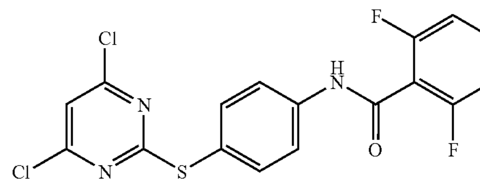
2,6-Difluoro -N-[4-(4,6-dichloro-pyrimidin-2-ylsulfanyl)-phenyl]-benzamide
