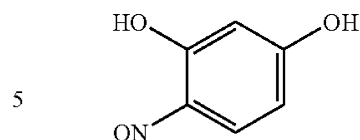
a 4-nitrosoresorcinol
