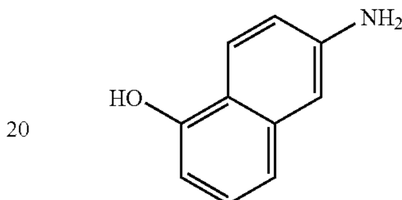
a 1,6-naphthalenediol
