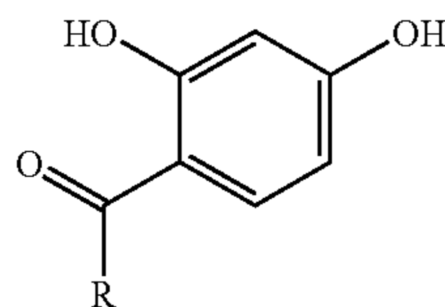
a 4-acylresorcinol
