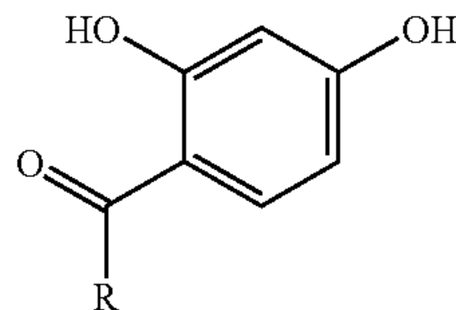
a 4-acylresorcinol
