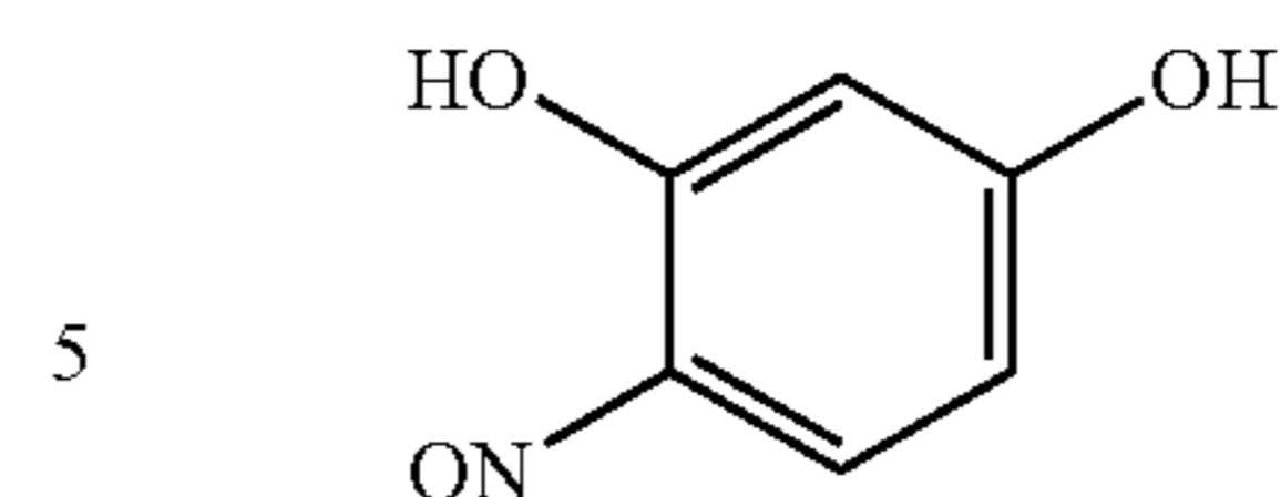
a 4-nitrosoresorcinol
