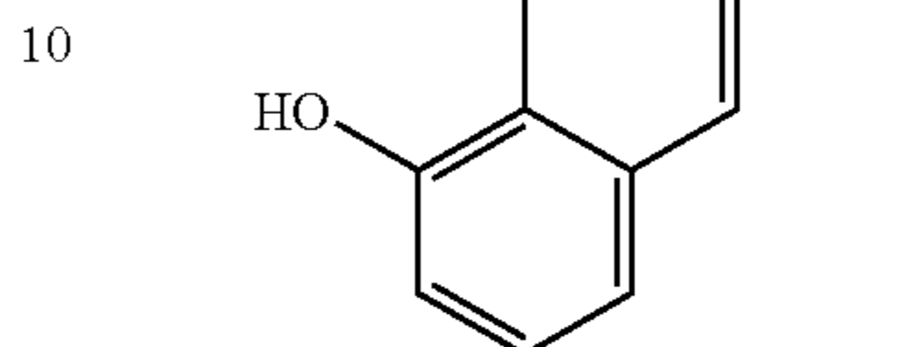
a 1,6-naphthalenediol
