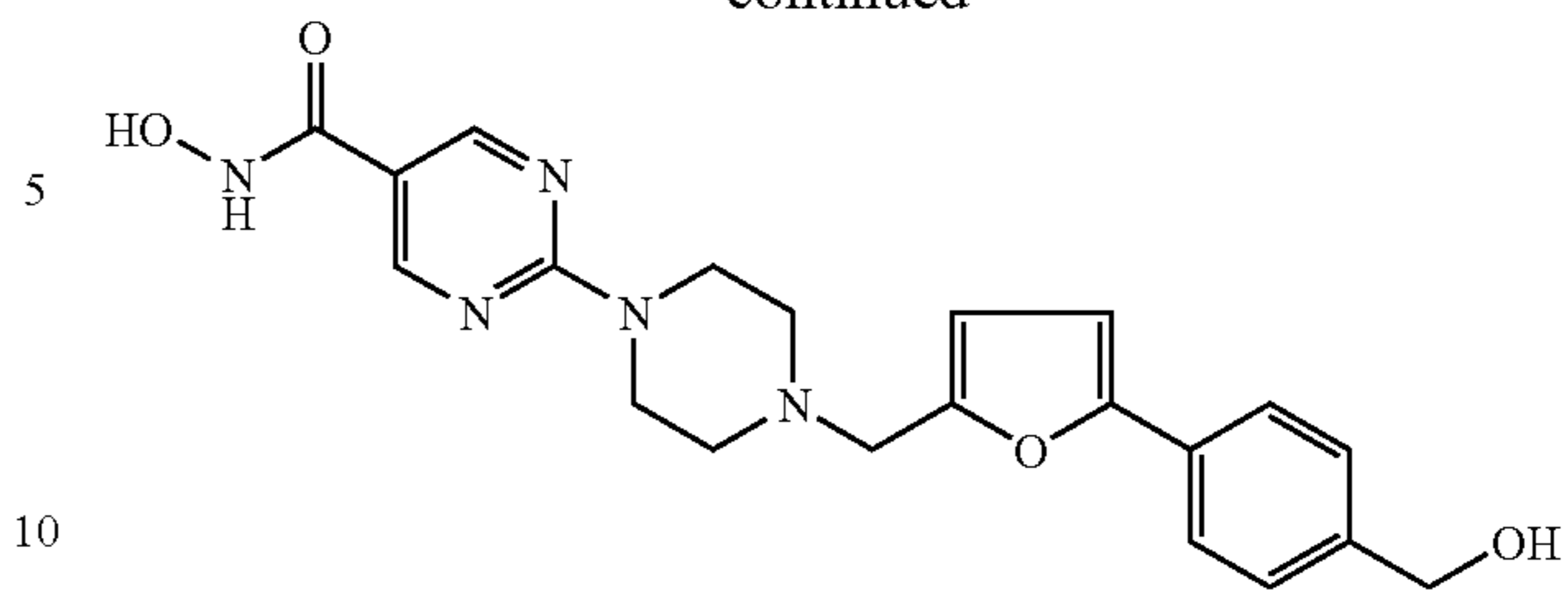
0.83 C_2HF_3O_2 ; Co. No. 5
