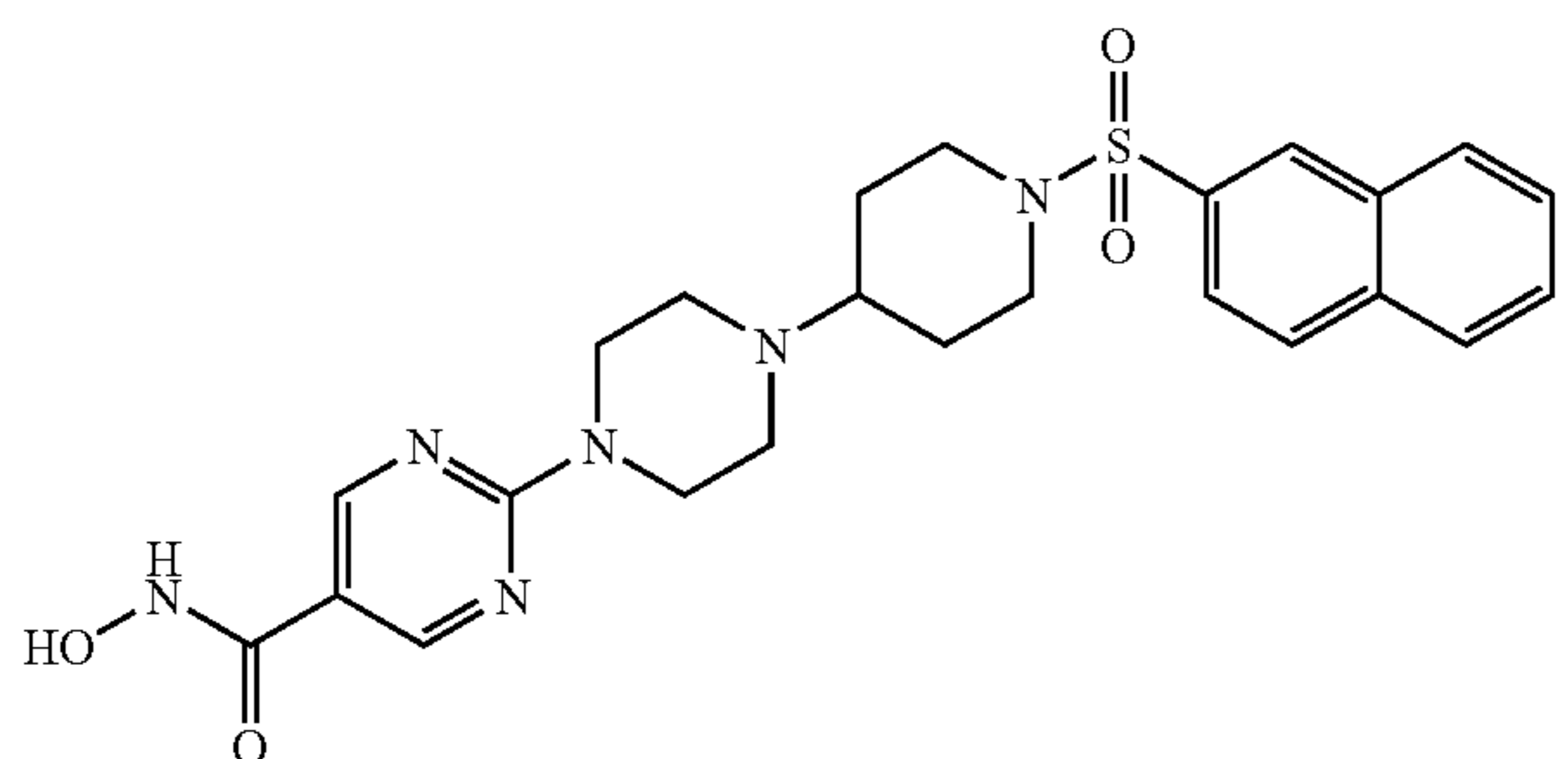
0.91 C_2HF_3O_2 ; Co. No. 3
