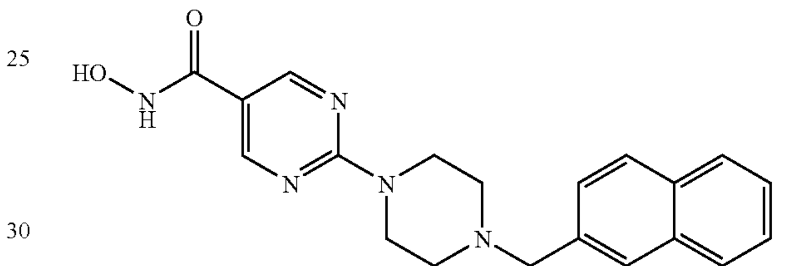
0.83 C_2HF_3O_2 ; Co. No. 6
