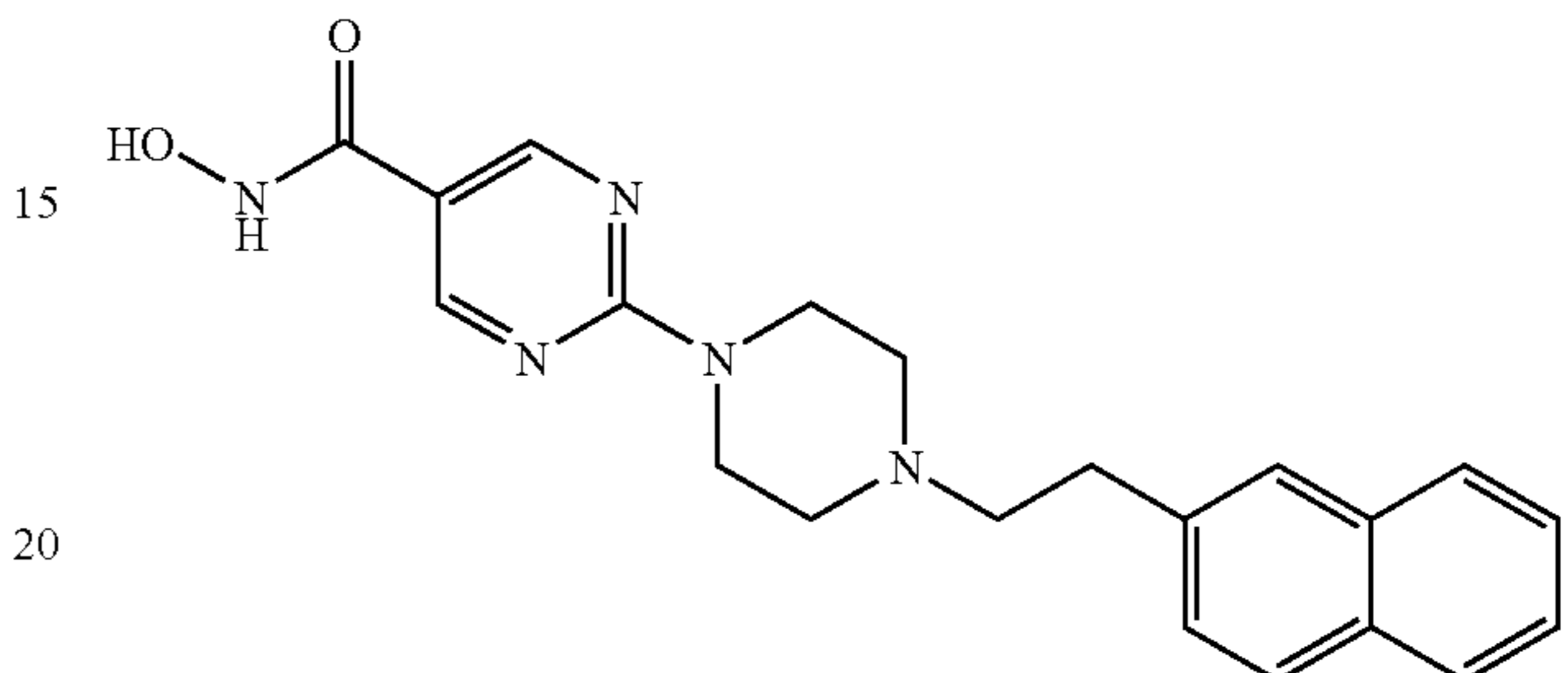
0.79 C_2HF_3O_2 ; Co. No. 7
