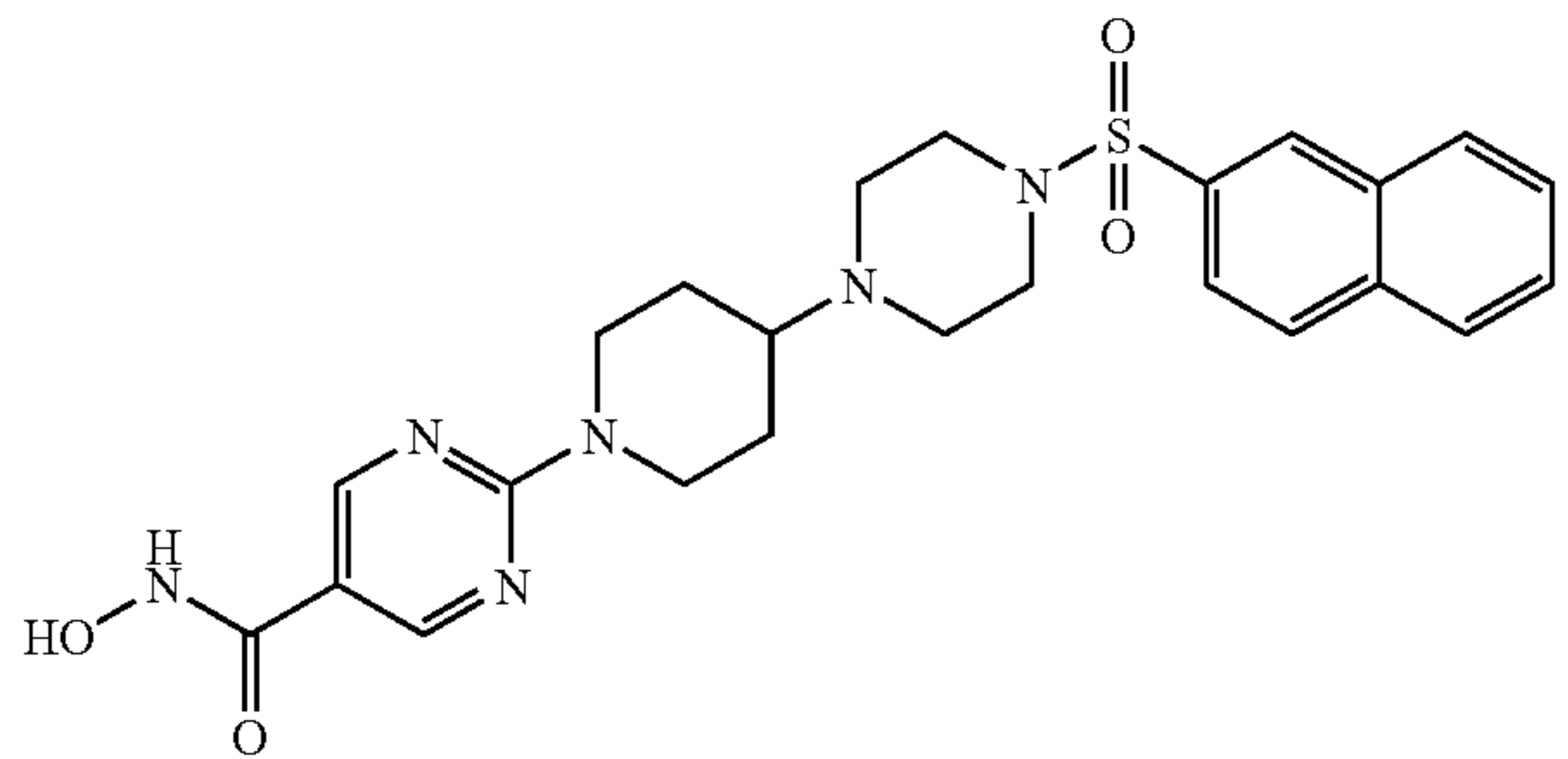
0.86 C_2HF_3O_2 ; Co. No. 4
