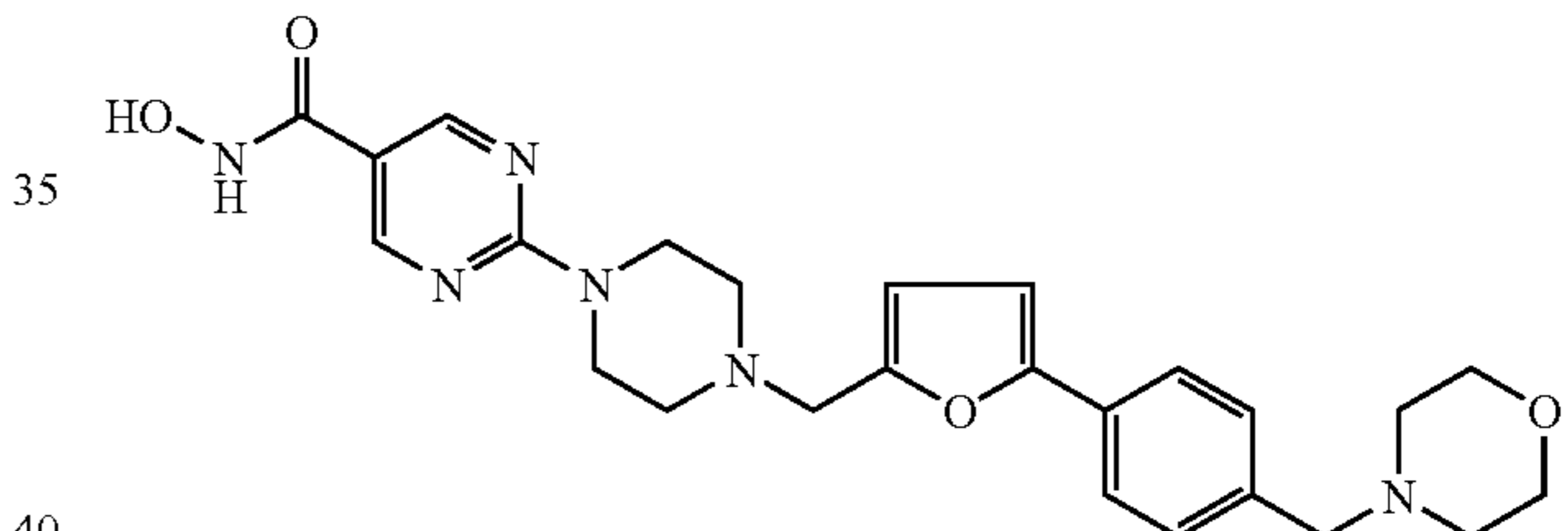
0.47 H_2O •1.99 C_2HF_3O_2 ; Co. No. 9
