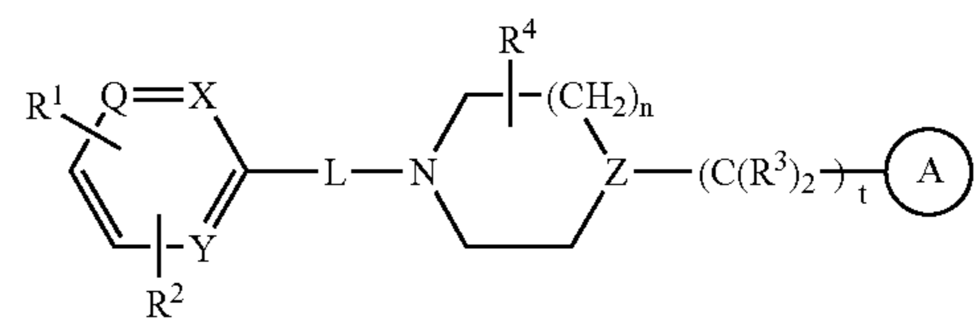
(I-a)
