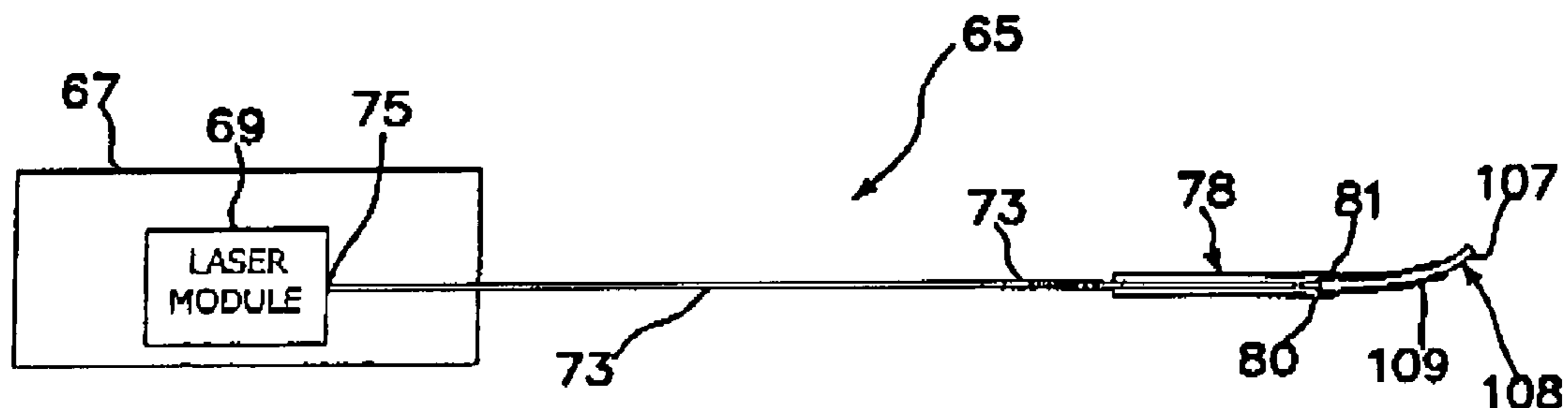
FIG. 3
