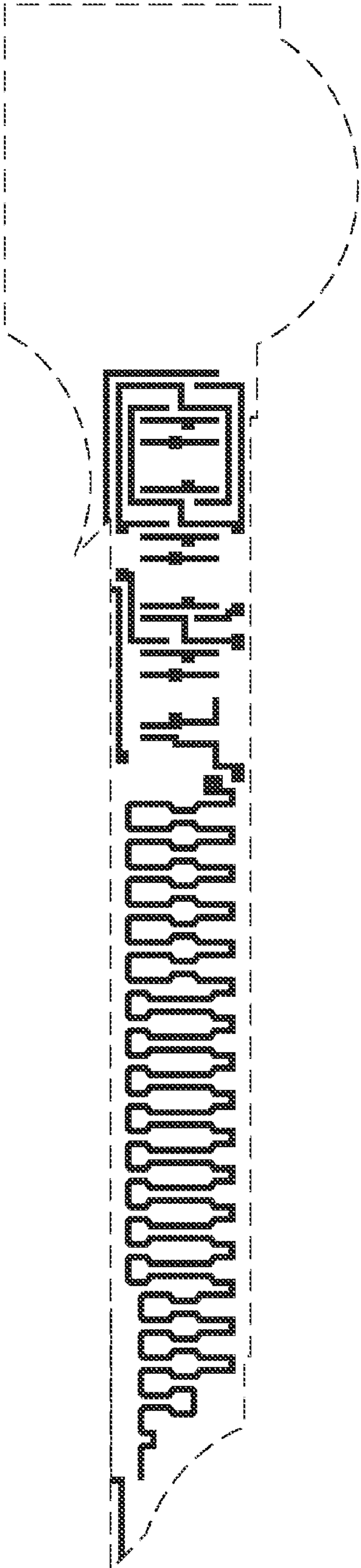
Poly mask
