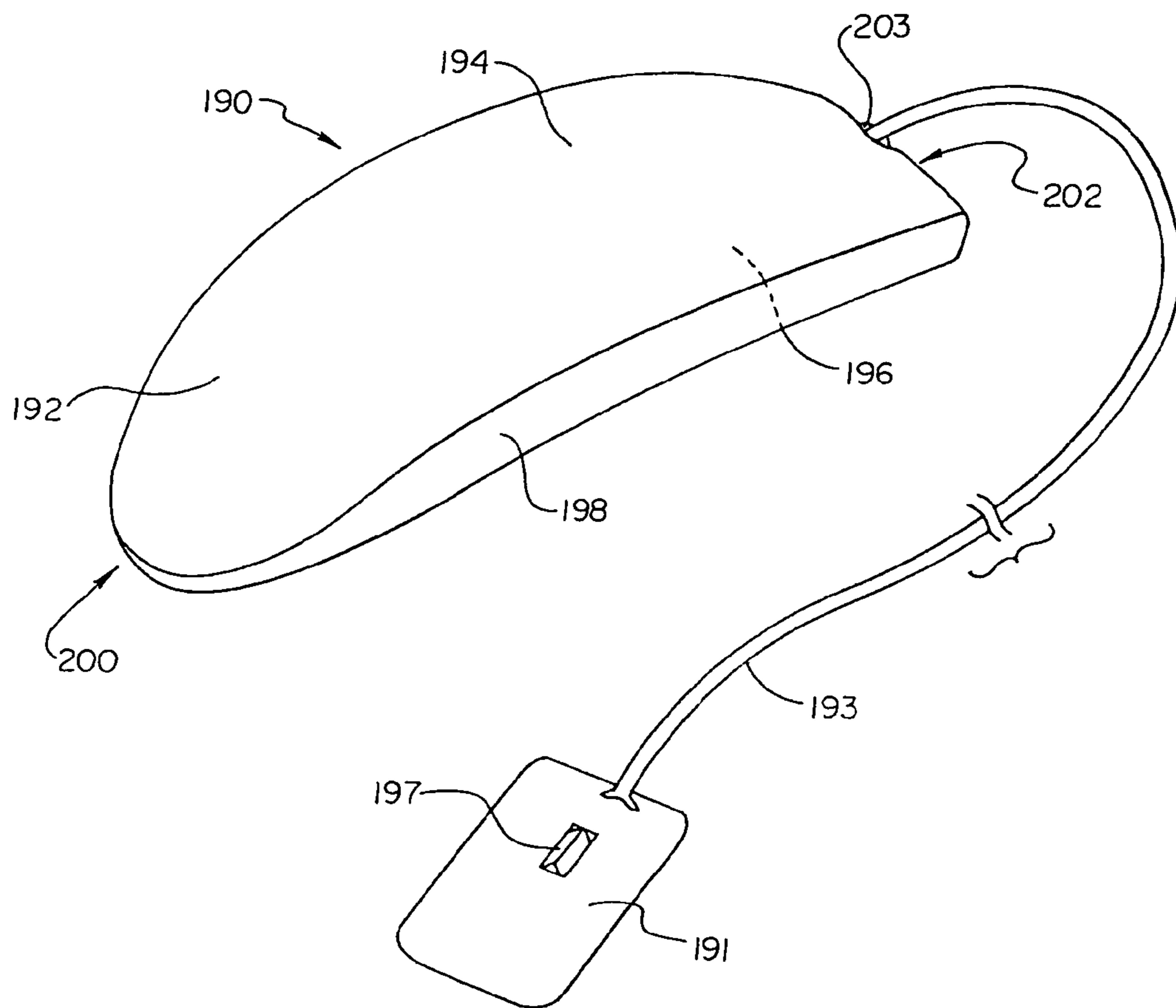
Fig. 19
