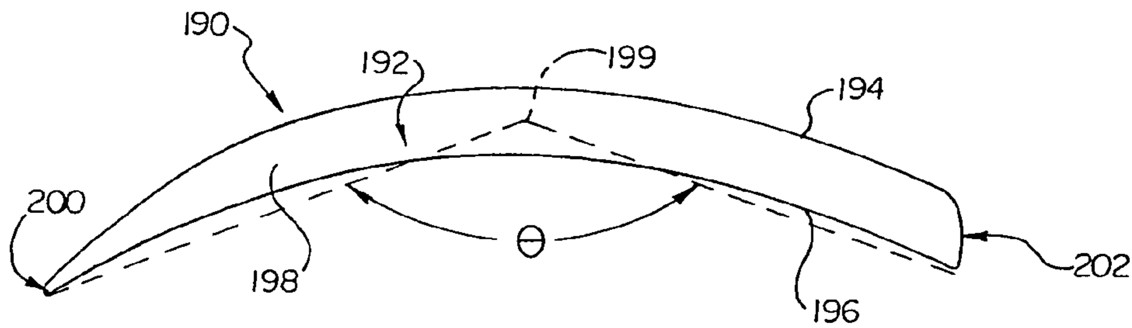
Fig. 21
