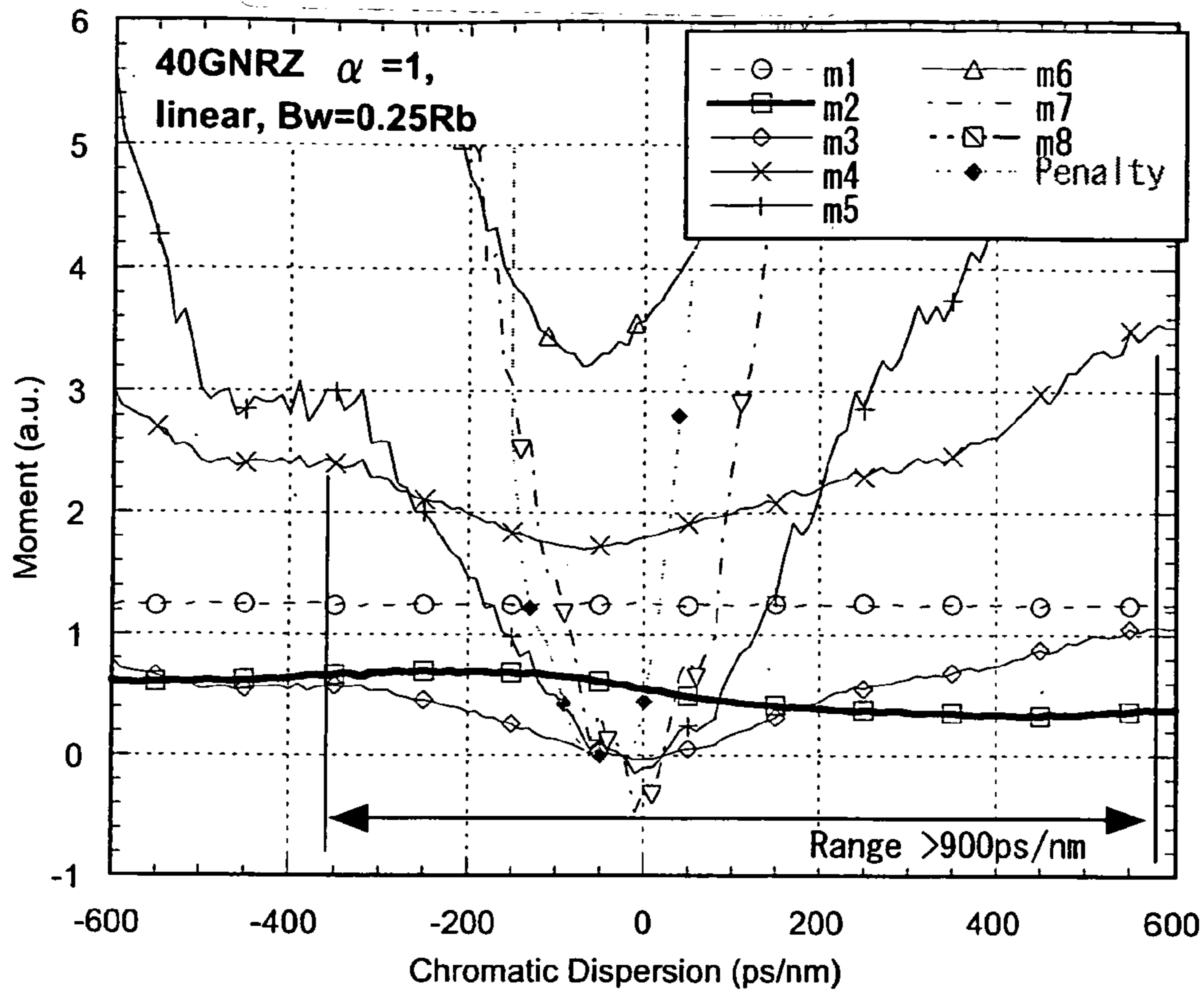
Fig.12 A NRZ
