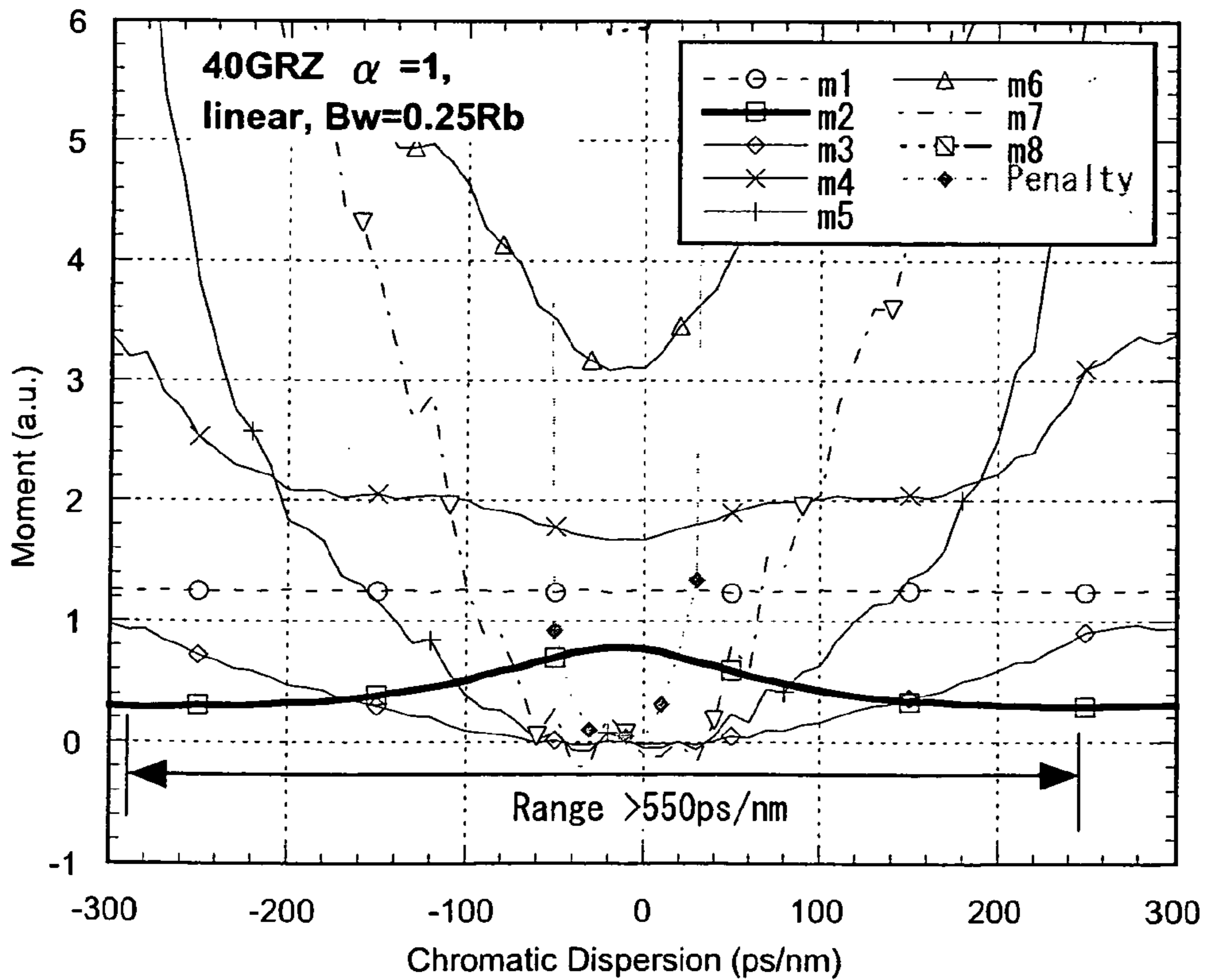
Fig.12 B RZ
