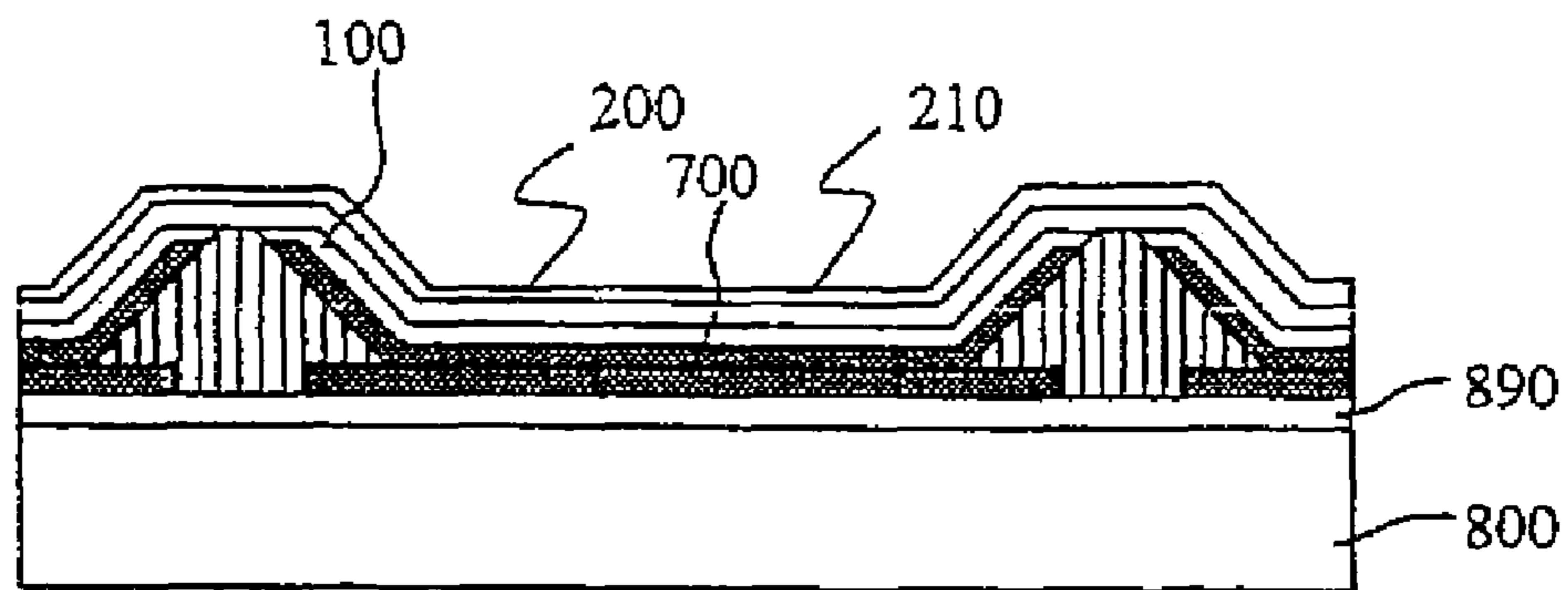
FIG. 25B EXPOSURE
