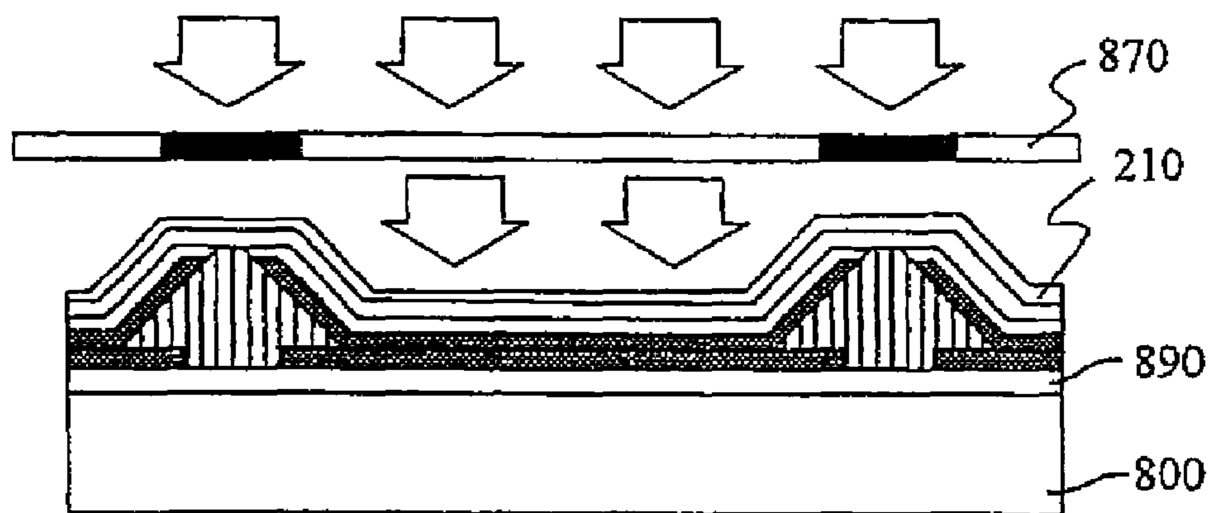
FIG. 25B EXPOSURE
