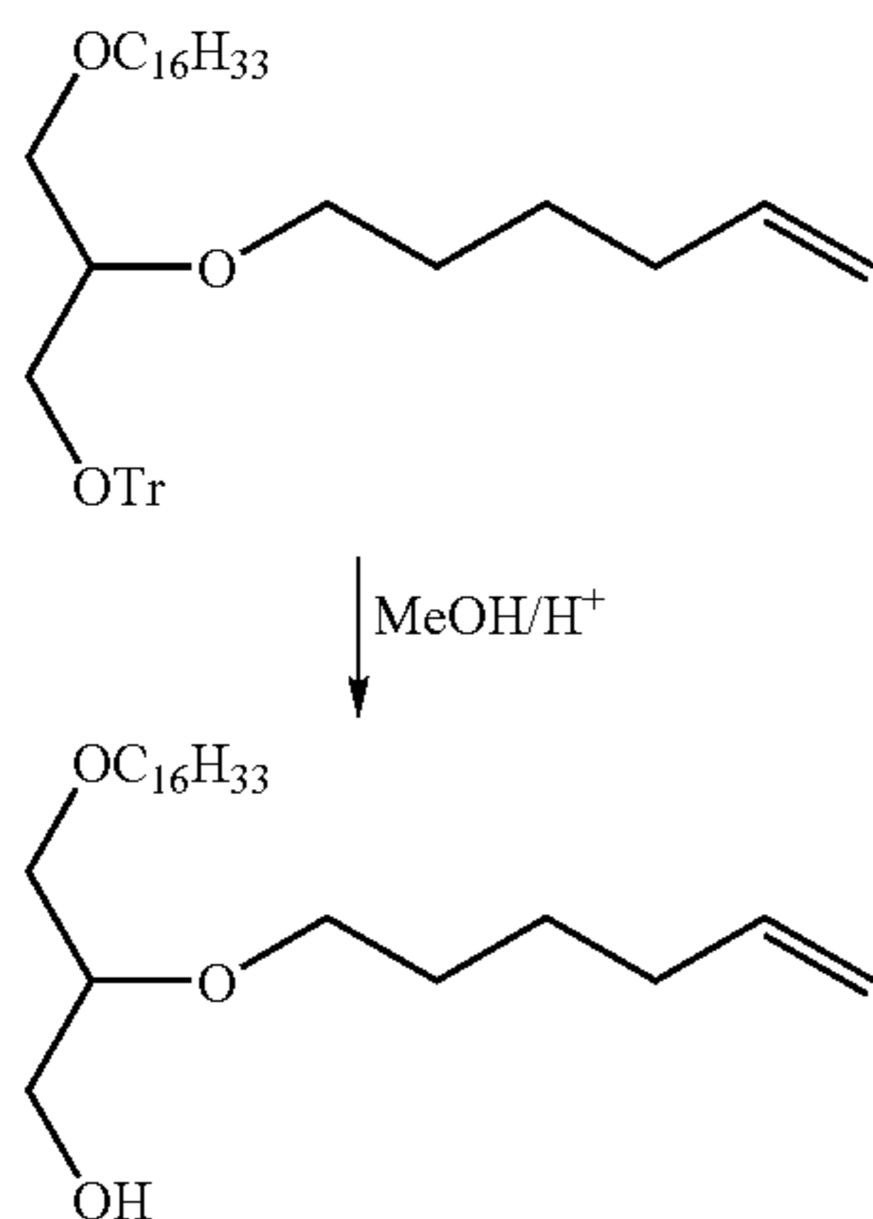
Scheme VI
