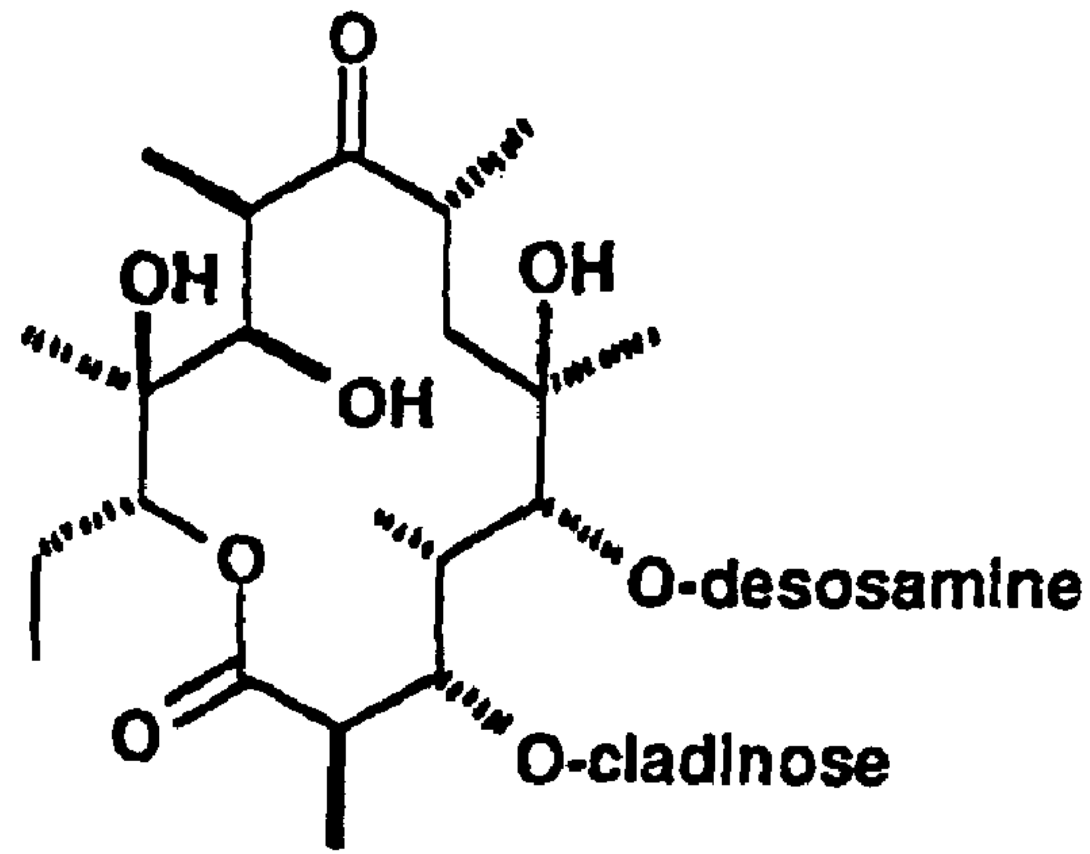
Erythromycin A
