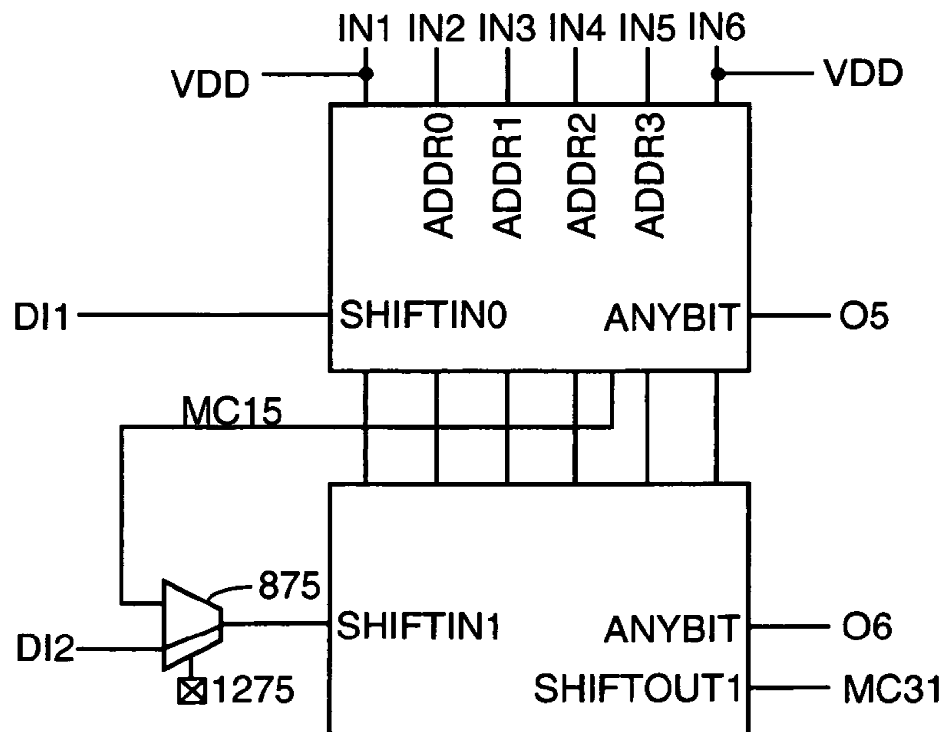
FIG. 13 (16x2 SRL)
