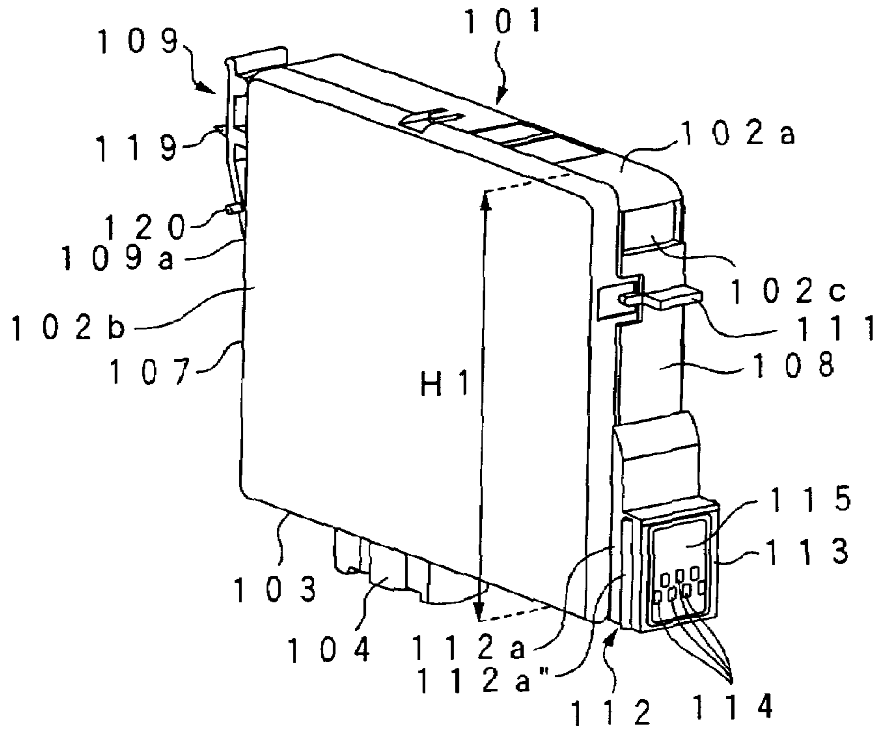
FIG. 14E
