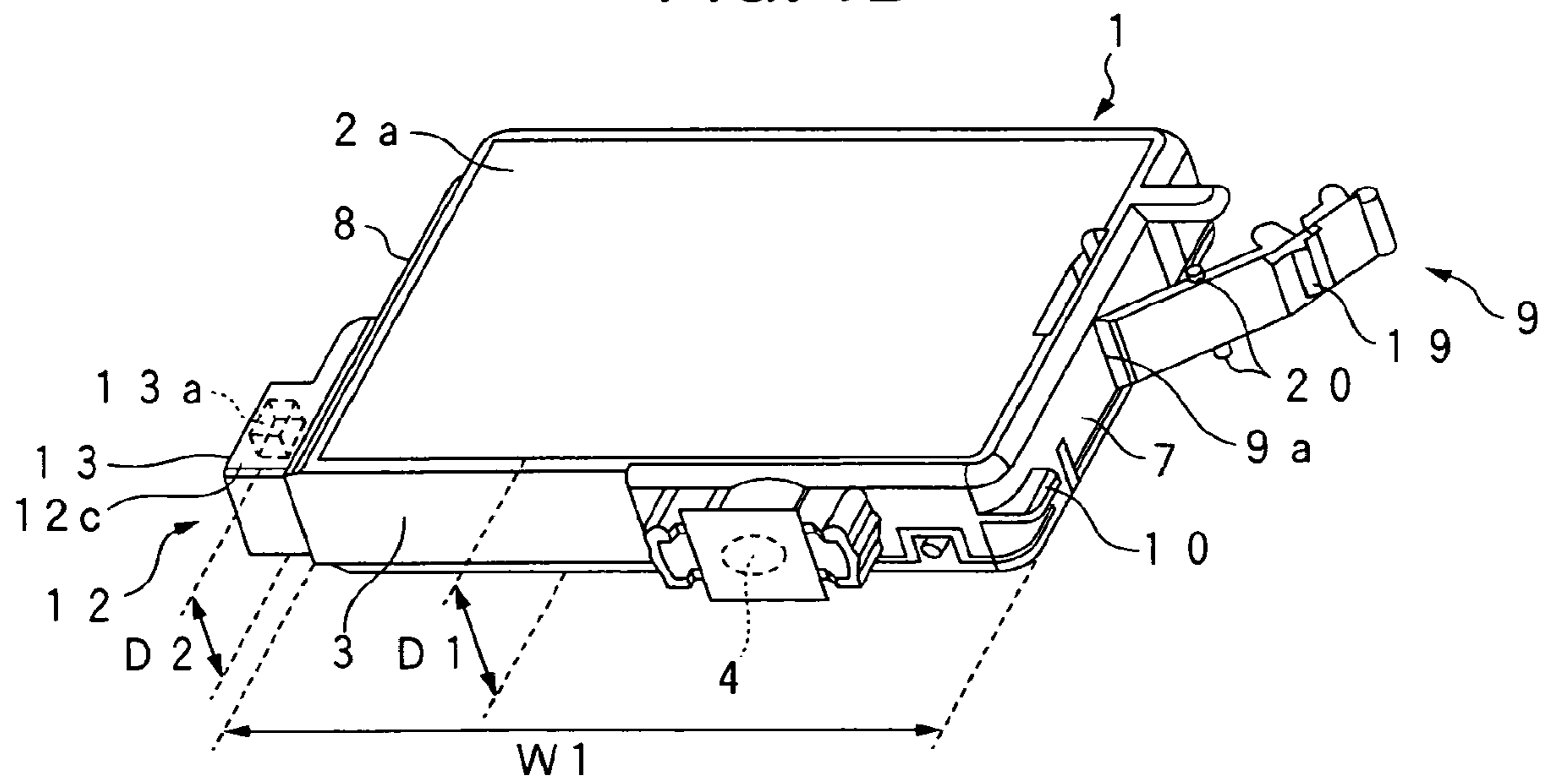
FIG. 1B
