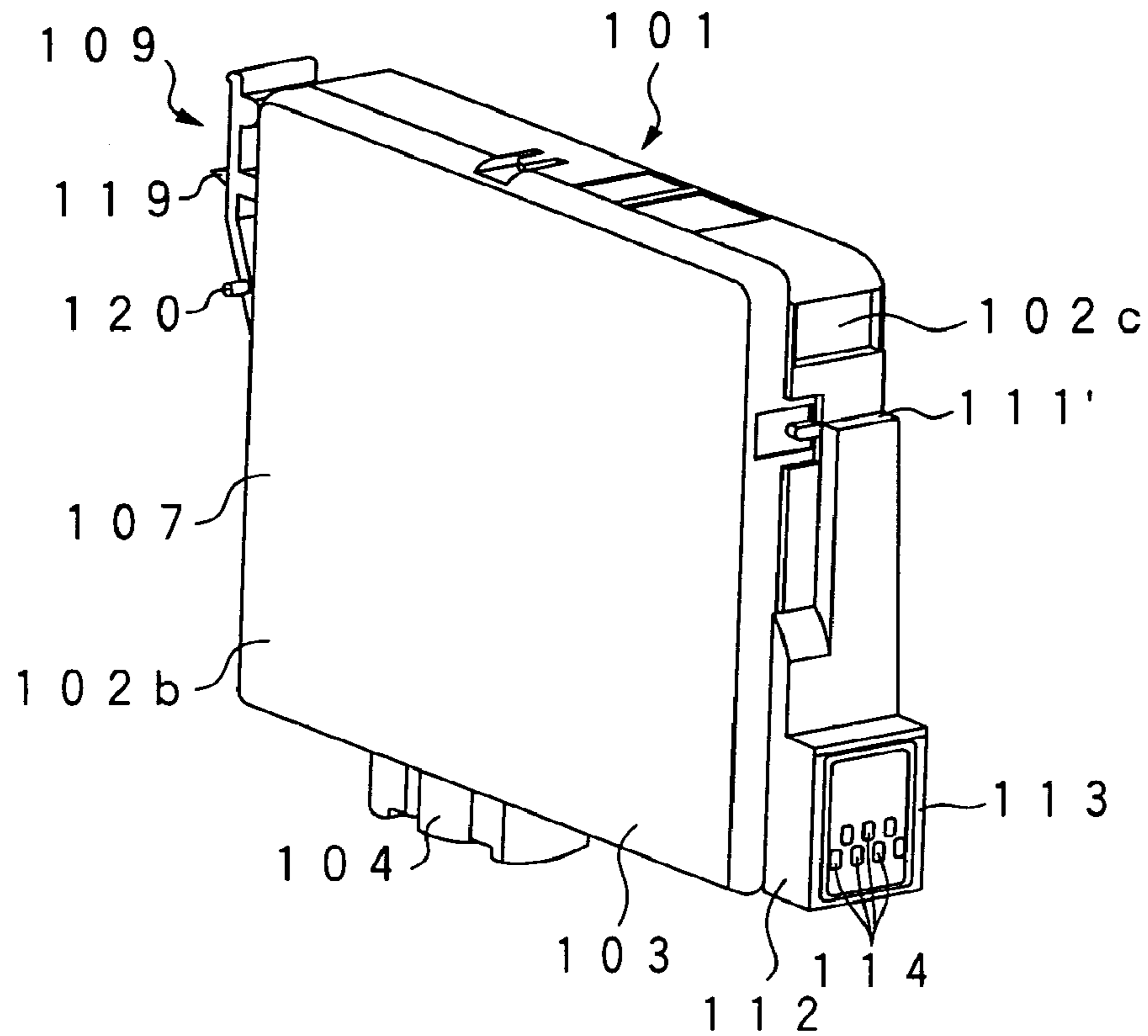
FIG. 21A
