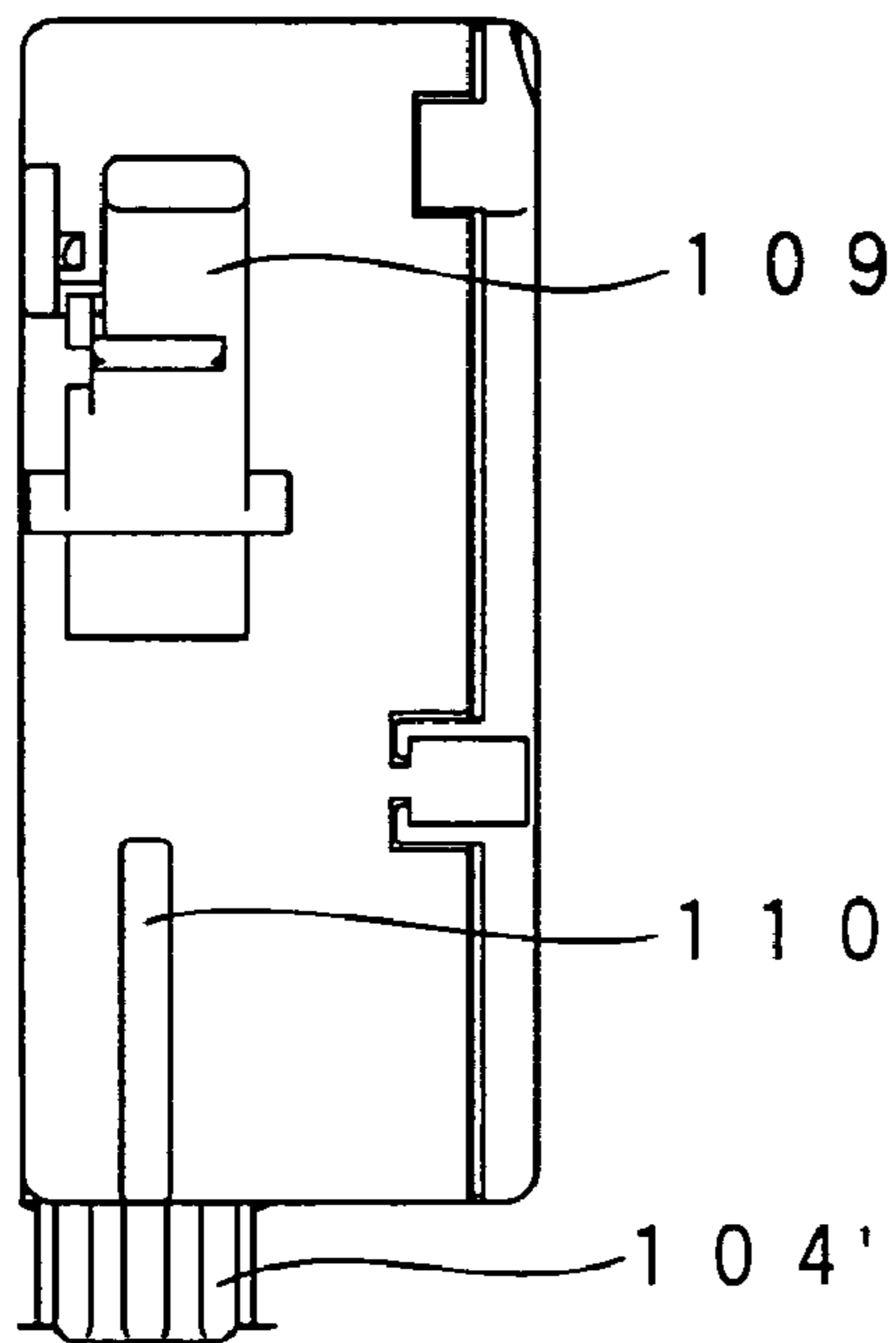
FIG. 25A
