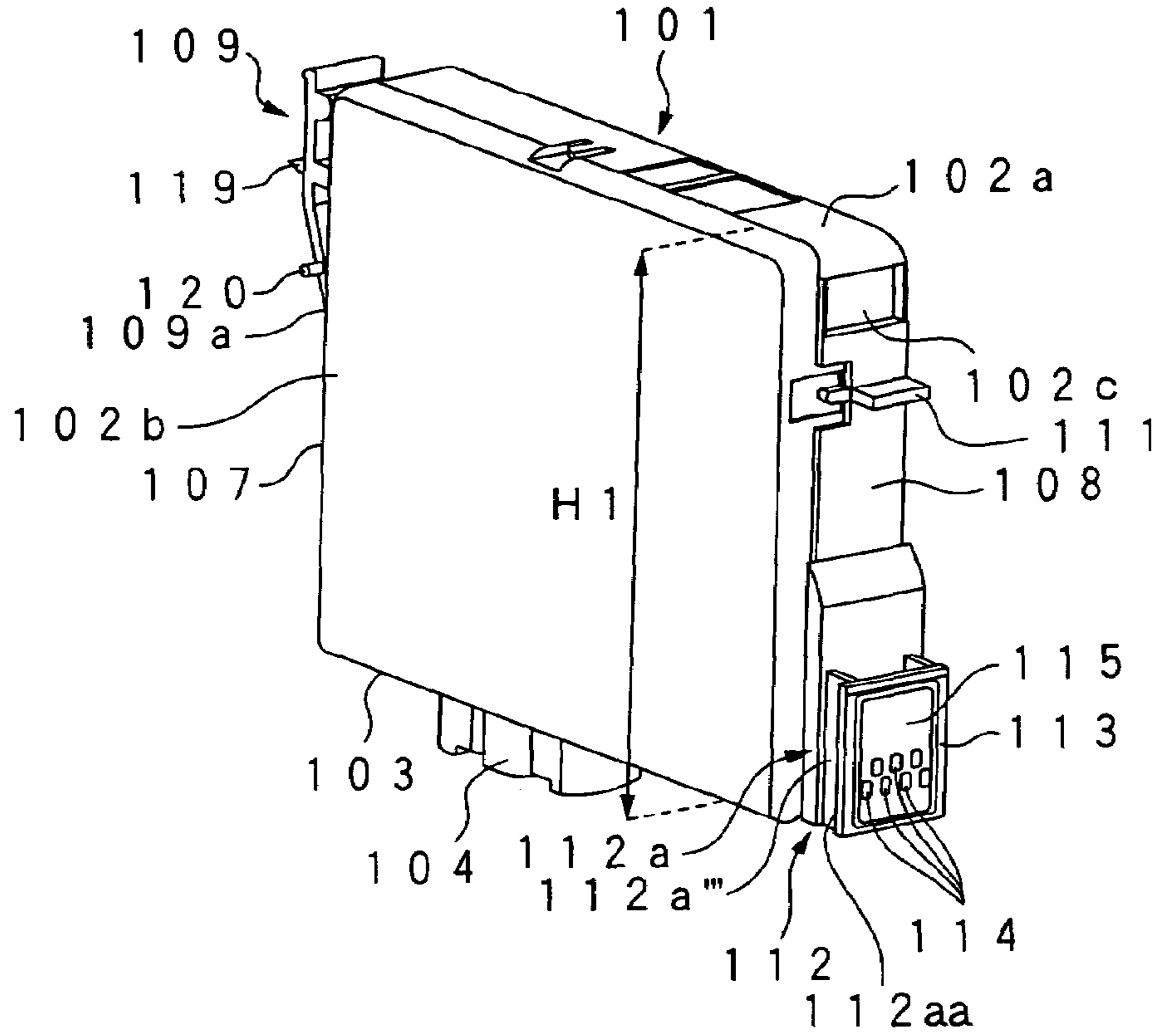
FIG. 14H
