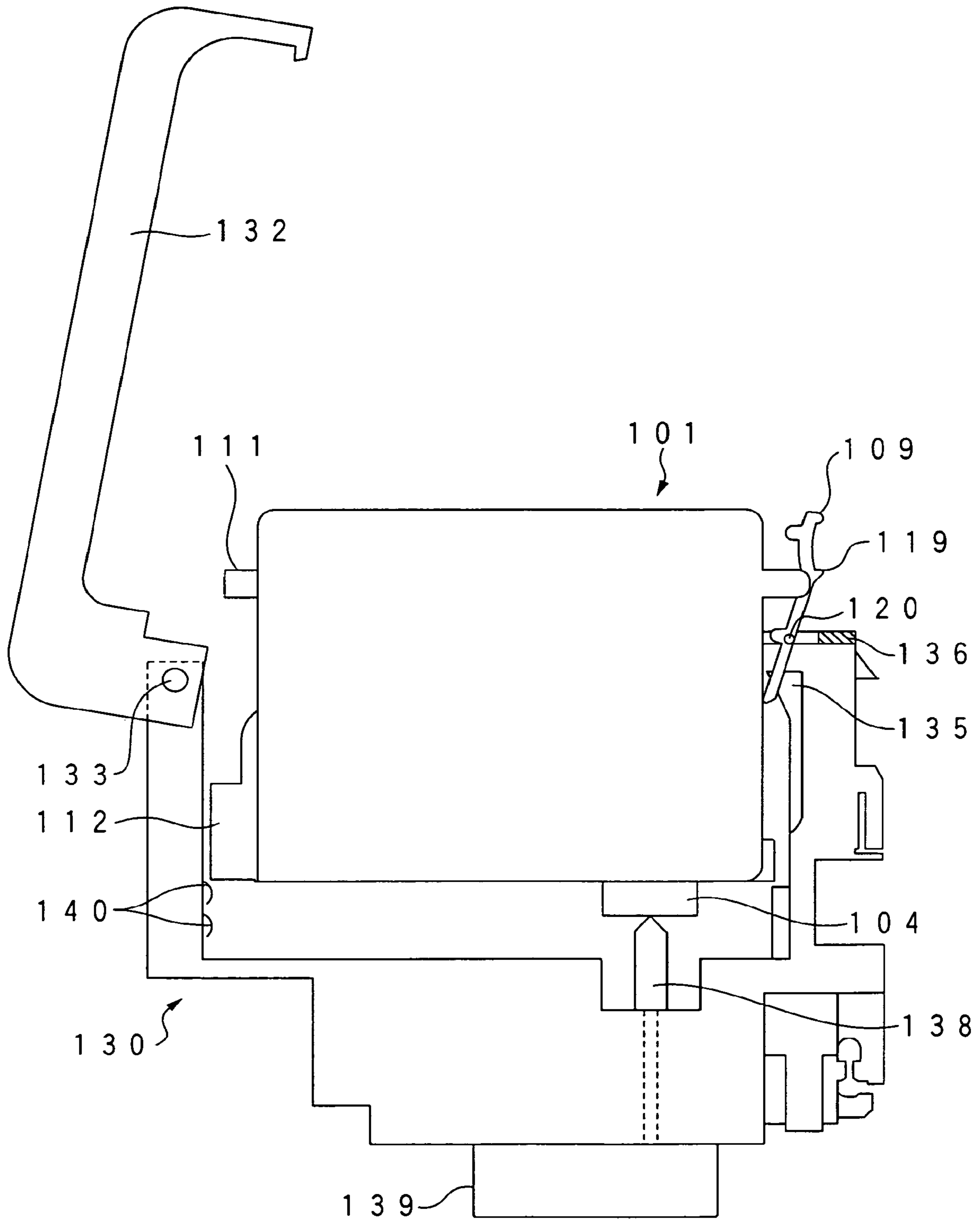
FIG. 18
