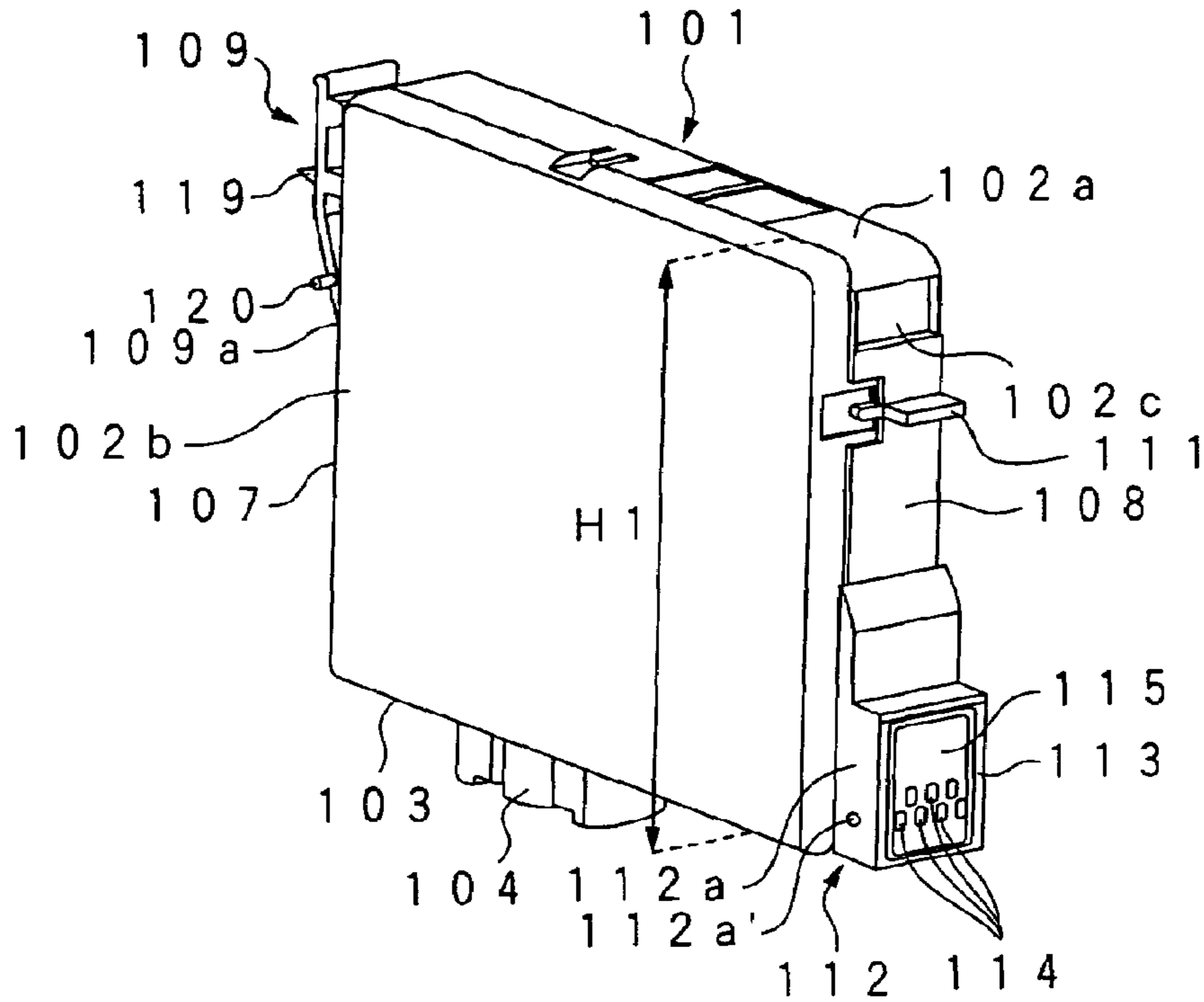
FIG. 14C
