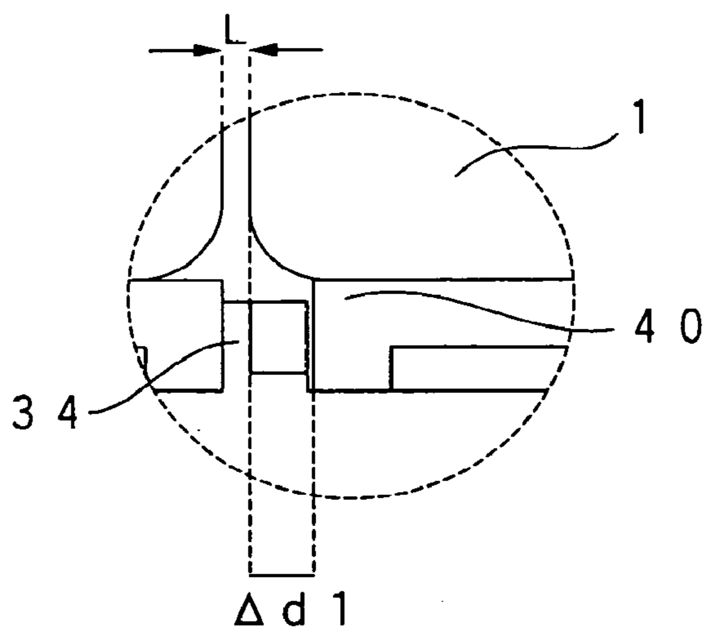
FIG. 6B
