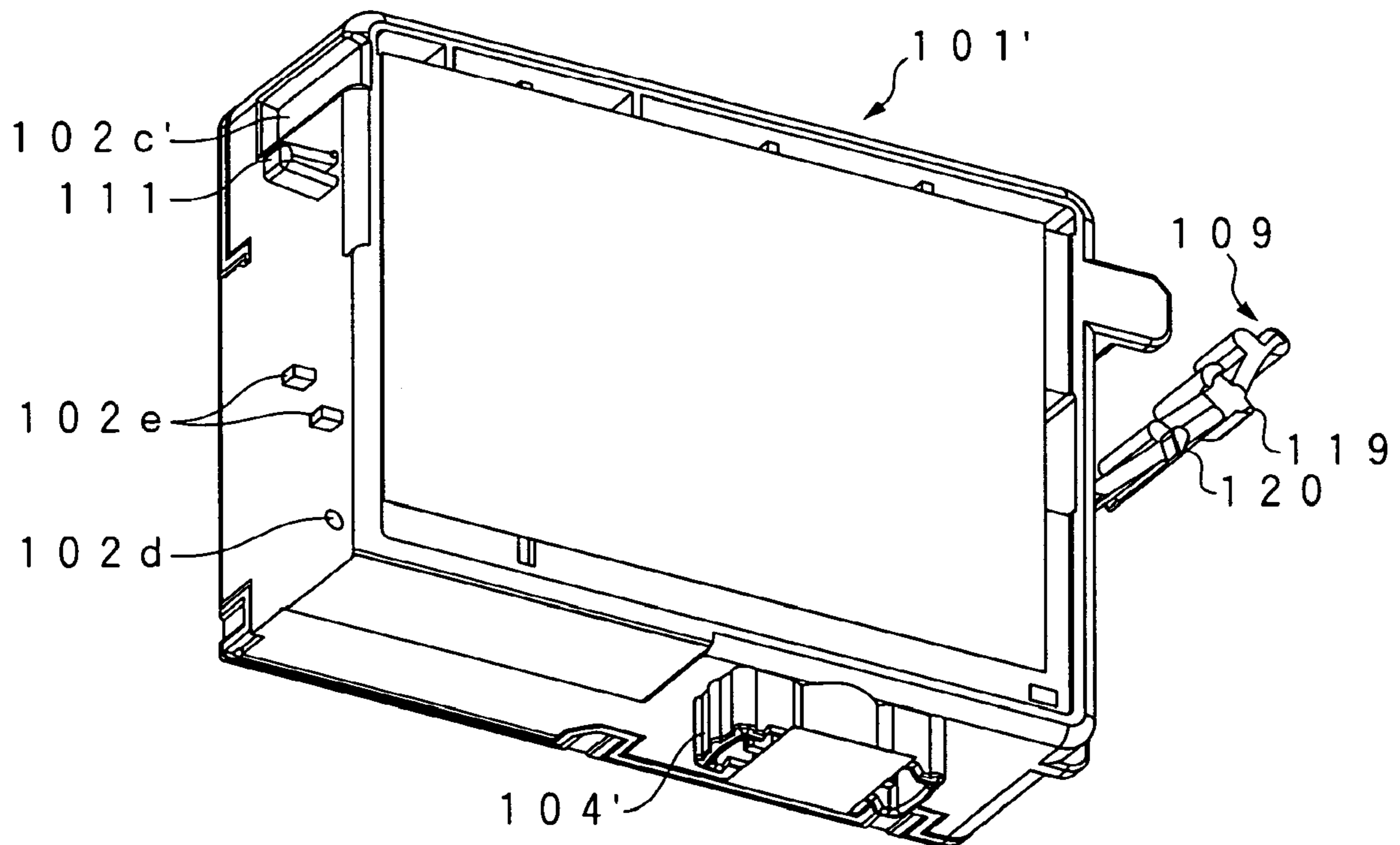
FIG. 29B
