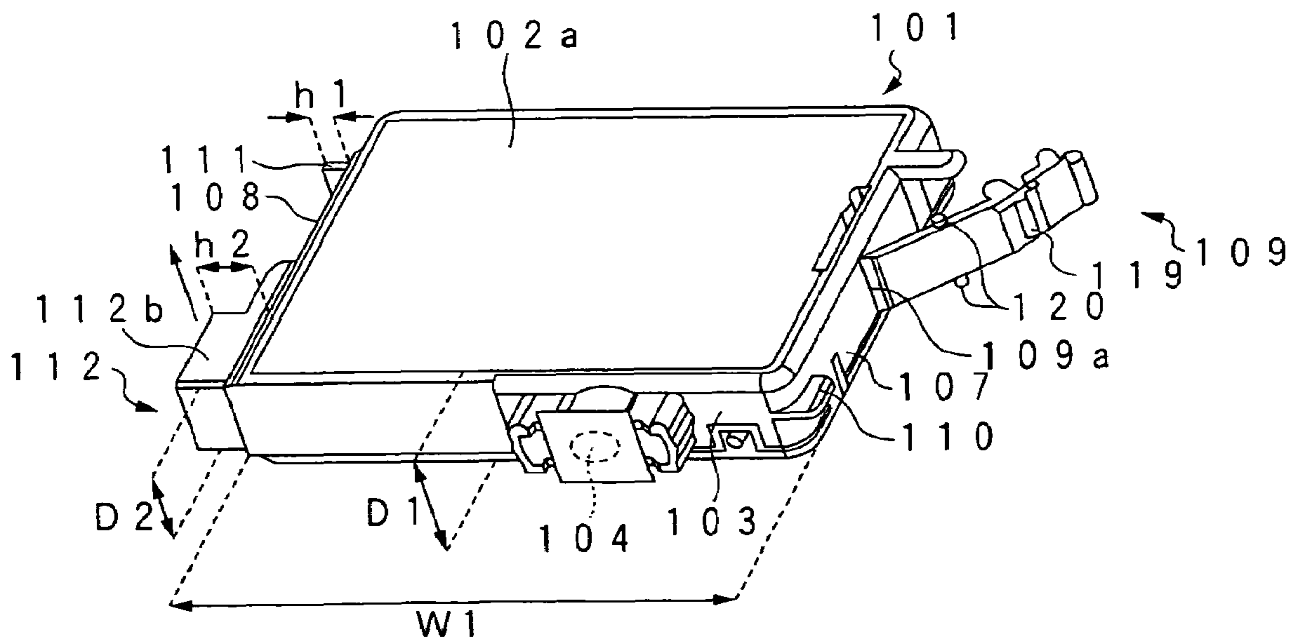
FIG. 14B
