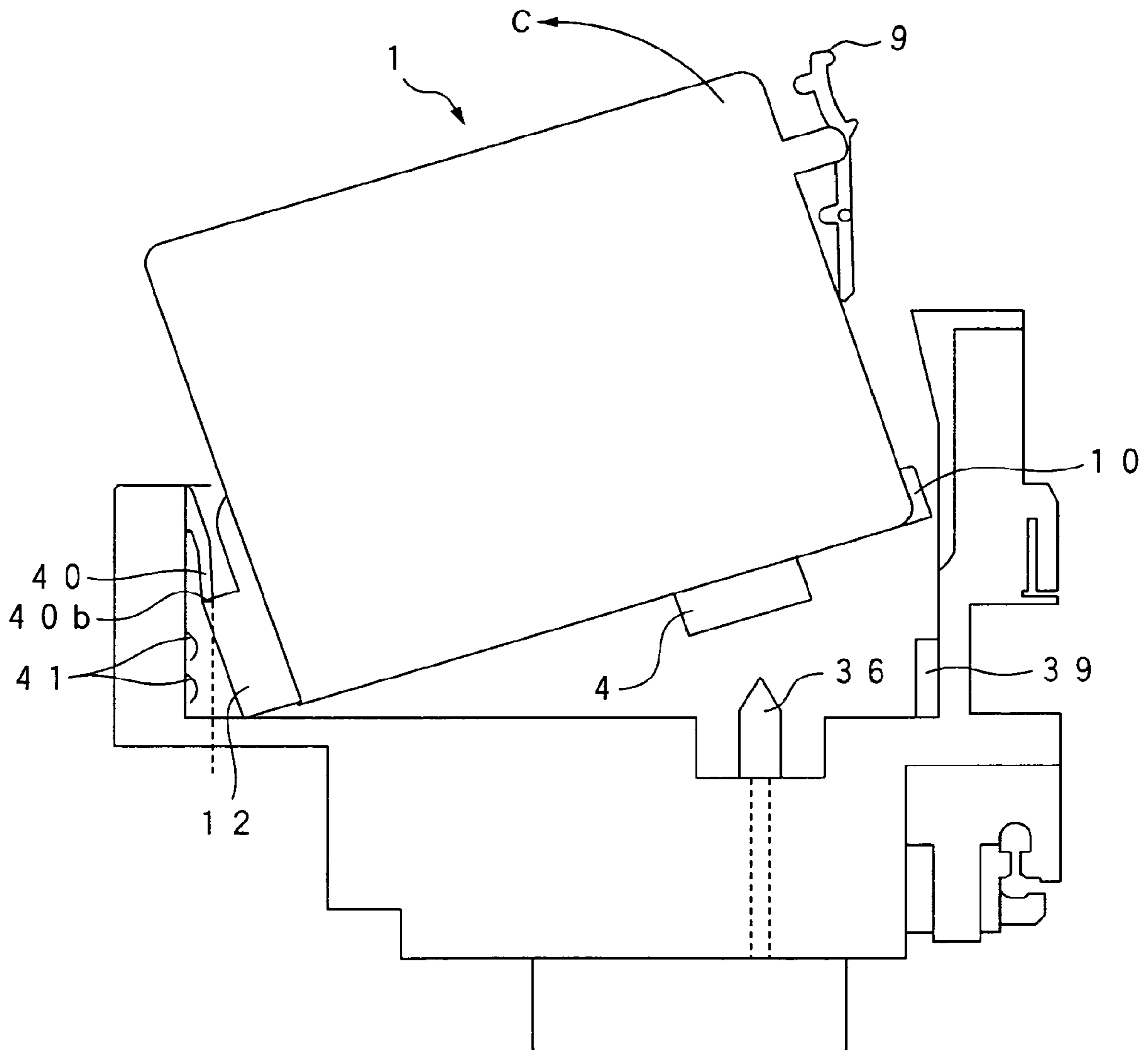
FIG. 11
