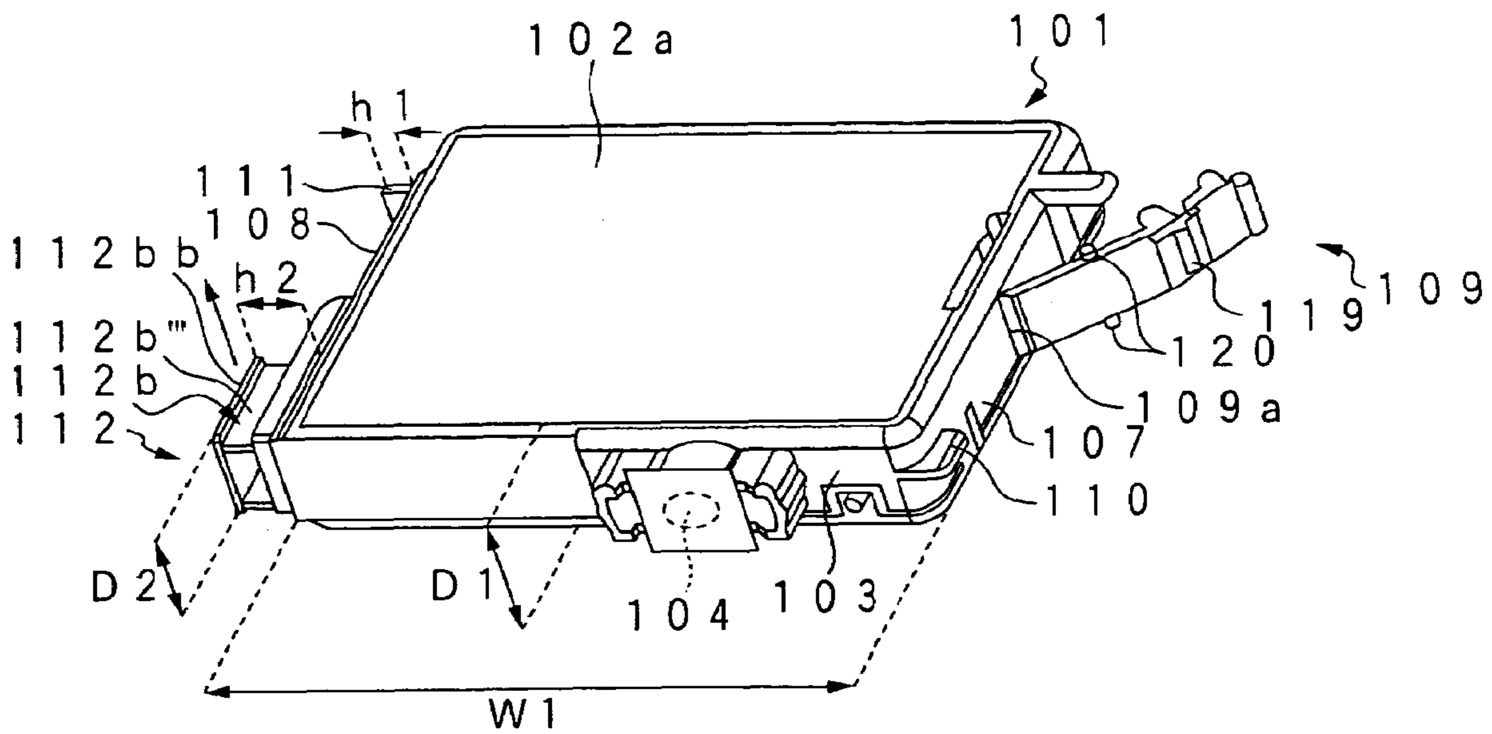
FIG. 14H
