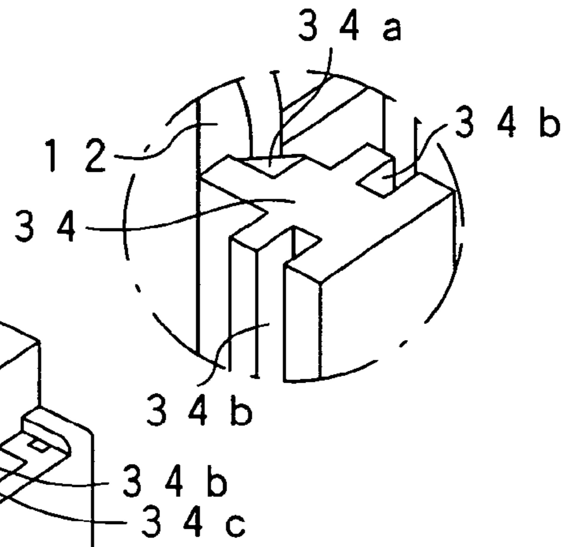
FIG. 7B
