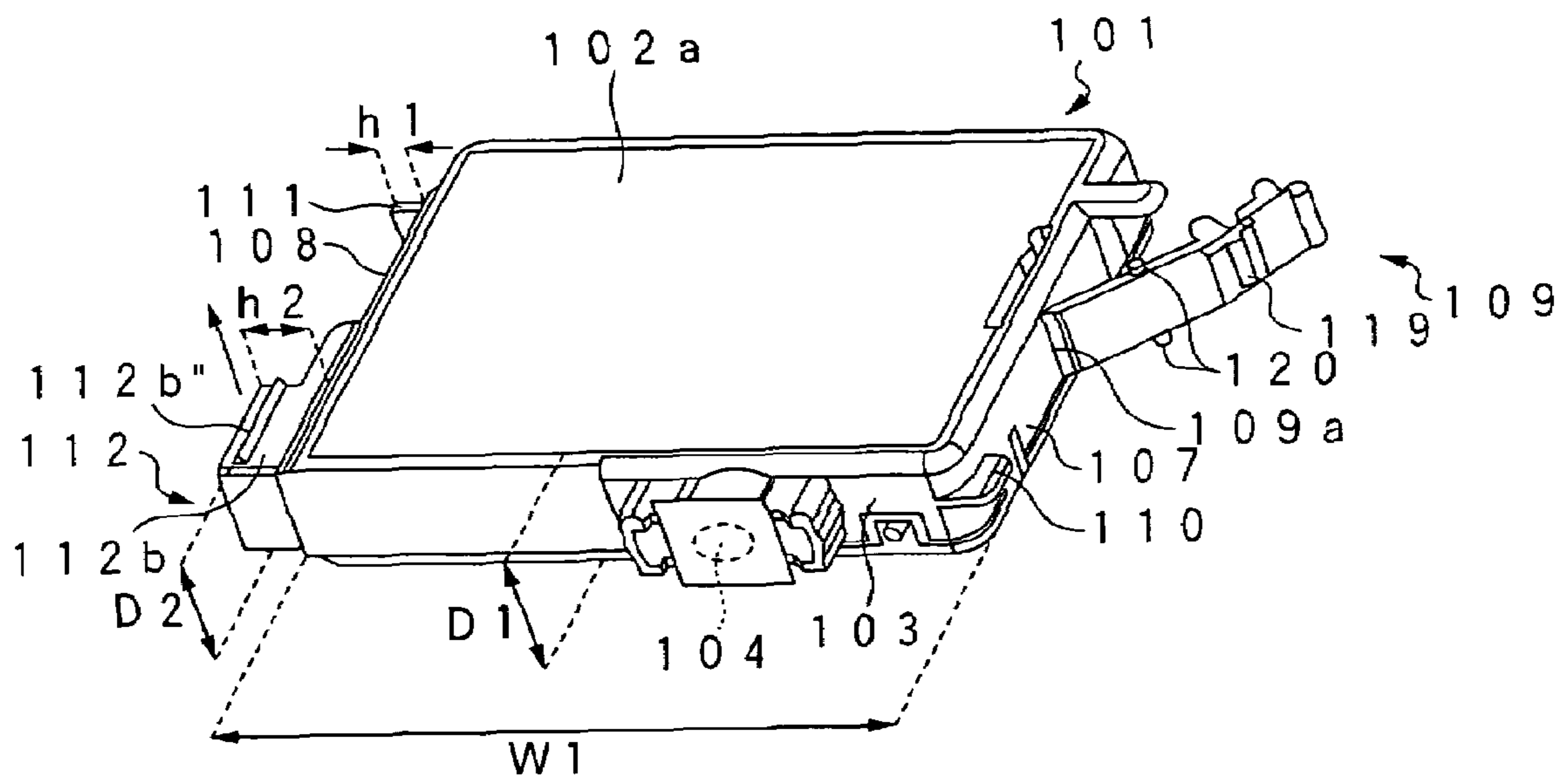
FIG. 14F
