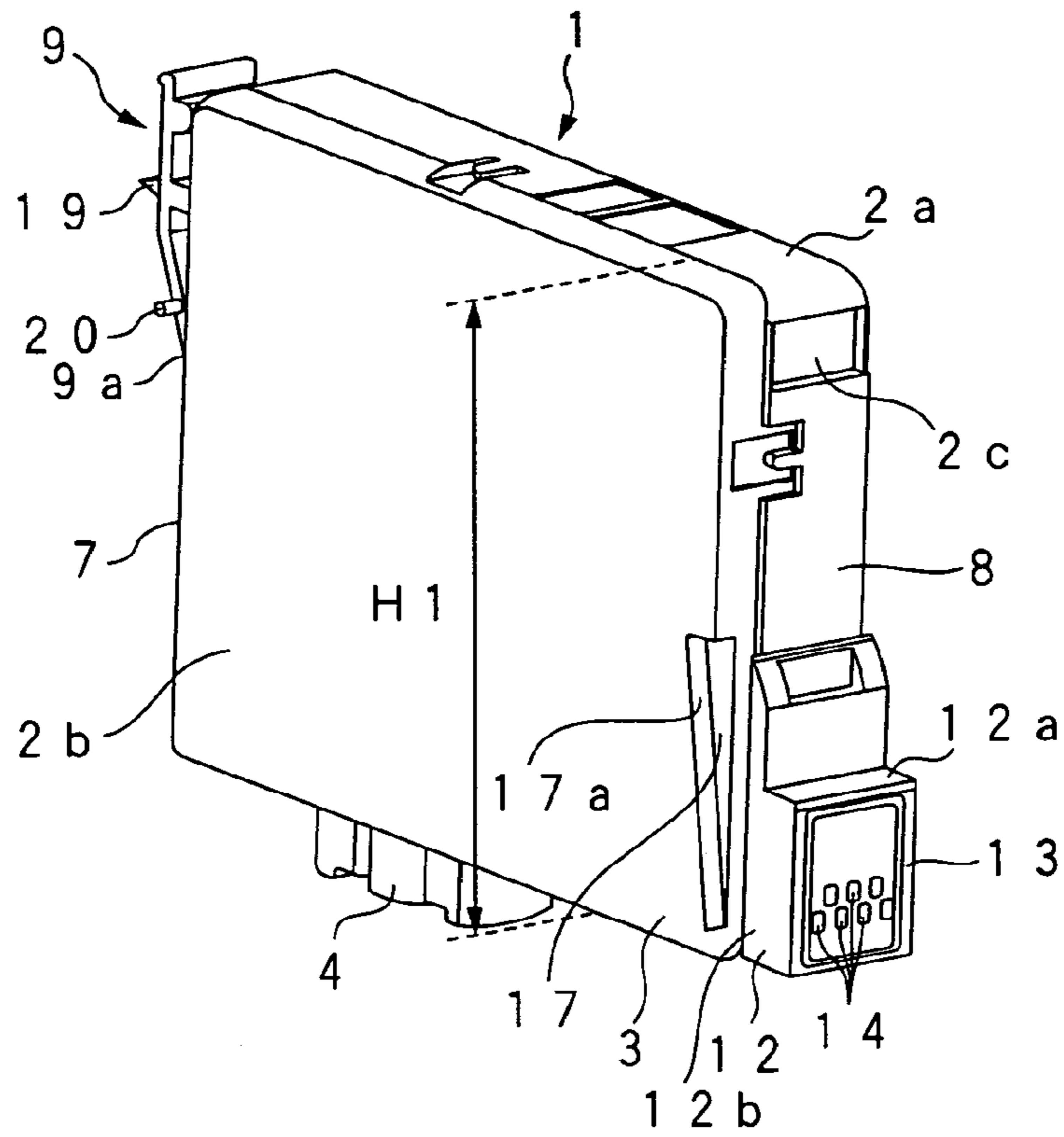
FIG. 1B
