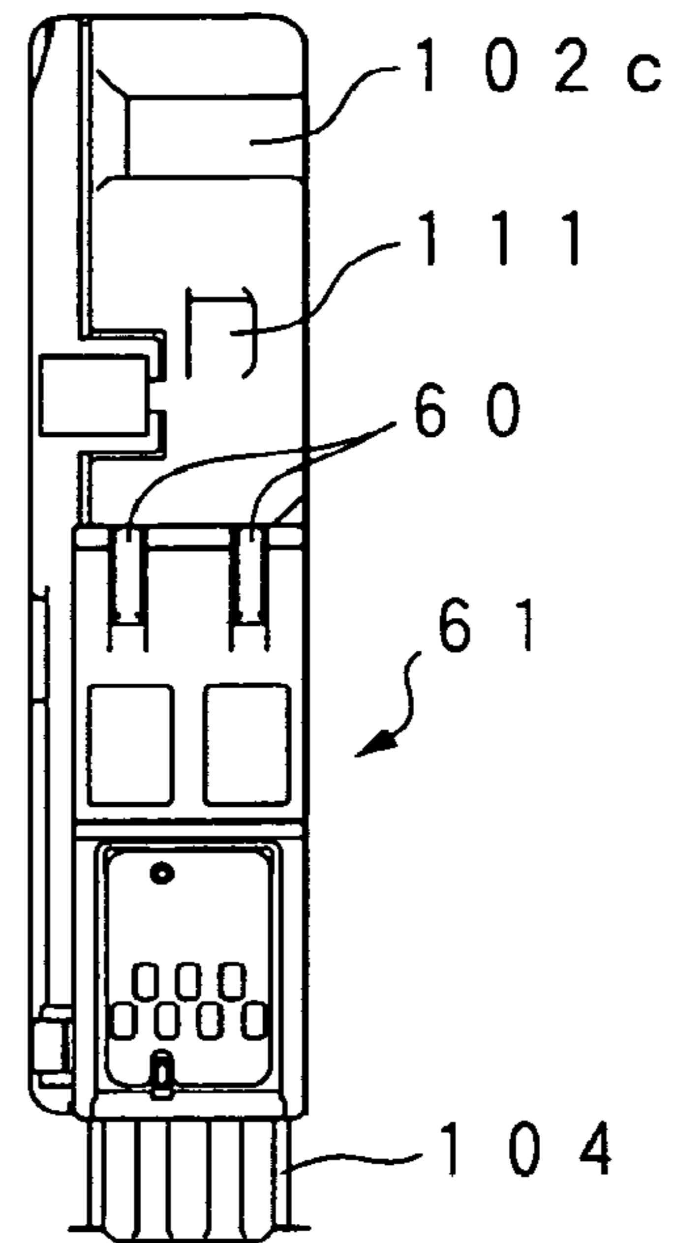
FIG. 23B
