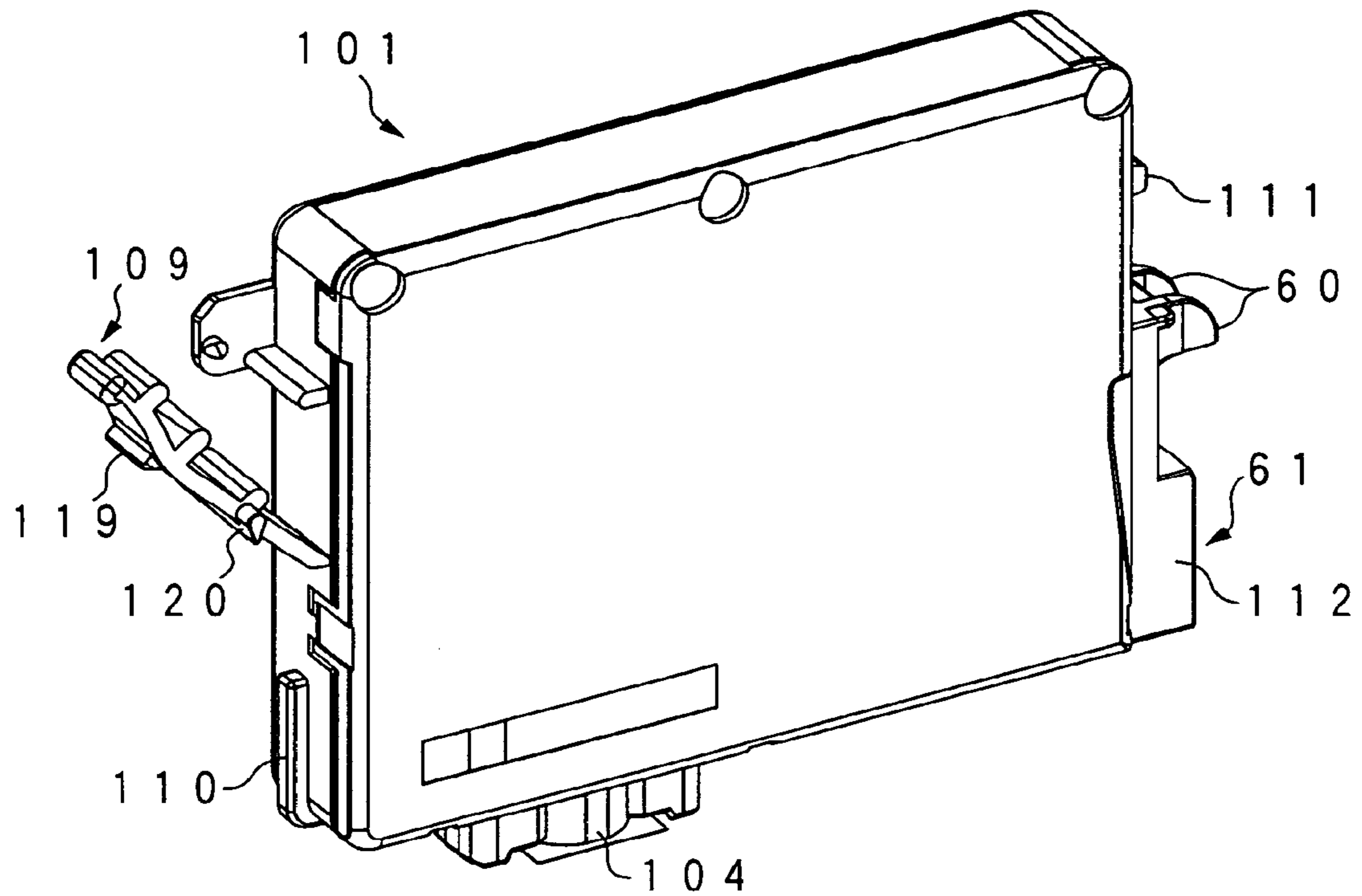
FIG. 22A
