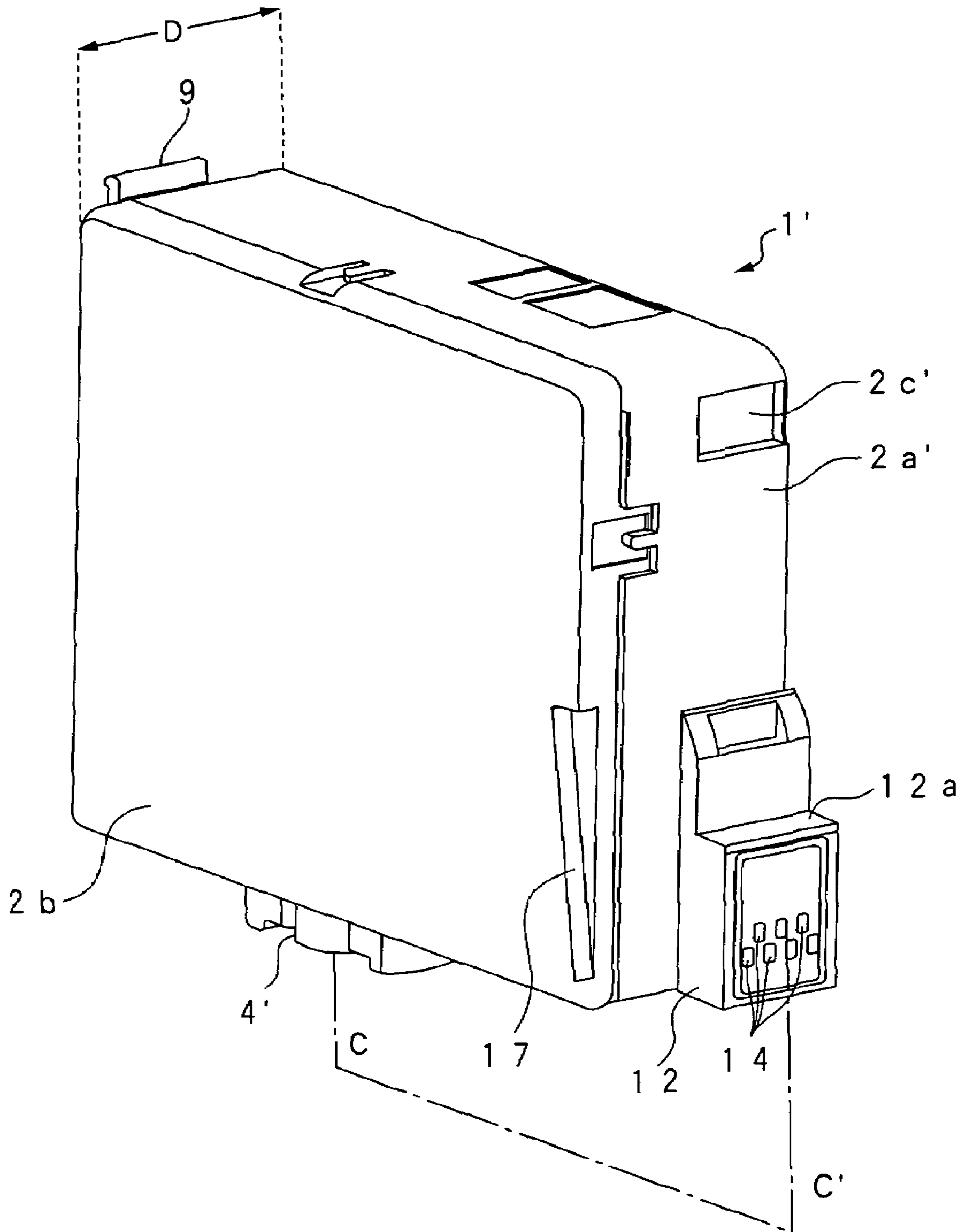
FIG. 13
