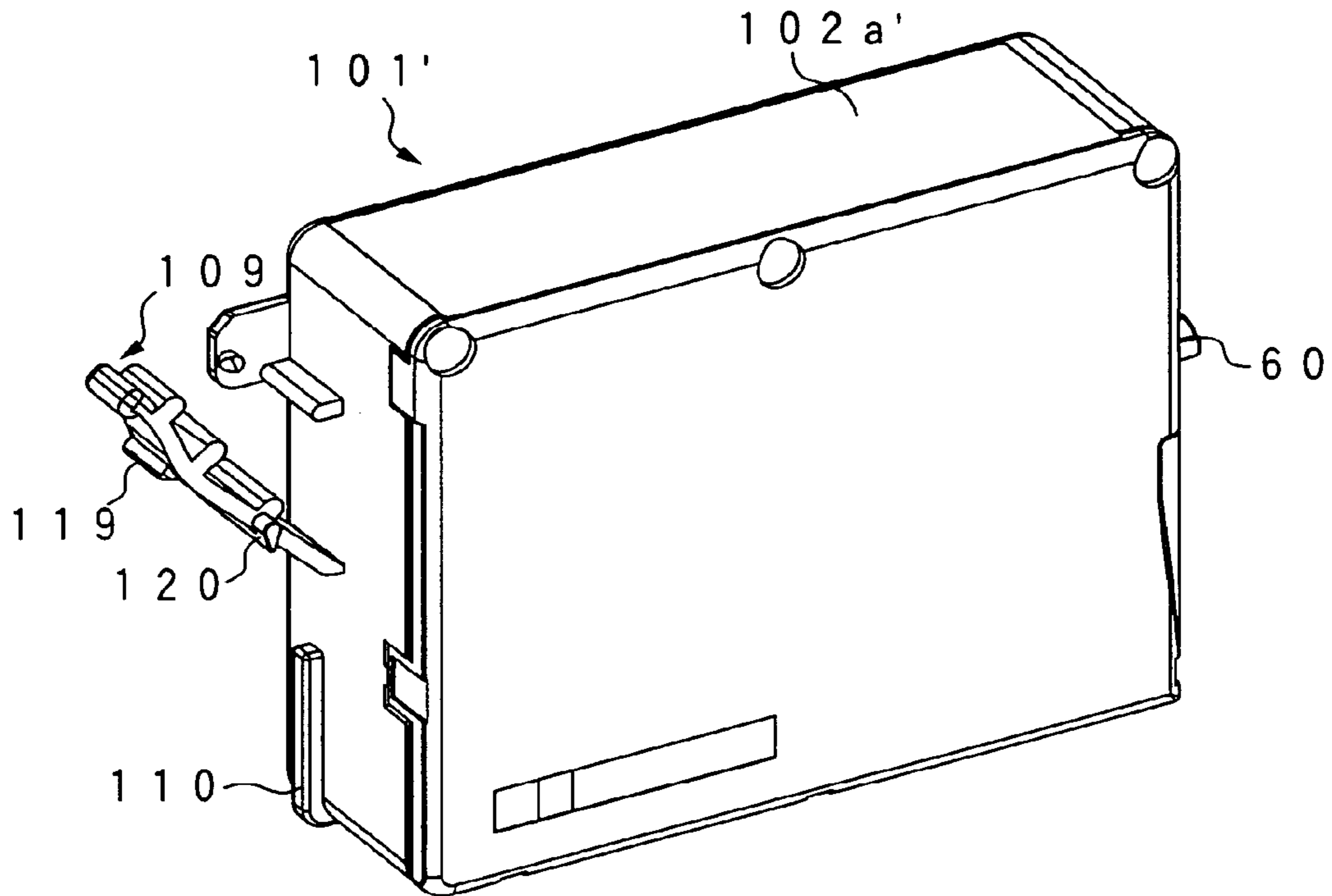
FIG. 24A
