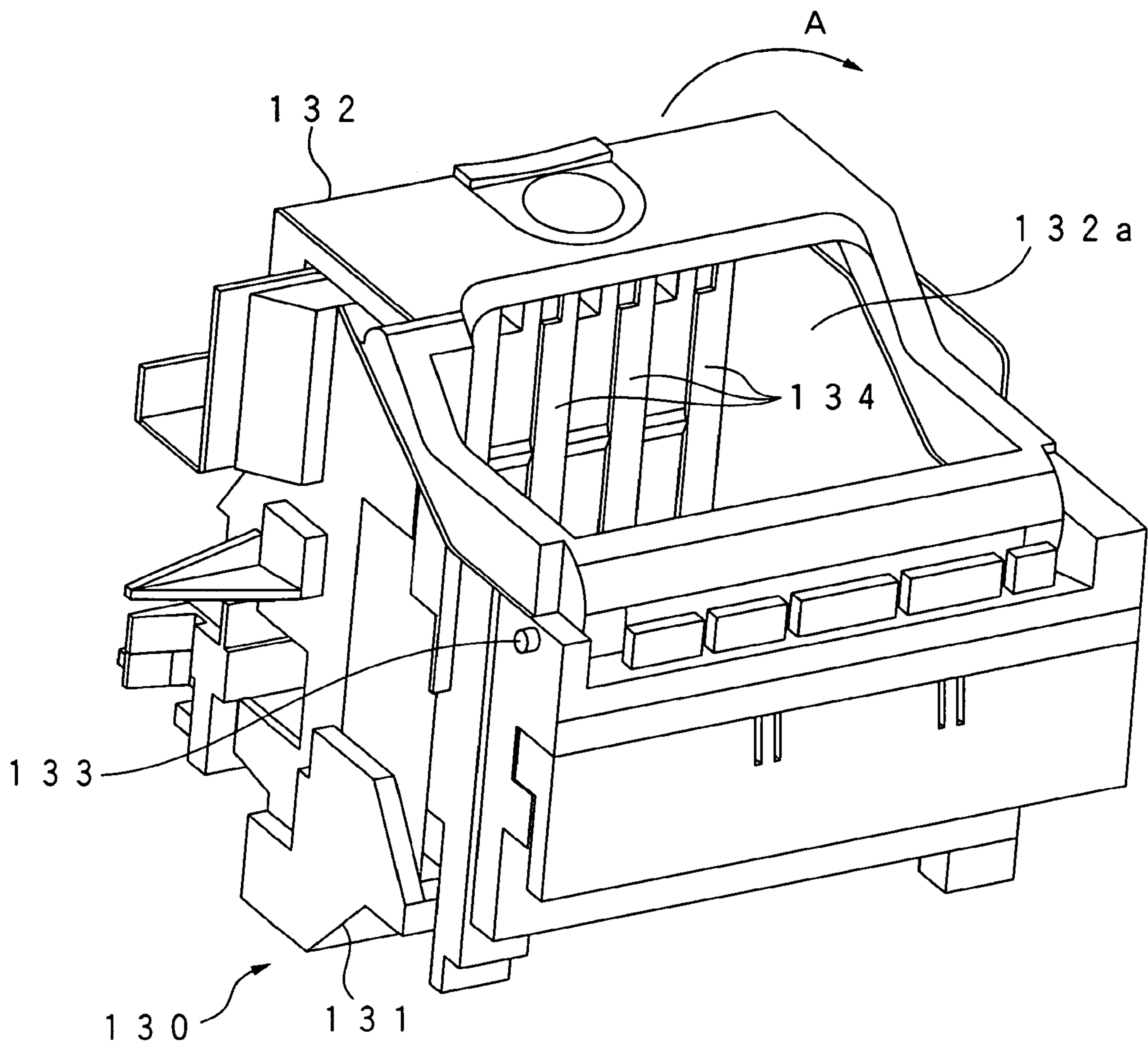
FIG. 15
