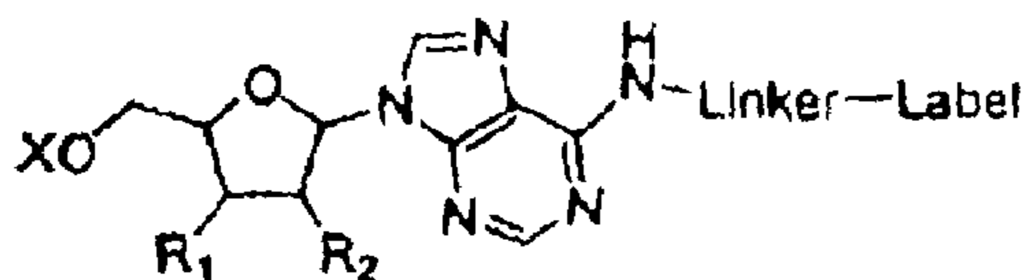
Adenosine N6-linker
