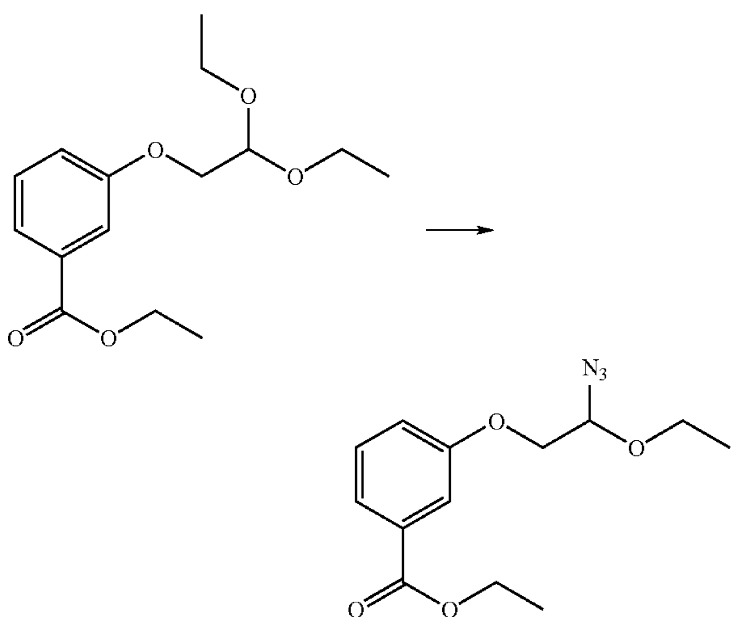
3-(2-Azido-2-ethoxy-ethoxy)-benzoic acid ethyl ester
