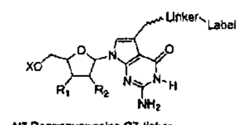
N7 Deazaguanosine C7-linker
