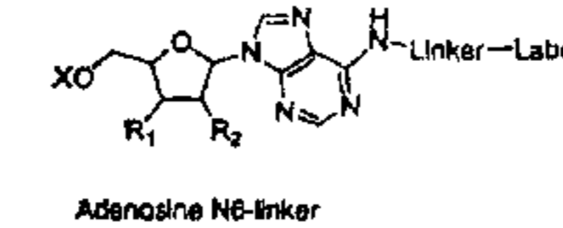
Adenosine N6-linker
