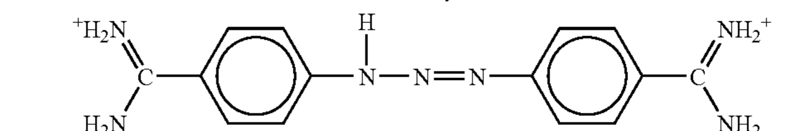
Berenil
