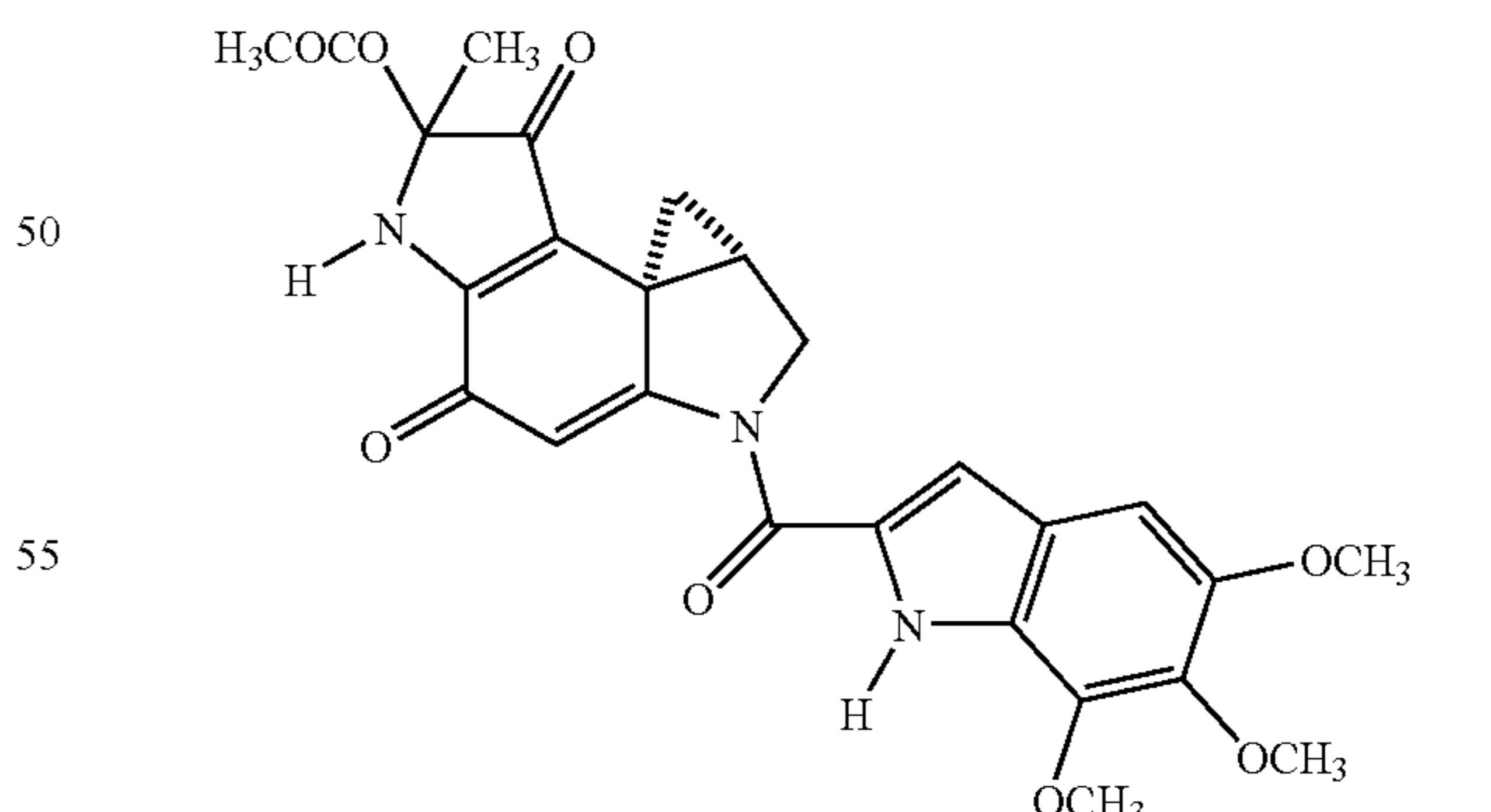
Duocarmycin SA
