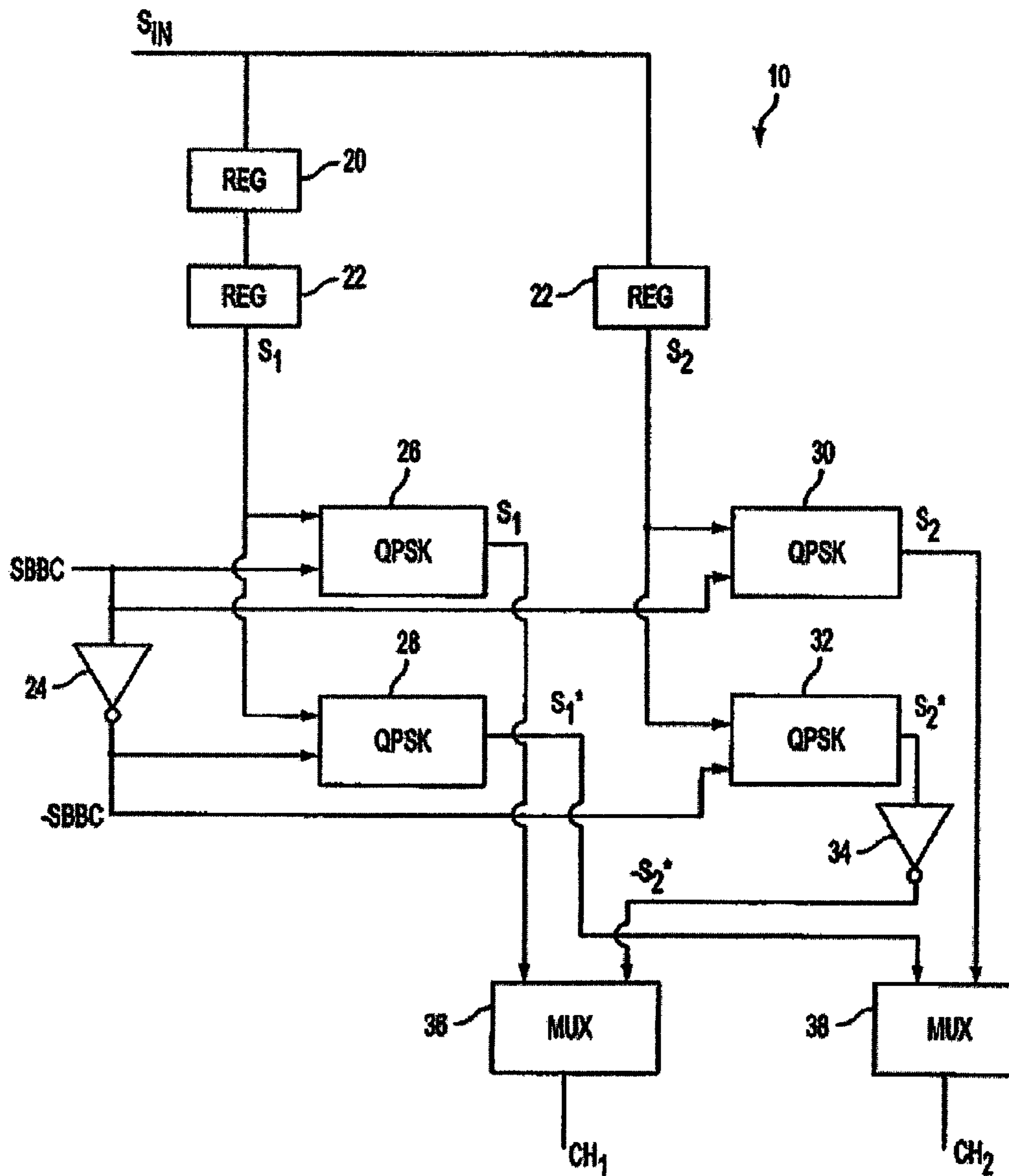
FIG. 3 (PRIORART)
