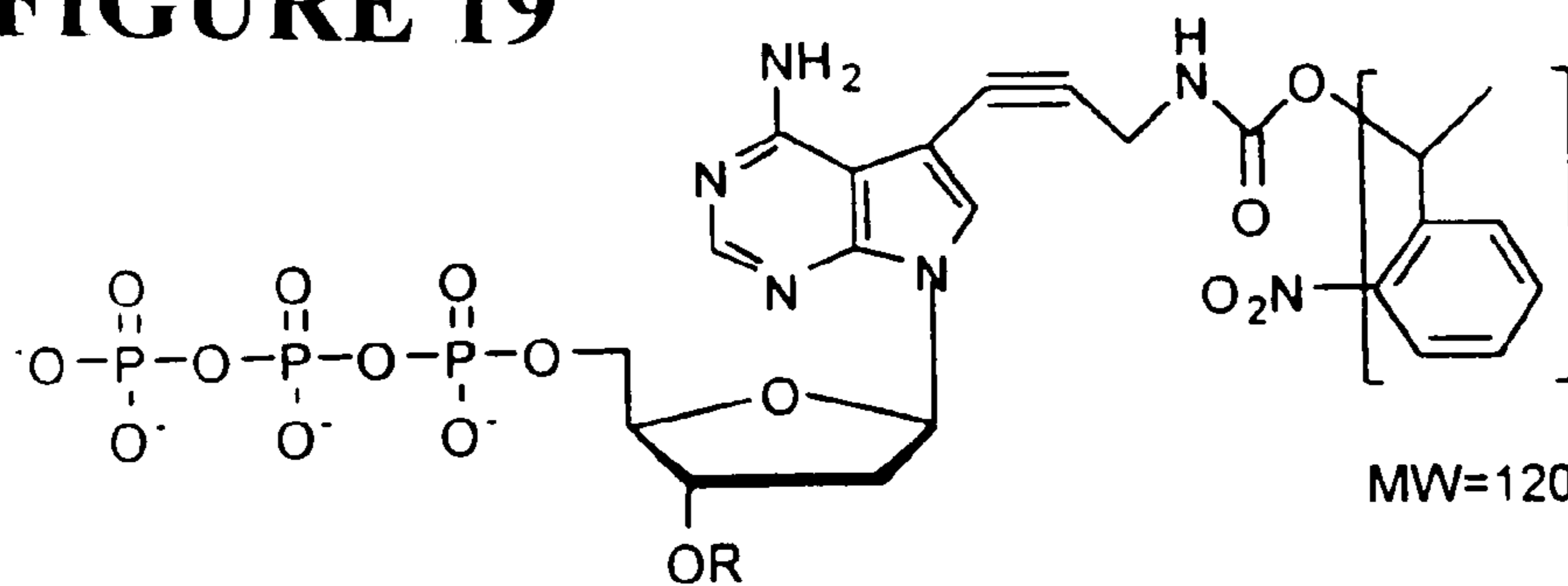
(Nitro-Benzyl)-dATP
