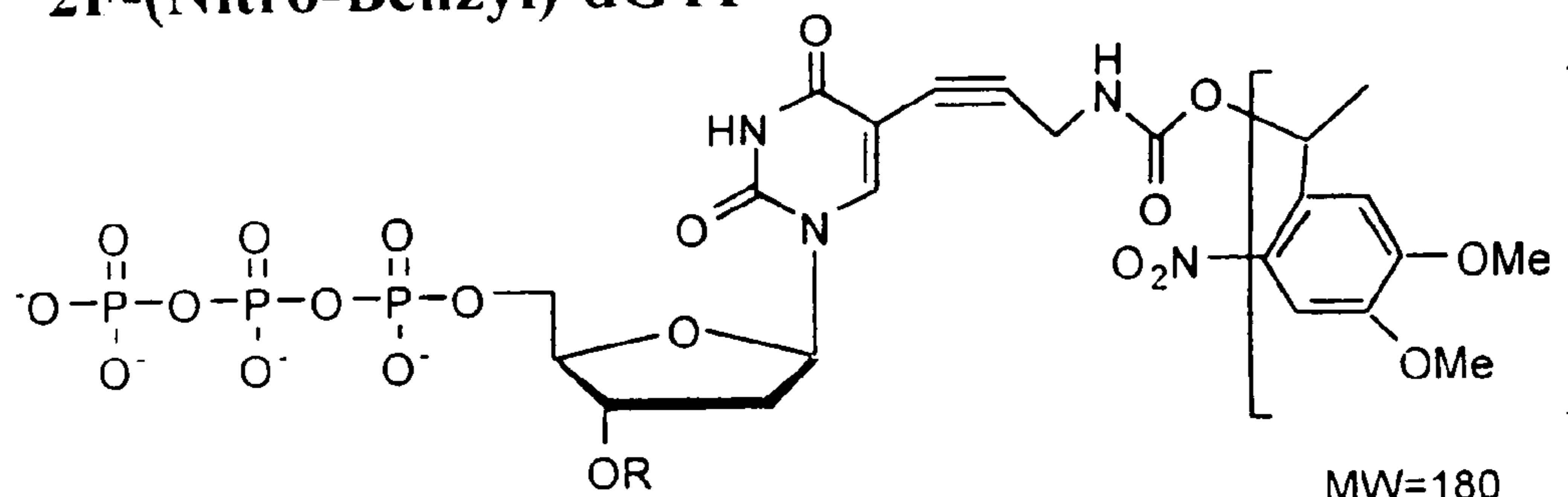
2(Meo)-(Nitro-Benzyl)-dTTP
