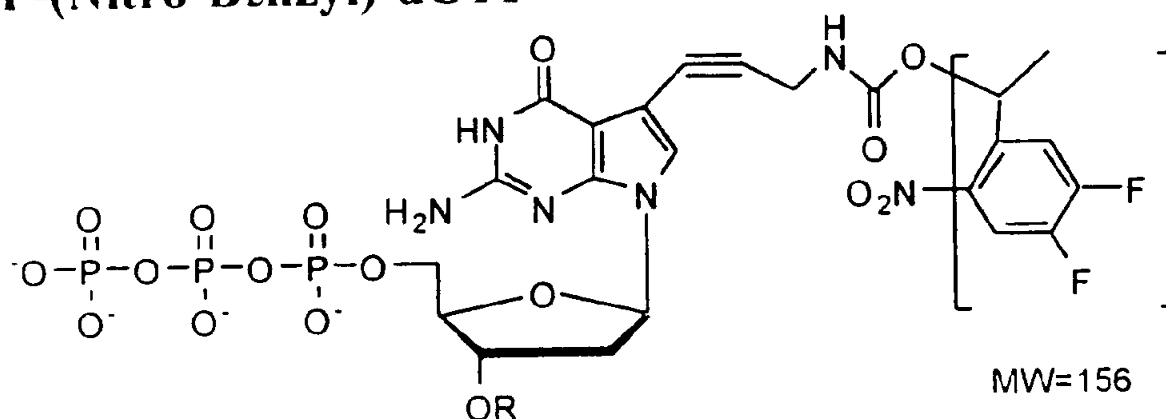
2F-(Nitro-Benzyl)-dGTP
