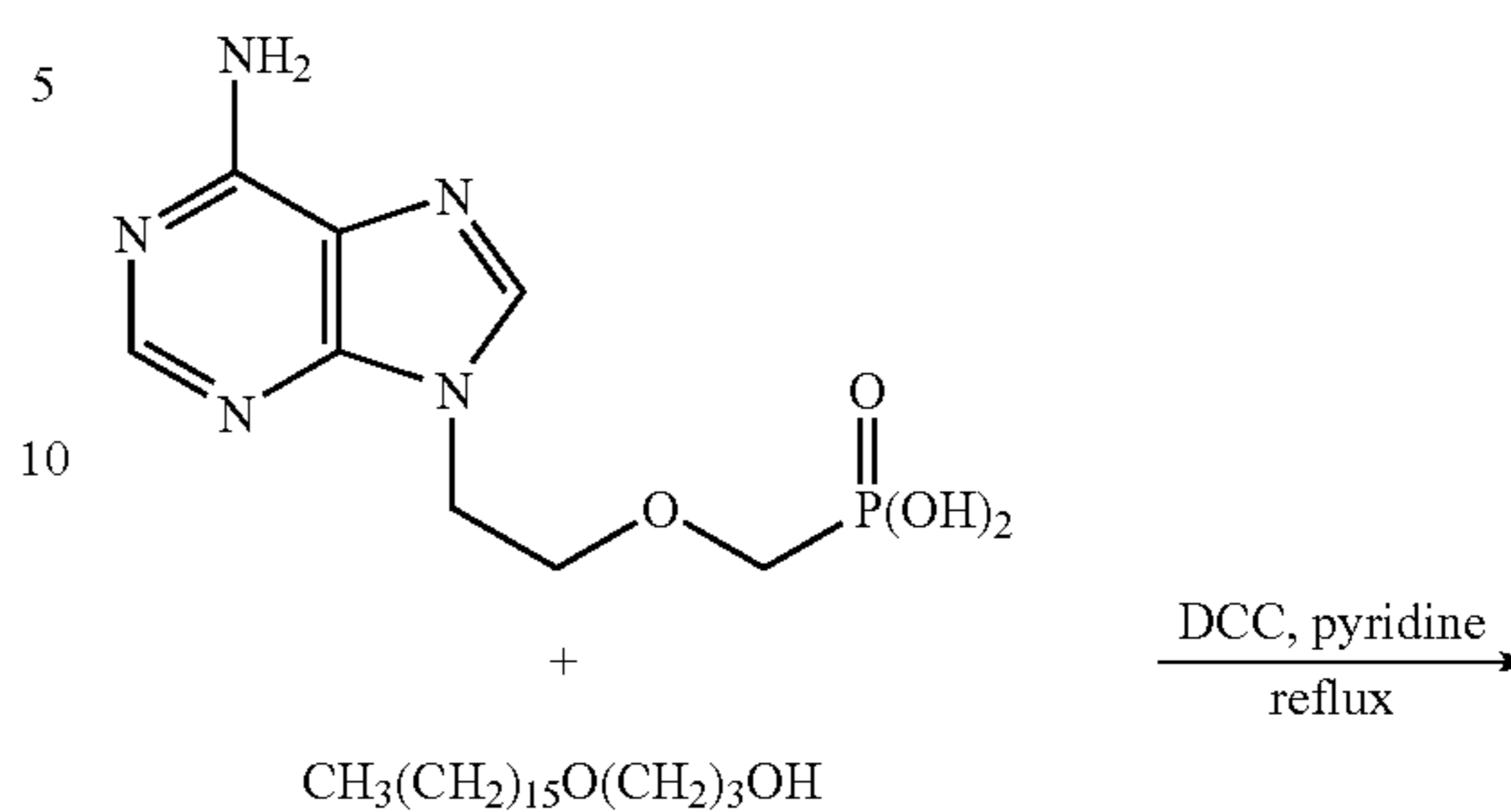
Scheme VI
