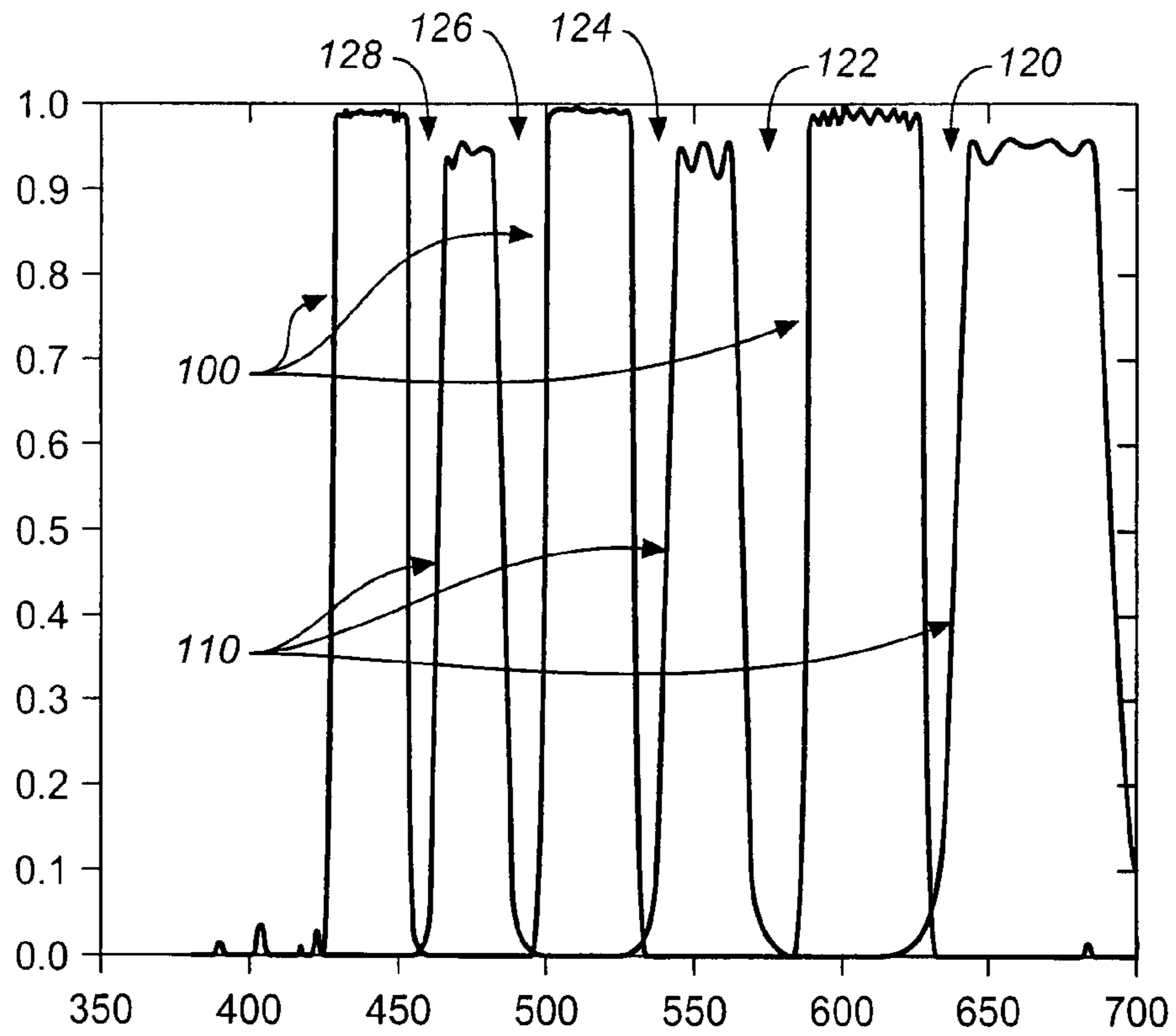
FIG. 1B
