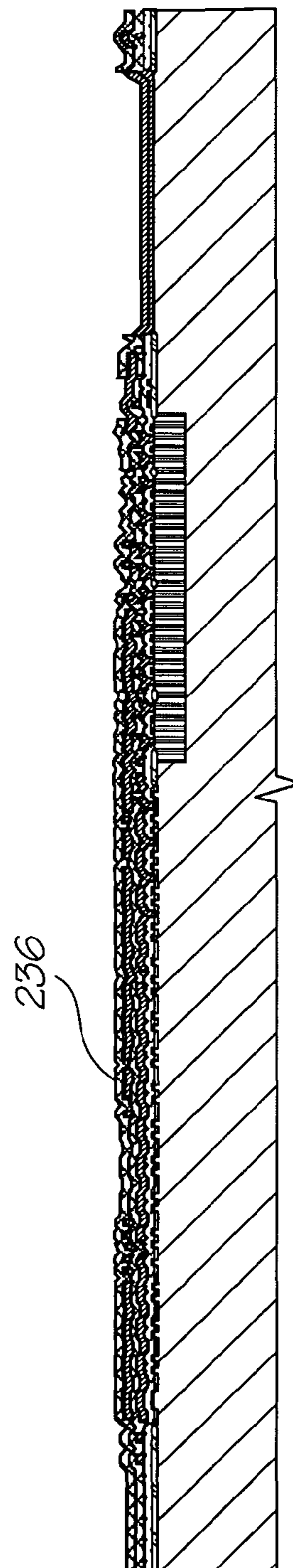
Deposit ILD 3, etch vias
