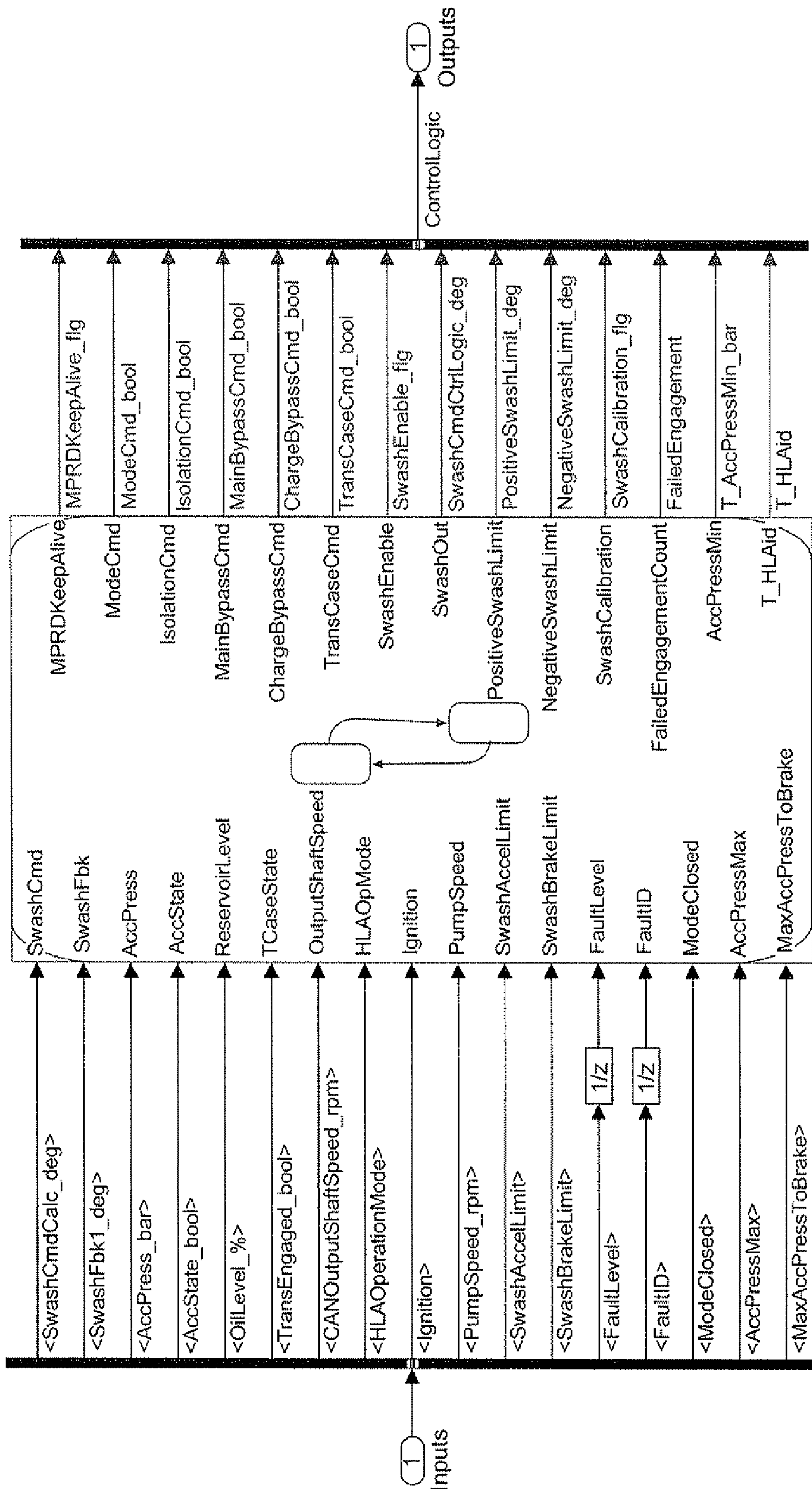
HLAControl :: HLAStateMachine
