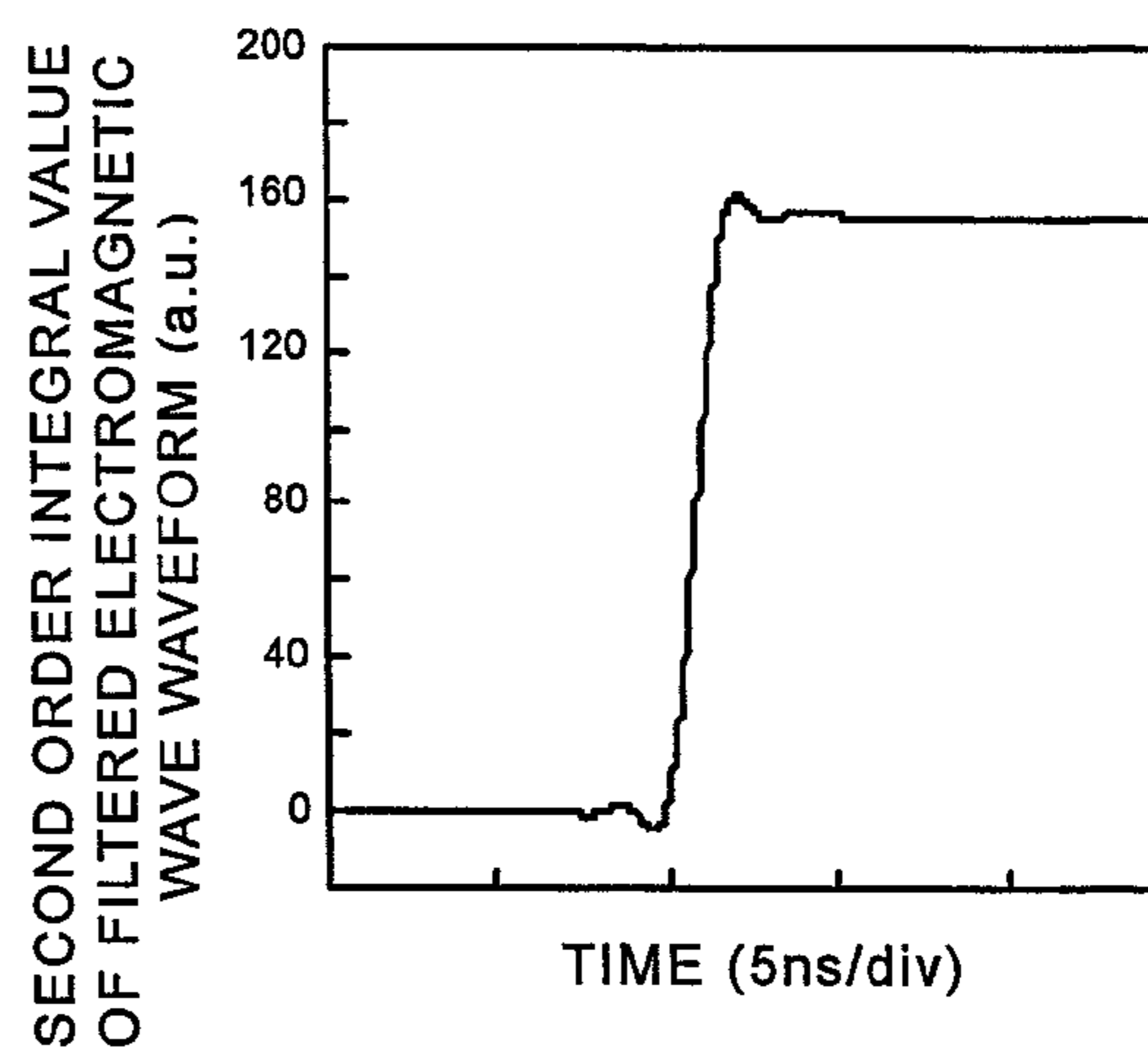
(d) SECOND ORDER INTEGRAL VALUE OF (b)
