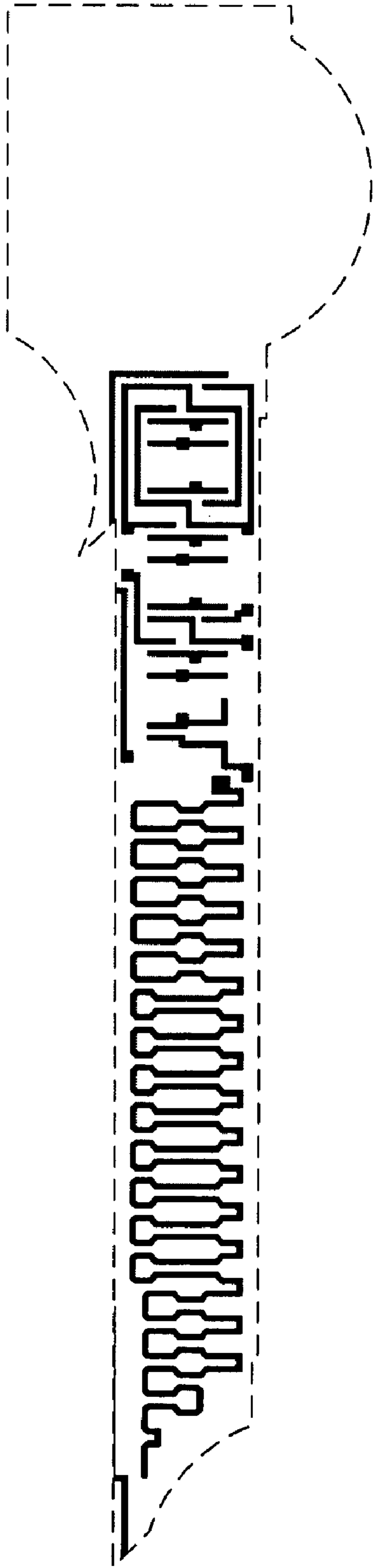
Poly mask
