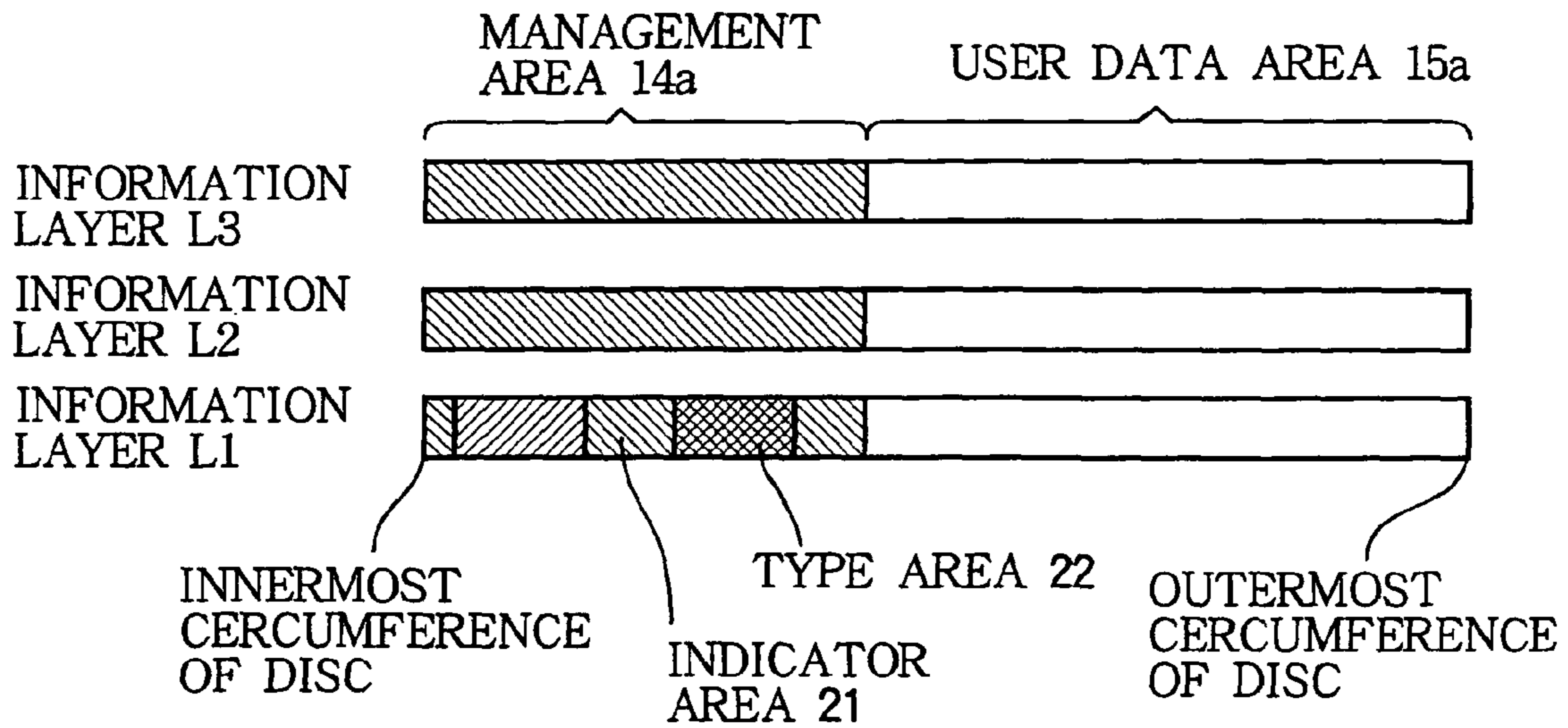
FIG. 11
